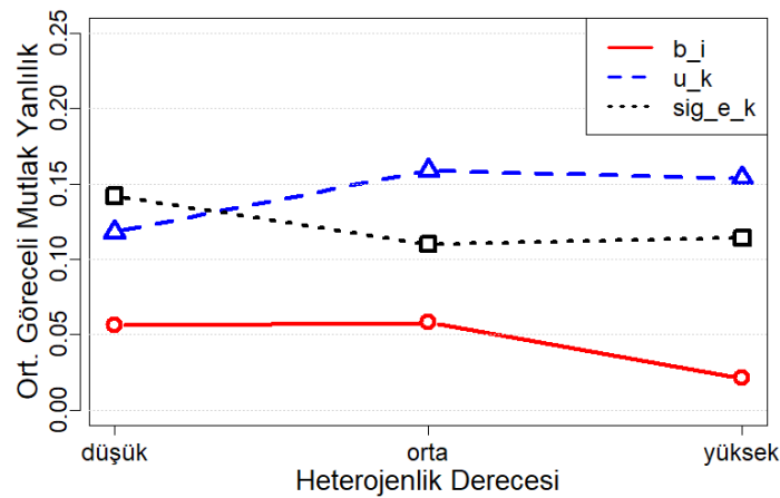
Şekil 14. Temel parametrelere ait ortalama göreceli mutlak yanlışlık değerlerinin değişimi.
