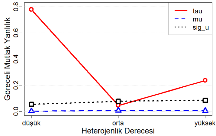
Şekil 9. Aşırı parametrelere ait göreceli mutlak yanlışlık değerlerinin değişimi.
