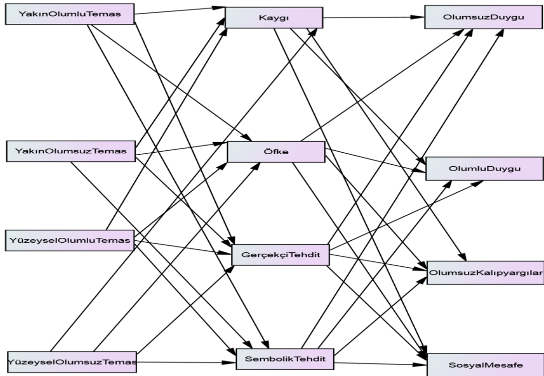
Şekil 1.1 : Test edilmesi amaçlanan model
