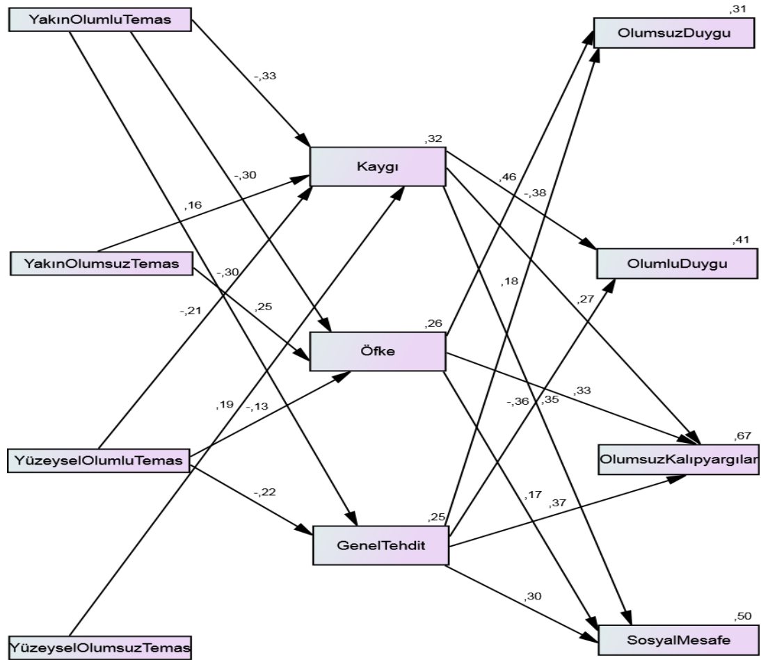
Şekil 3.2 : Standardize katsayıların gösterimiyle yol analizinin sonuçları.
