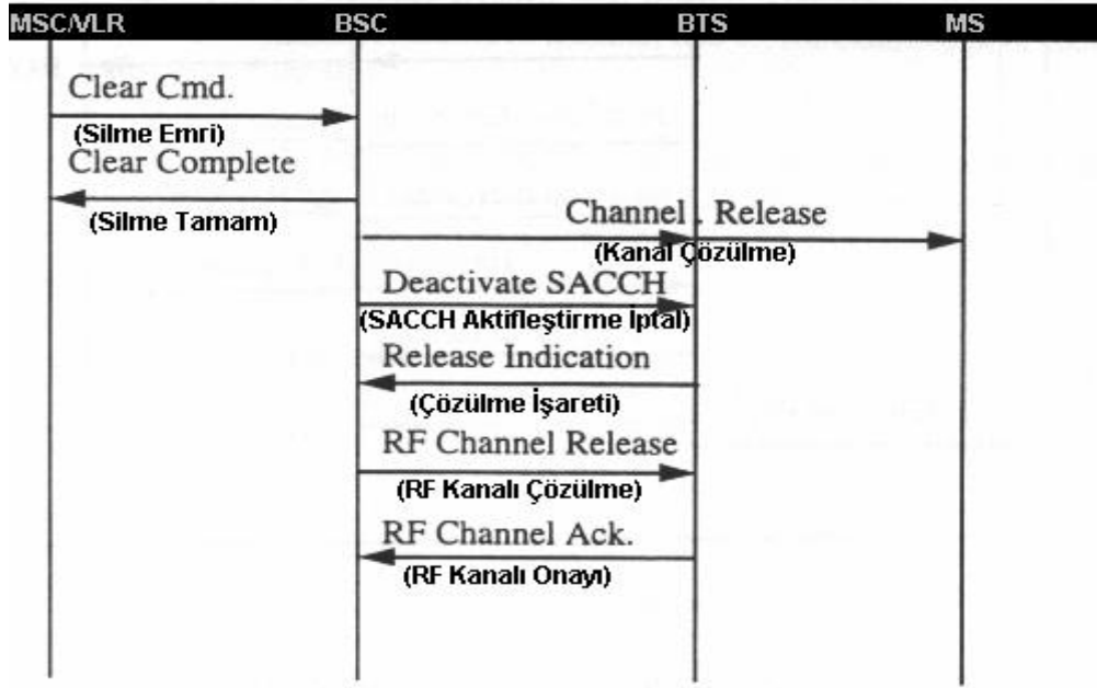
Şekil 3.11 - Silme için BSS işaretlenmesi
