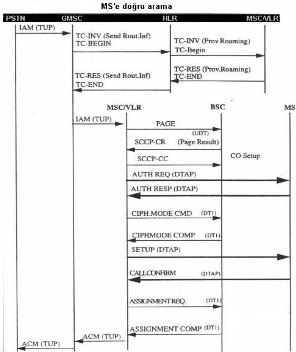
Şekil 3.4 - MS'e gelen bir aramanın işaretleşme sırası (1. Kısım)
