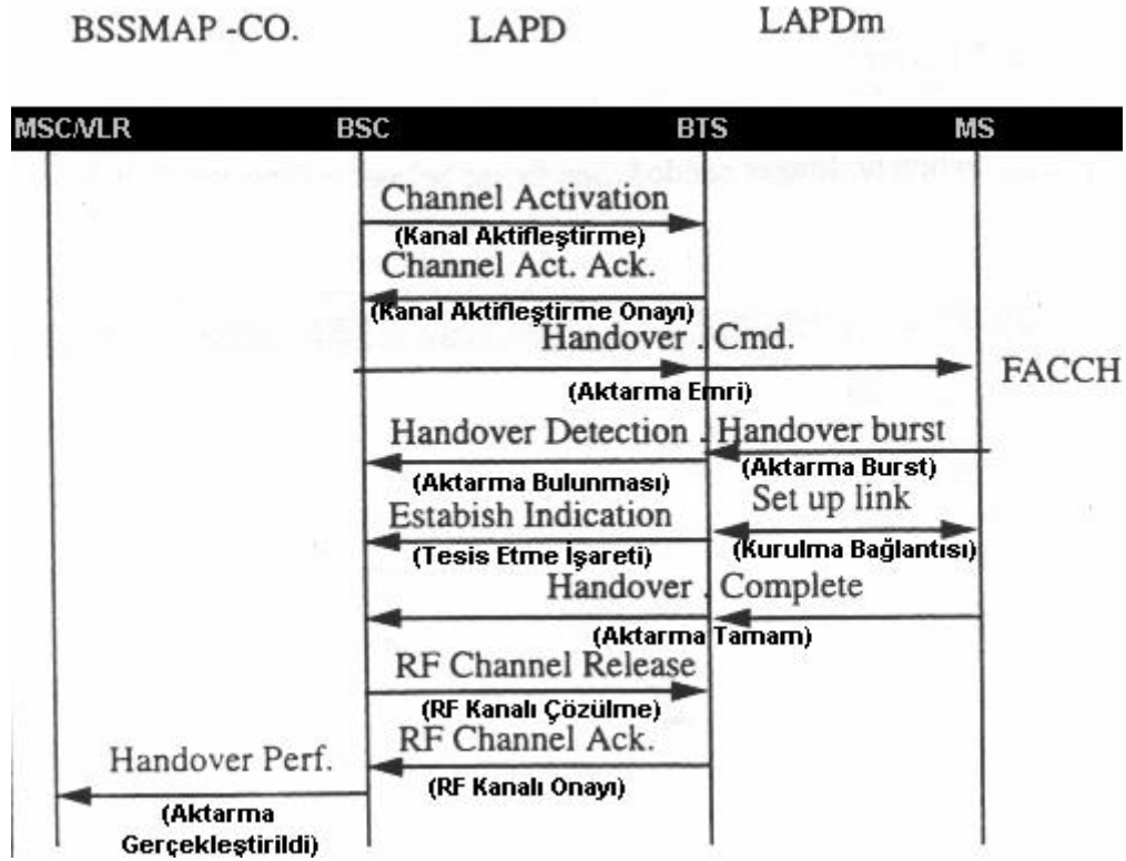
Şekil 3.10 - BSS içi aktarma
