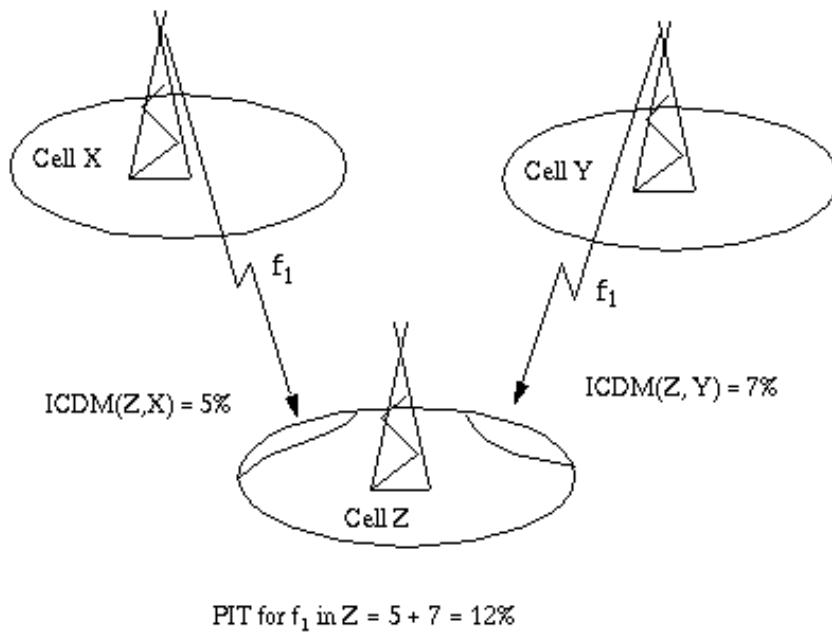
Şekil 4.4 - PIT Hesaplaması
