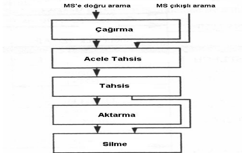
Şekil 3.6 - BSS temel dahili arama yönetimi
