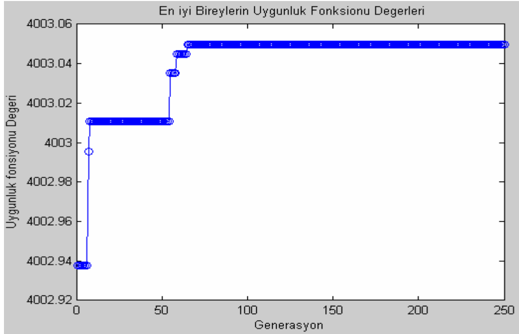
Şekil 5.10. IEEE 9 baralı sistemdeki beş numaralı yük barasının kritik aktif güç değerinin GA yöntemi ile elde edilmesi
