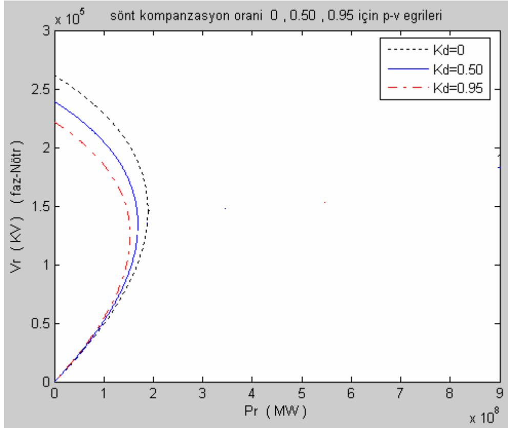
Şekil 4.10. Değişik şönt kompanzasyon oranları için P-V eğrileri
