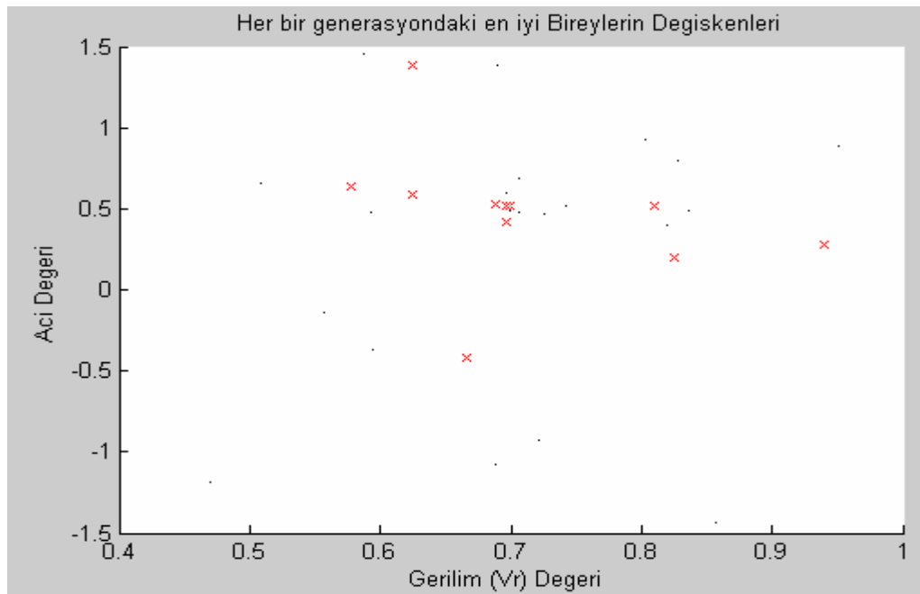
Şekil 5.11. IEEE 9 baralı sistemdeki beş numaralı yük barasının kritik gerilim ve açı değerinin GA yöntemi ile elde edilmesi
