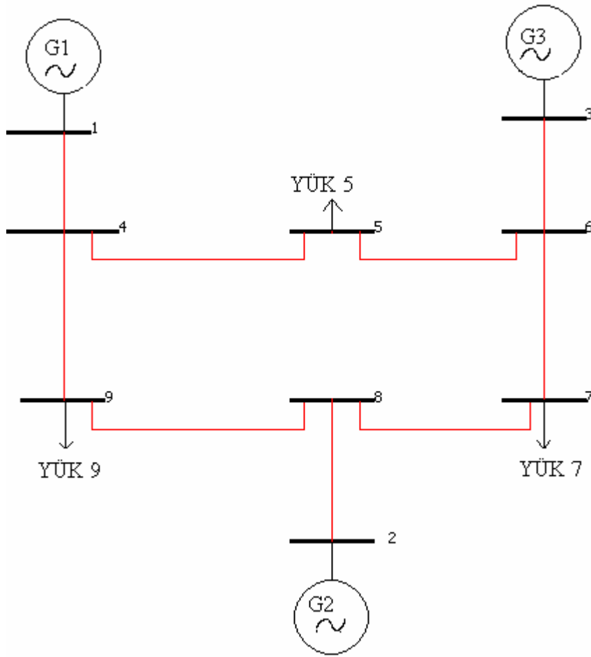
Şekil 5.9. IEEE'nin örnek dokuz baralı güç sistemi
