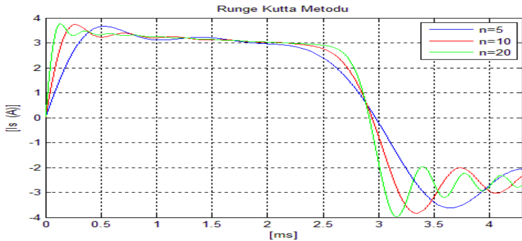
Şekil 4.4. Uygulama 4.1 için Runge Kutta yöntemi ile elde edilen kaynak akımı
