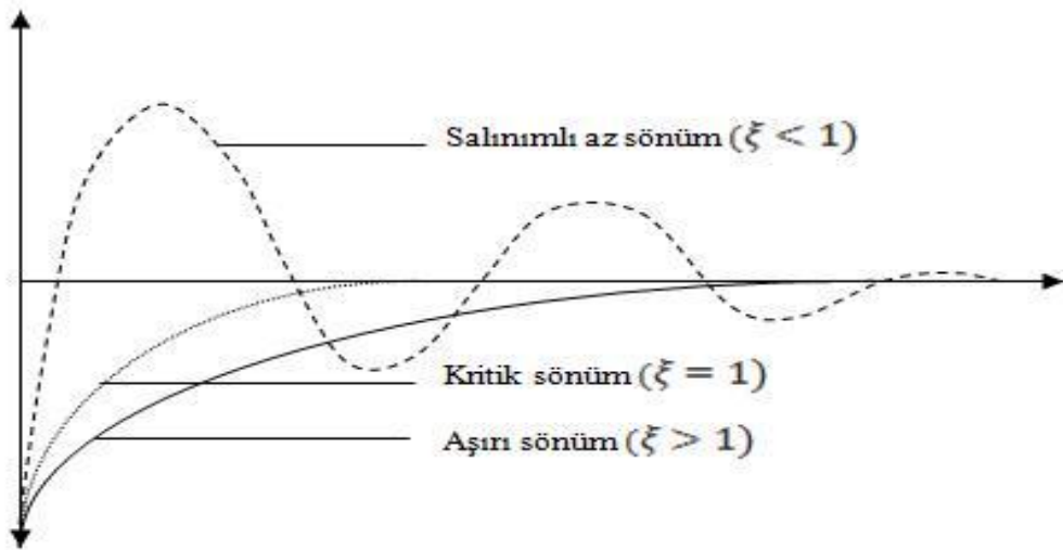
Şekil 3.14. Dalga sönüm şekilleri
