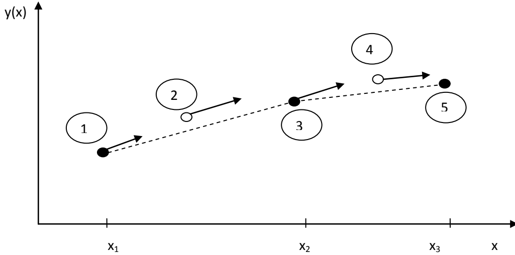
Şekil 3.11. Runge Kutta yöntemi grafiği
