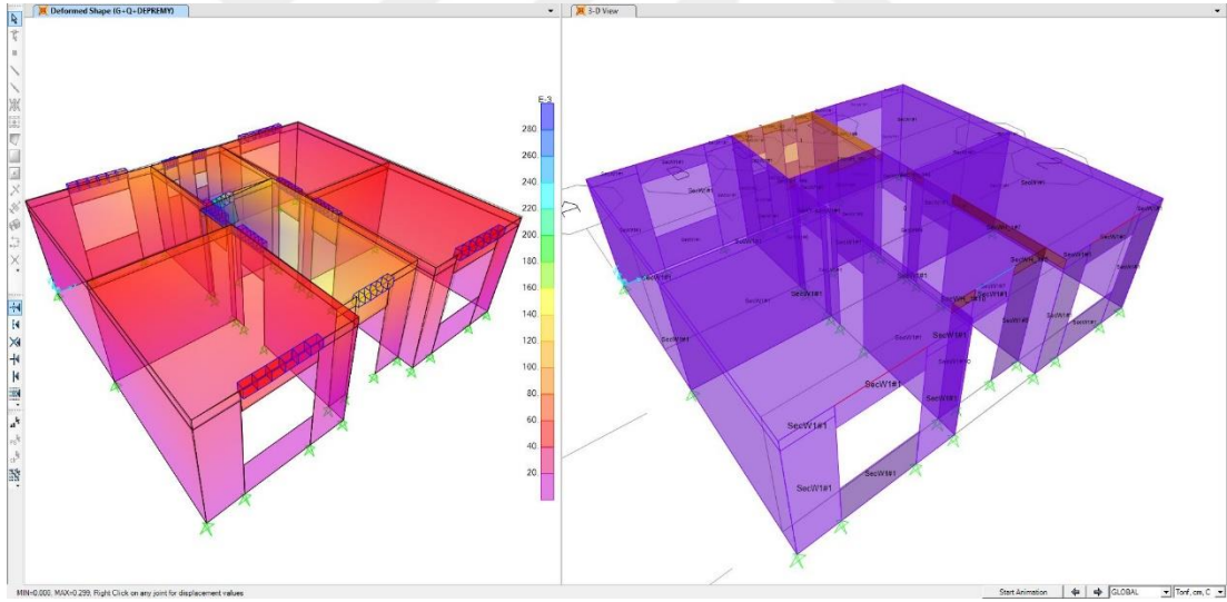
Şekil 6.12. Mevcut yapıya üç boyutlu deplasmanları (G+Q+DEPREM)
