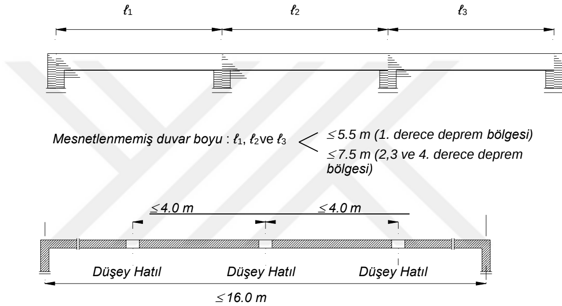
Şekil 6.5. Planda duvar boyları için sınırlar
