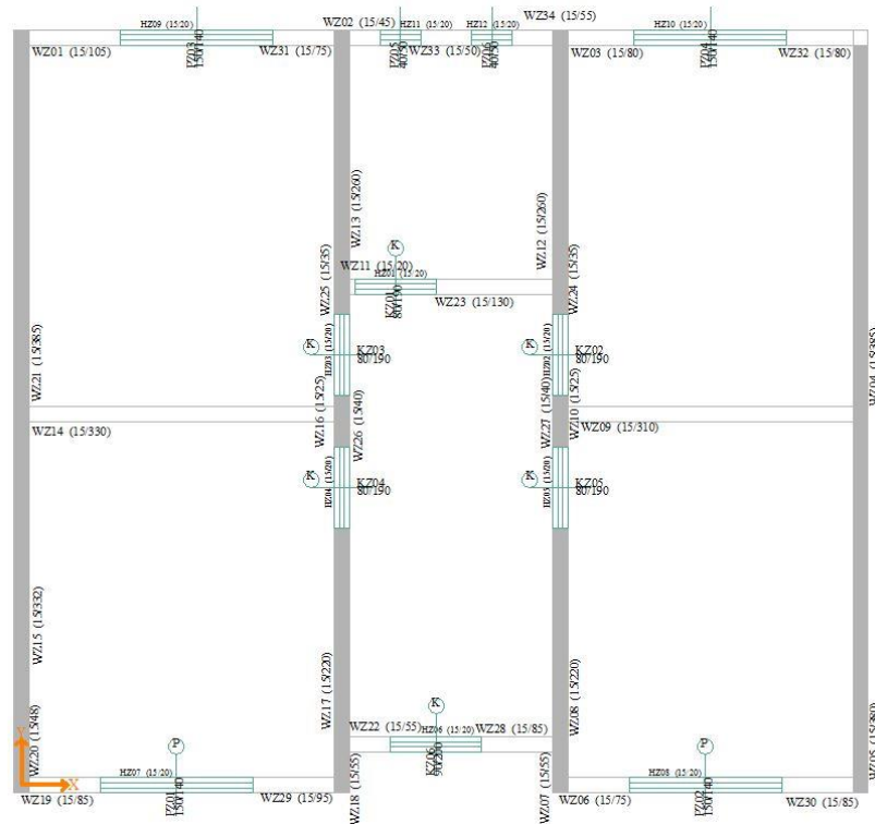
Şekil 6.9. Mevcut yığma yapının duvar yönleri
