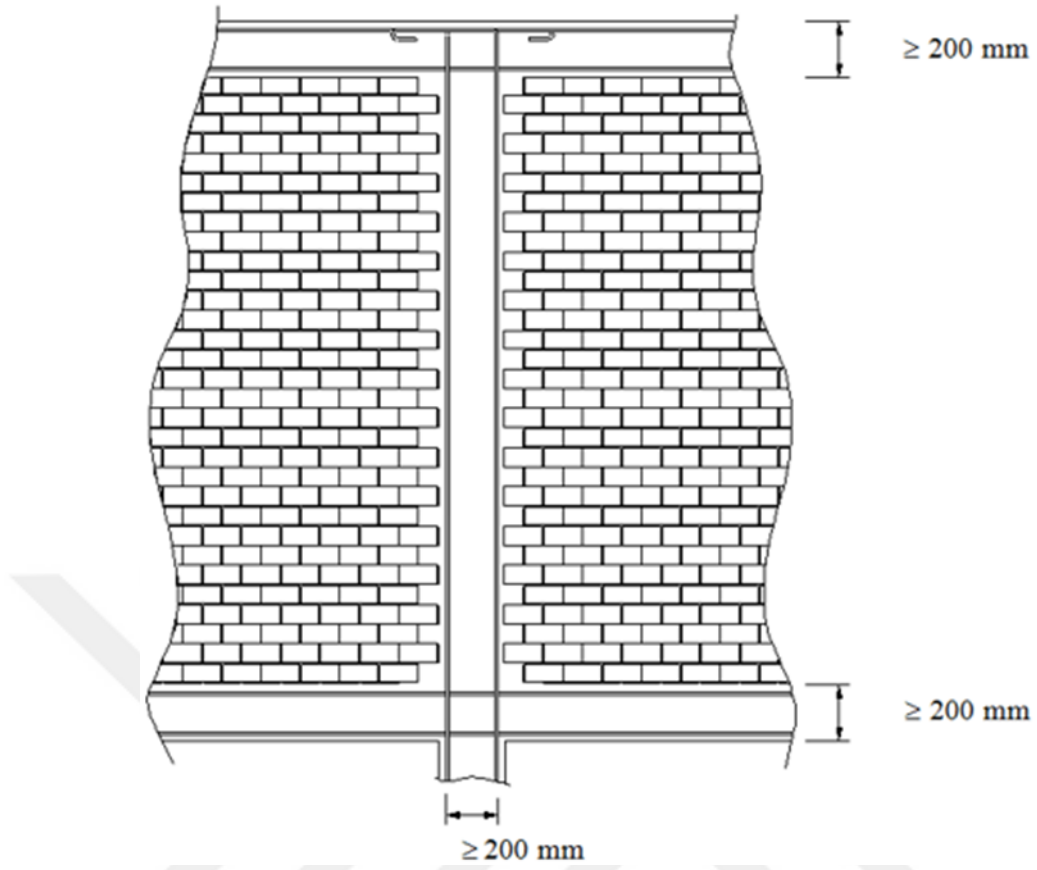
Şekil 6.7. Planda duvar boşlukları için sınırlar
