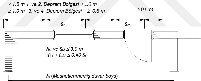
Şekil 6.6. Planda duvar boşlukları için sınırlar
