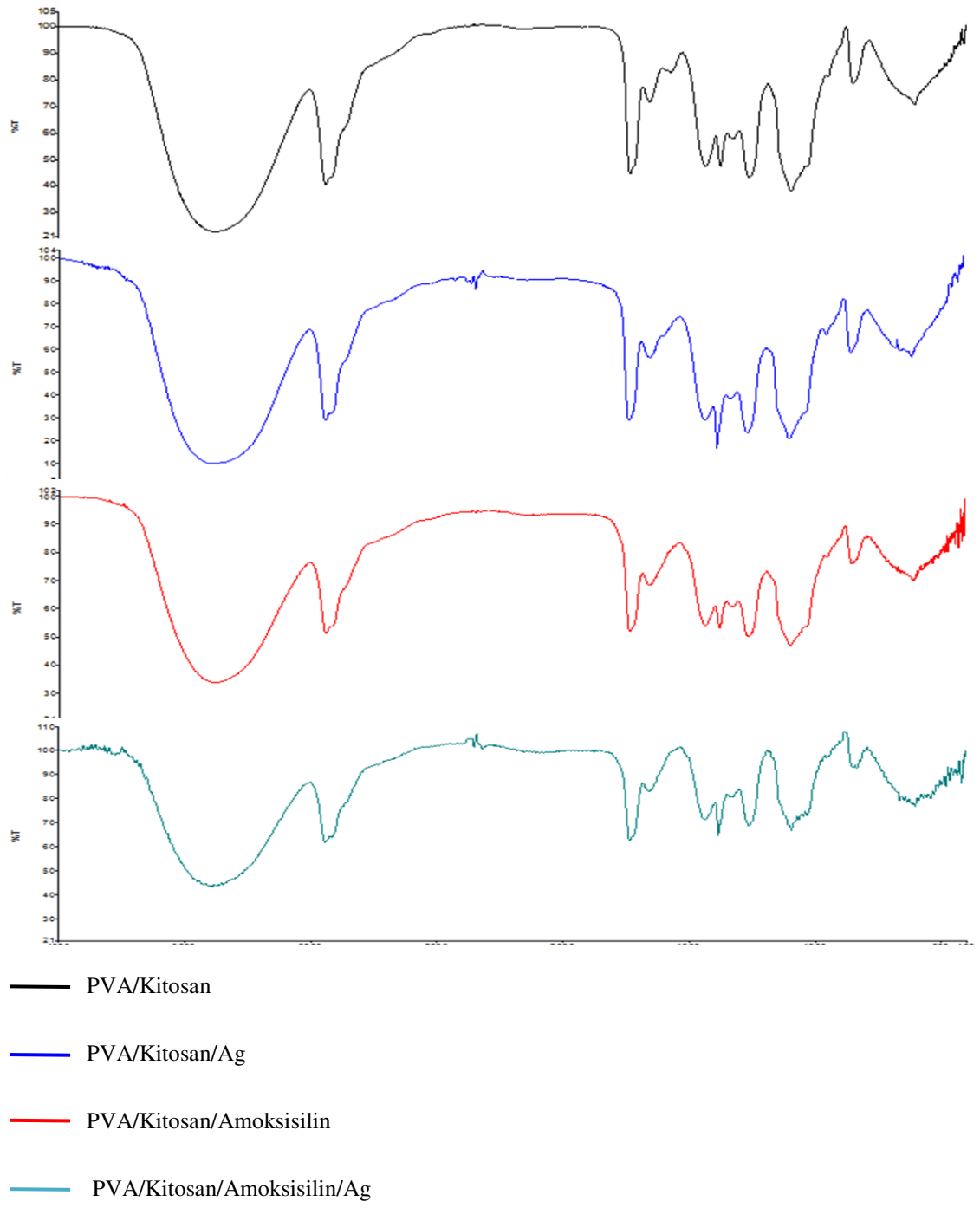
Şekil 4.1. Nanoliğlerin IR spektrumları
