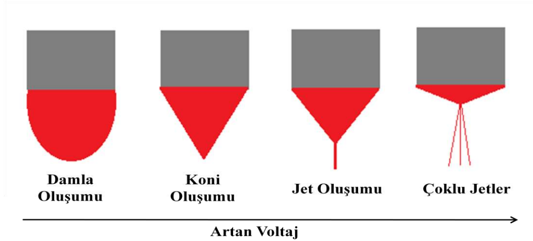
Şekil 2.8. Taylor konisi oluşumu
