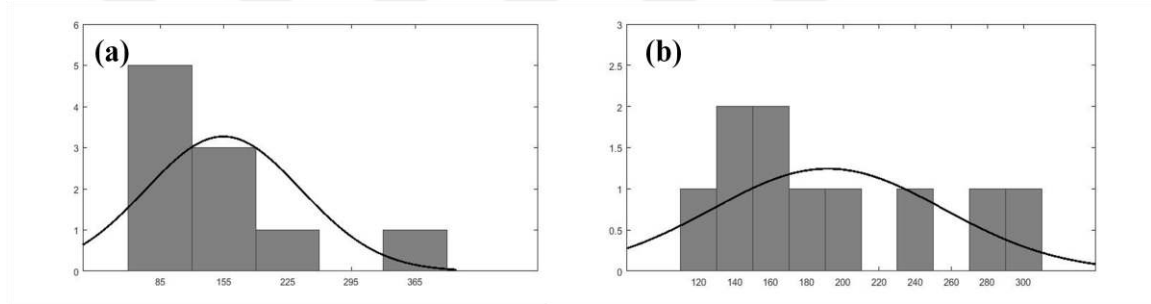
Şekil 4.20. PVA/Kitosan/Amoksisilin/Ag nanoliflerinin (a) çapraz bağlanma öncesi; (b) çapraz bağlanma sonrası çap histogramları
