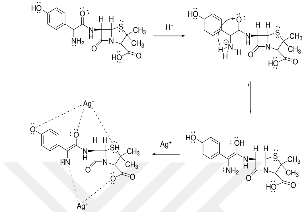
Şekil 4.12. Amoksisilin ile gümüş arasındaki reaksiyon mekanizması
