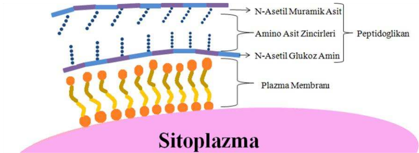
Şekil 2.3. \beta -Laktamlara karşı etki mekanizması
