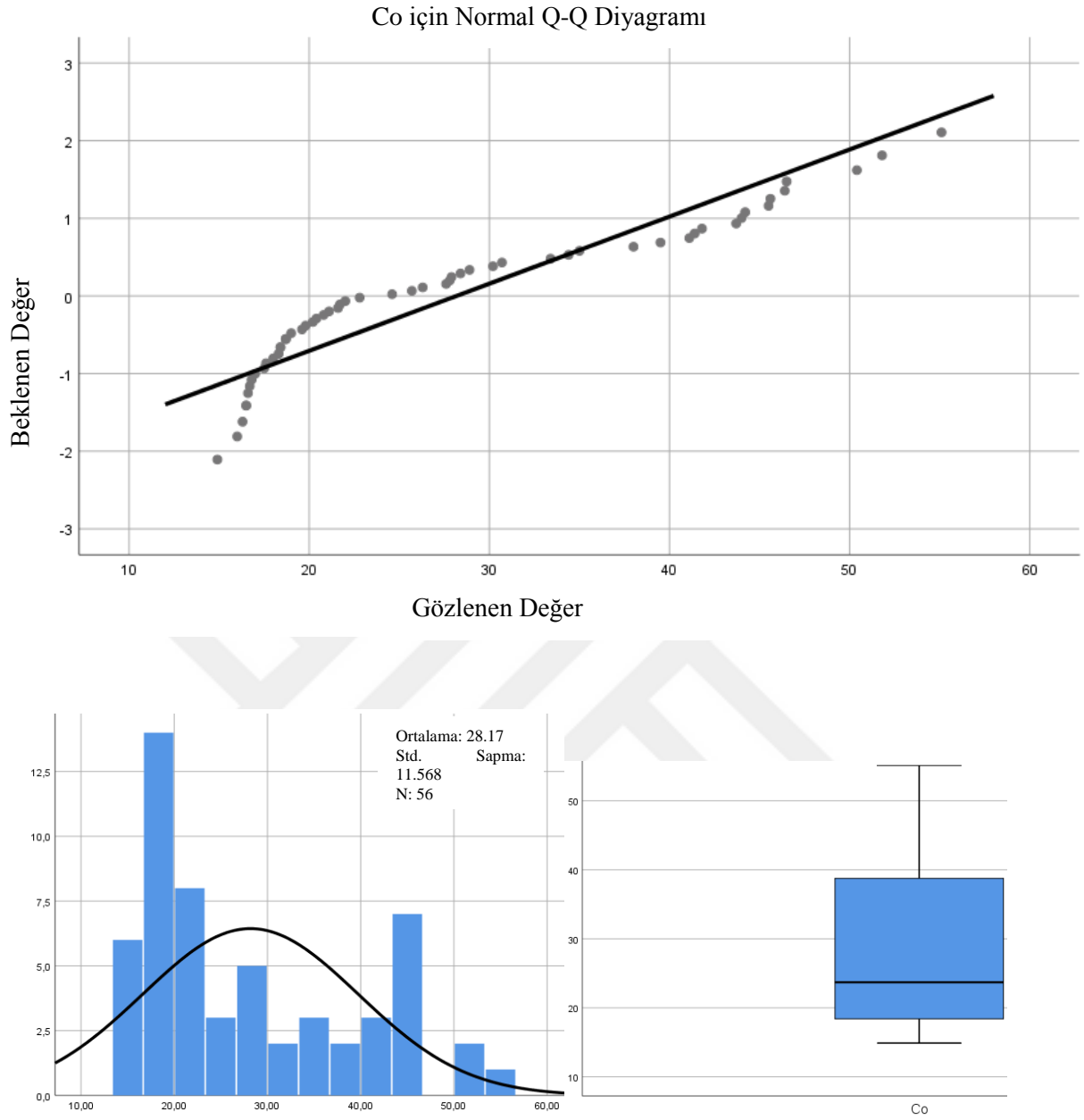
Şekil 3.28. Co elemetine ait dağılım oranları, histogram ve kutu diyagramı.
