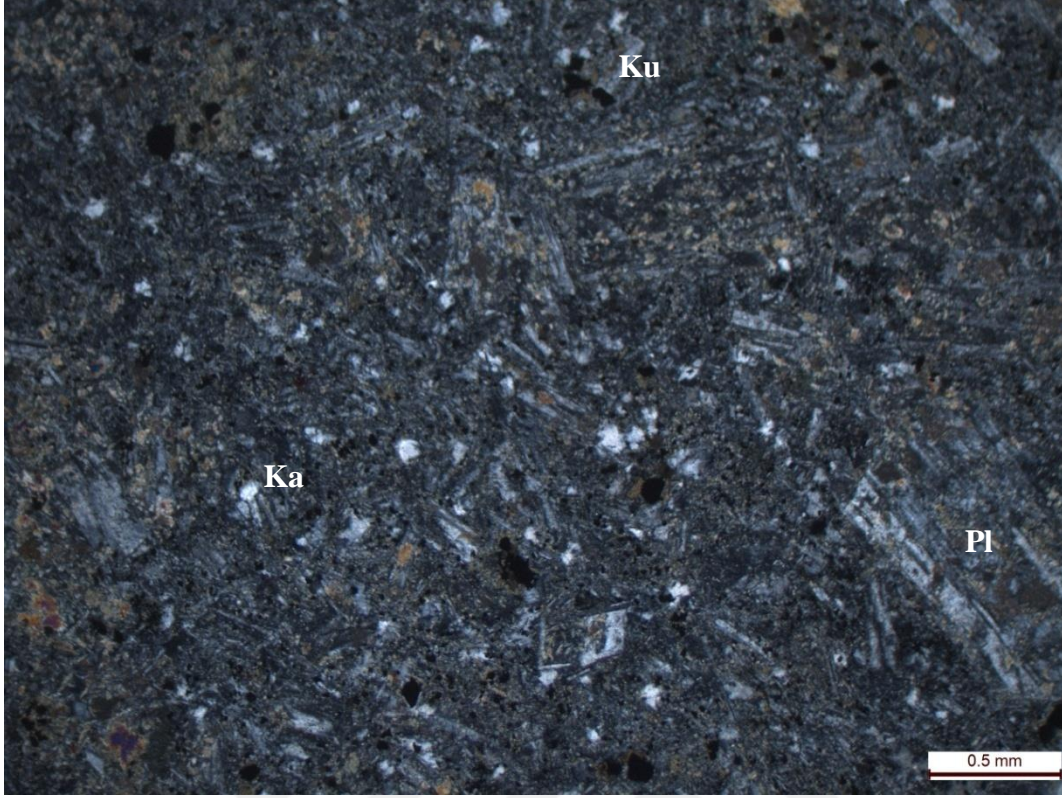
Şekil 3.8. Kermutdere Formasyonun'dan alınan kumtaşı örneğinin mikroskobik görünümü (Pl: Plajiyoklas, Ku: Kuvars, Ka: Kalsit, Ç.N)
