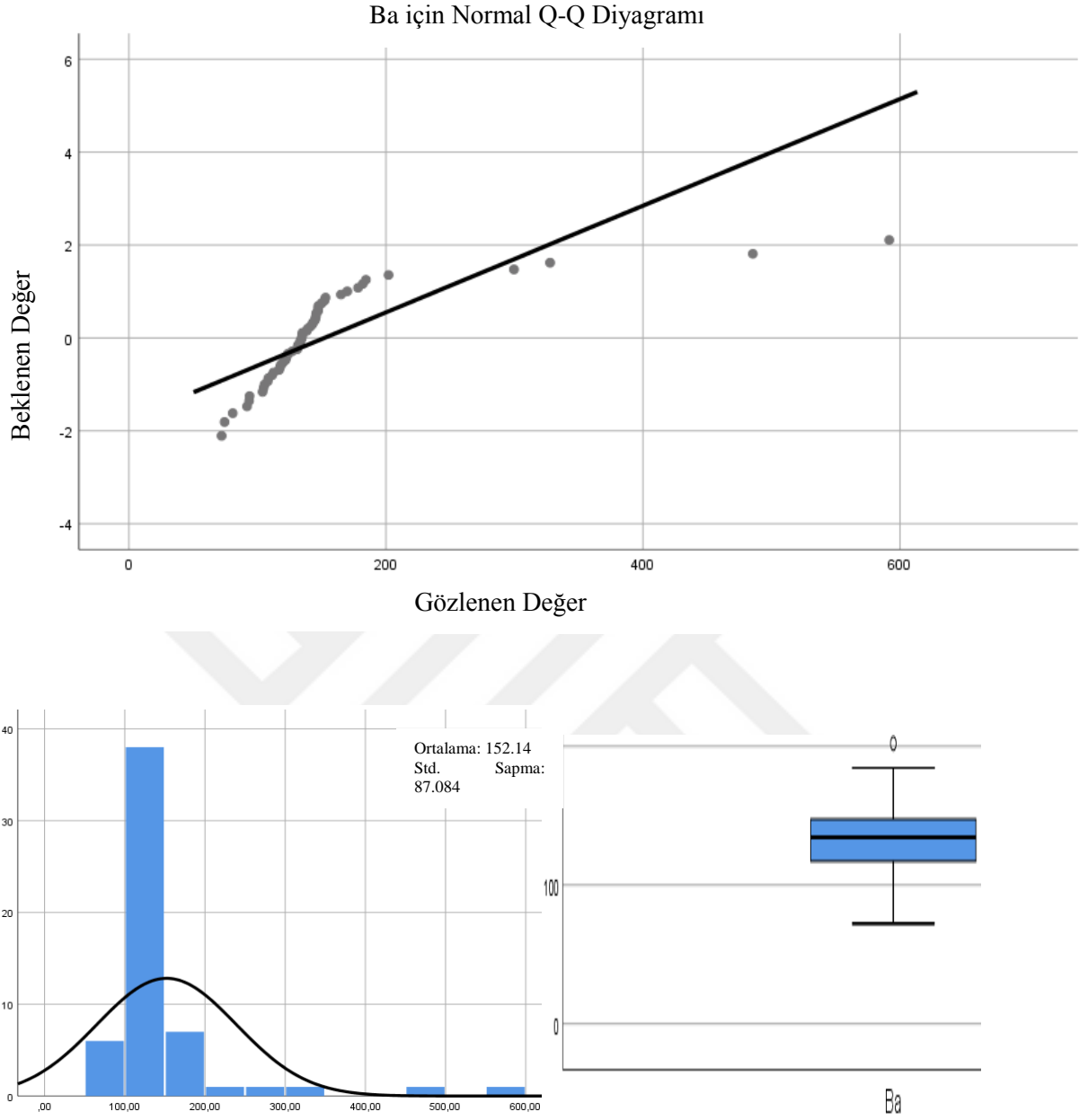
Şekil 3.40. Ba elemetine ait dağılım oranları, histogram ve kutu diyagramı.
