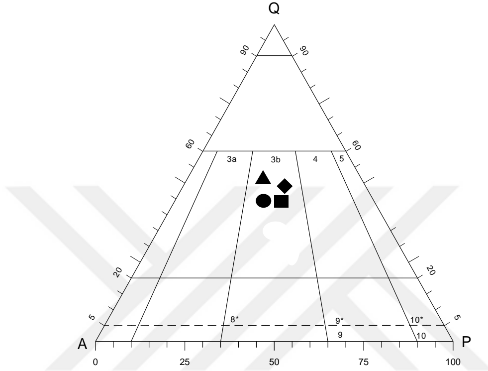
Şekil 3.2. Gümüşhane granitine ait kayaç örneklerinin QAP diyagramındaki konumları (Streckeisen, 1976).
