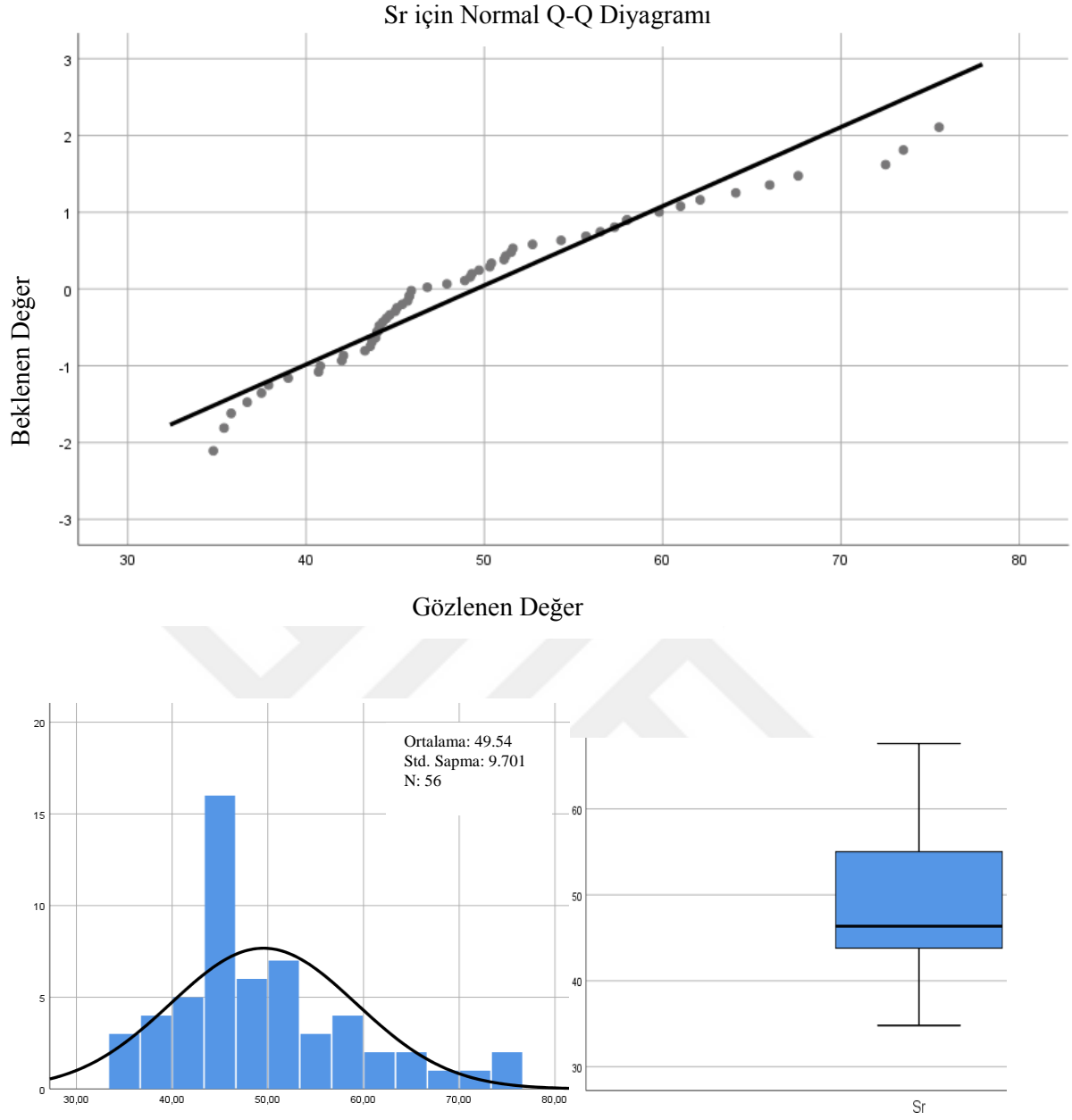
Şekil 3.33. Sr elemetine ait dağılım oranları, histogram ve kutu diyagramı.
