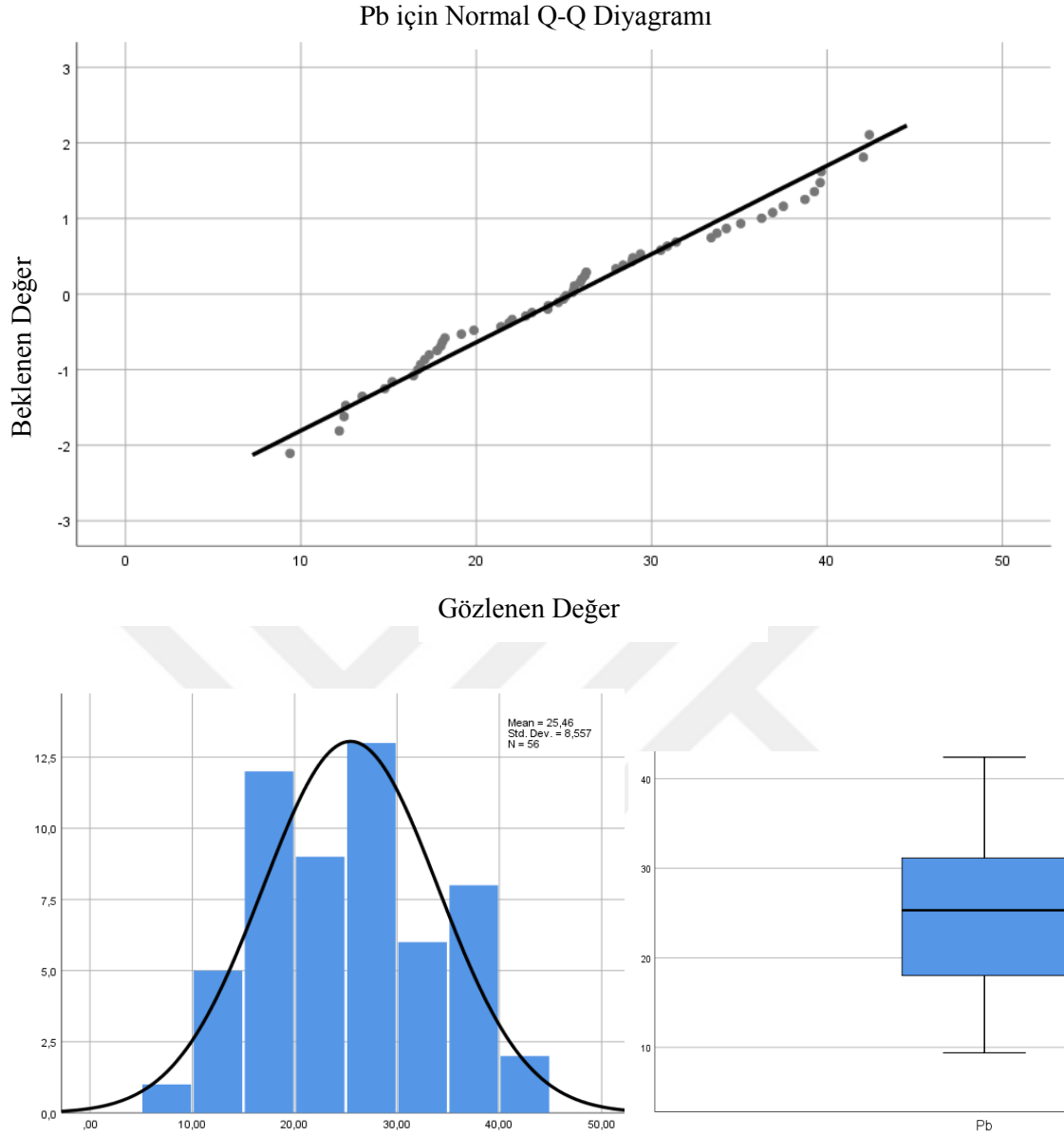
Şekil 3.24. Pb elemetine ait dağılım oranları, histogram ve kutu diyagramı.
