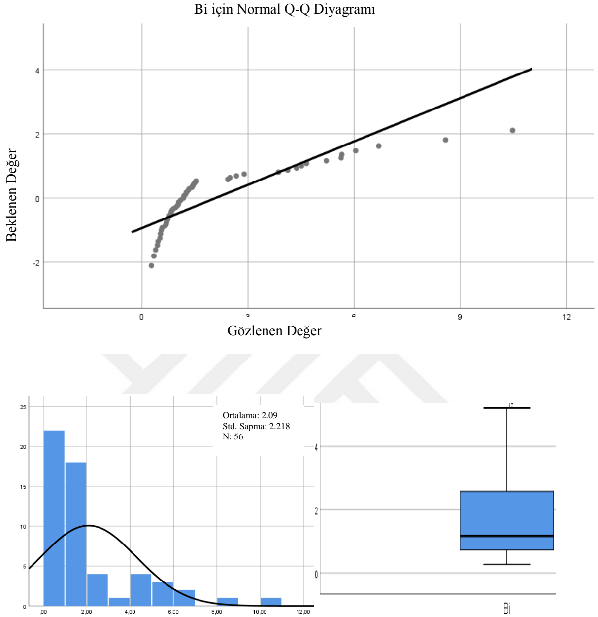
Şekil 3.36. Bi elemetine ait dağılım oranları, histogram ve kutu diyagramı.
