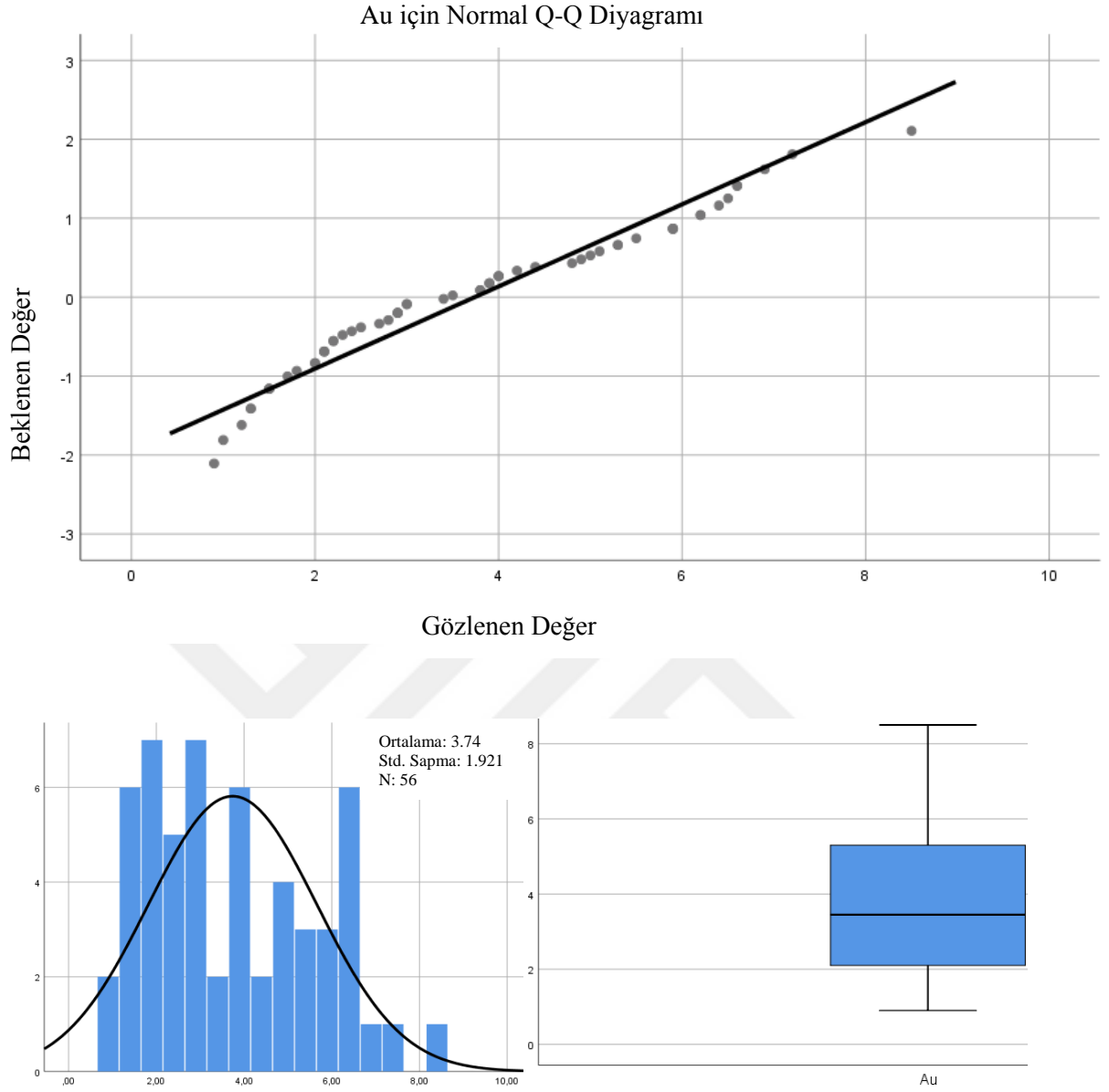
Şekil 3.32. Au elemetine ait dağılım oranları, histogram ve kutu diyagramı.
