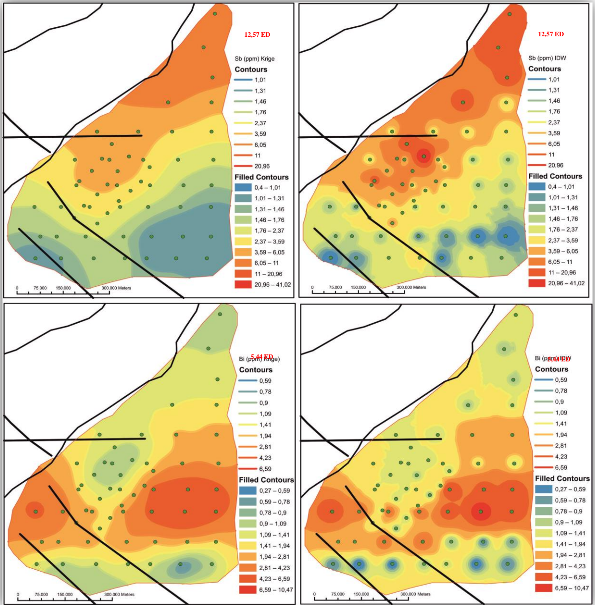
Şekil 3.51. Sb ve Bi elemetlerinin dağılım haritaları.
