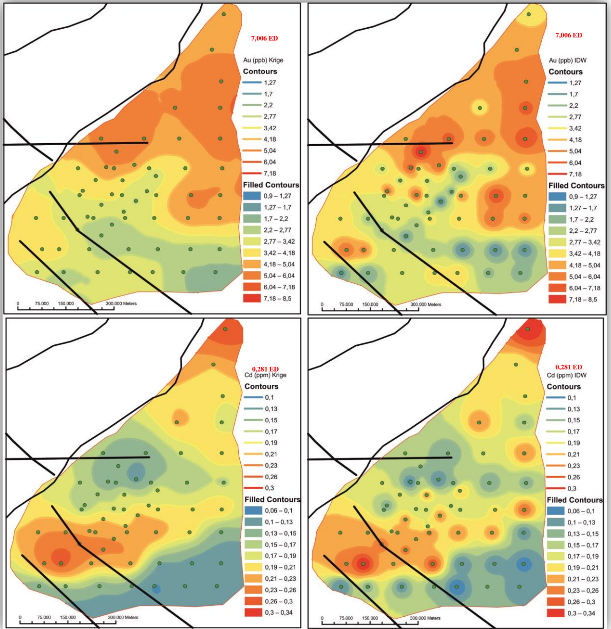
Şekil 3.50. Au ve Cd elementlerinin dağılım haritası.
