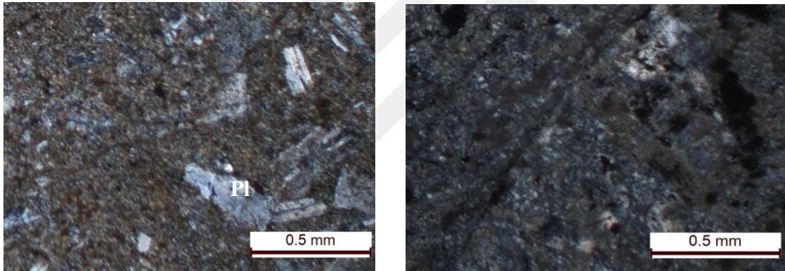
Şekil 3.4. Liyas volkanitlerini oluşturan kayalara ait mikroskopik görünüşleri. a) Mikrolitik doku, b) Mikrolitik porfirik doku (Ç.N., Pl: Plajiyoklas)
