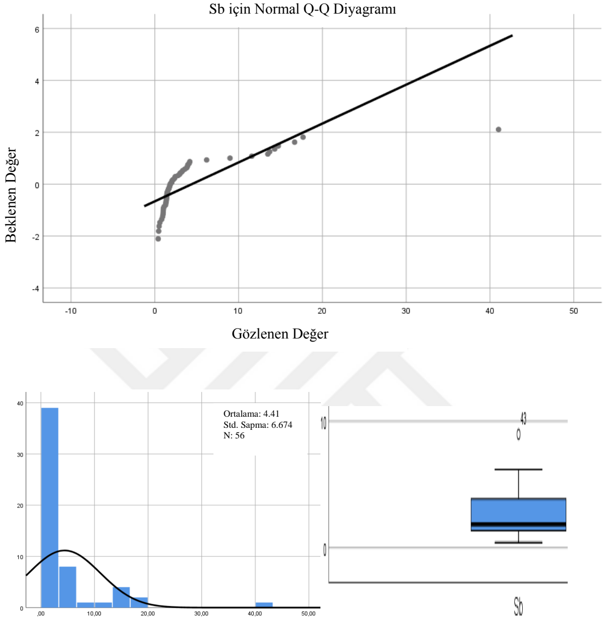
Şekil 3.35. Sb elemetine ait dağılım oranları, histogram ve kutu diyagramı.
