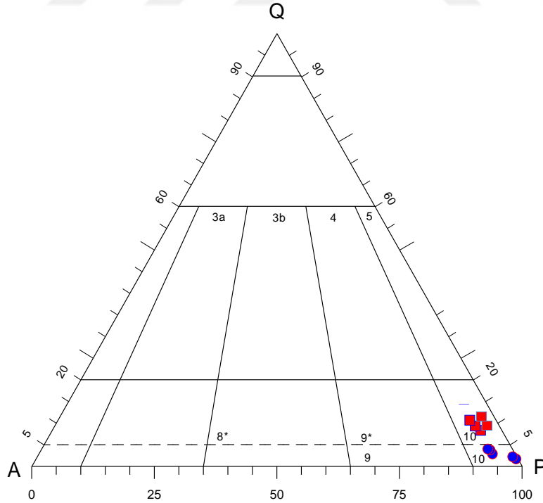
Şekil 3.14. Gümüştüğü Granitoyidi kayaç örneklerinin QAPF diyagramındaki konumları (Streckeisen, 1976).
