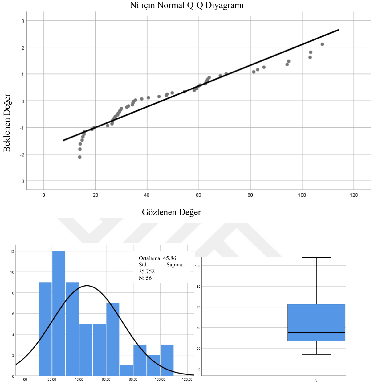
Şekil 3.27. Ni elemetine ait dağılım oranları, histogram ve kutu diyagramı.
