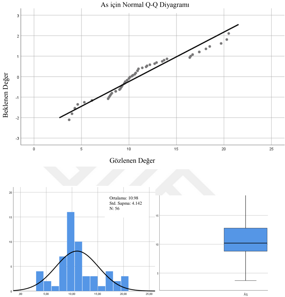
Şekil 3.31. As elemetine ait dağılım oranları, histogram ve kutu diyagramı.
