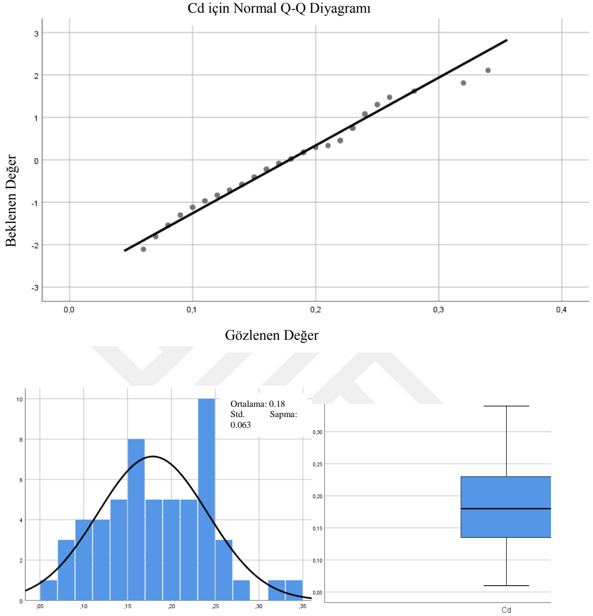
Şekil 3.34. Cd elemetine ait dağılım oranları, histogram ve kutu diyagramı.
