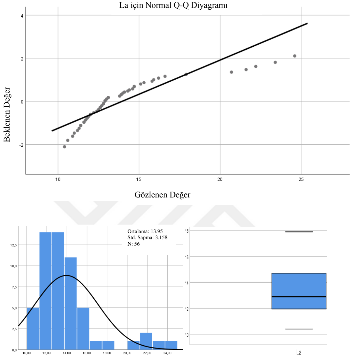
Şekil 3.38 La elemetine ait dağılım oranları, histogram ve kutu diyagramı.
