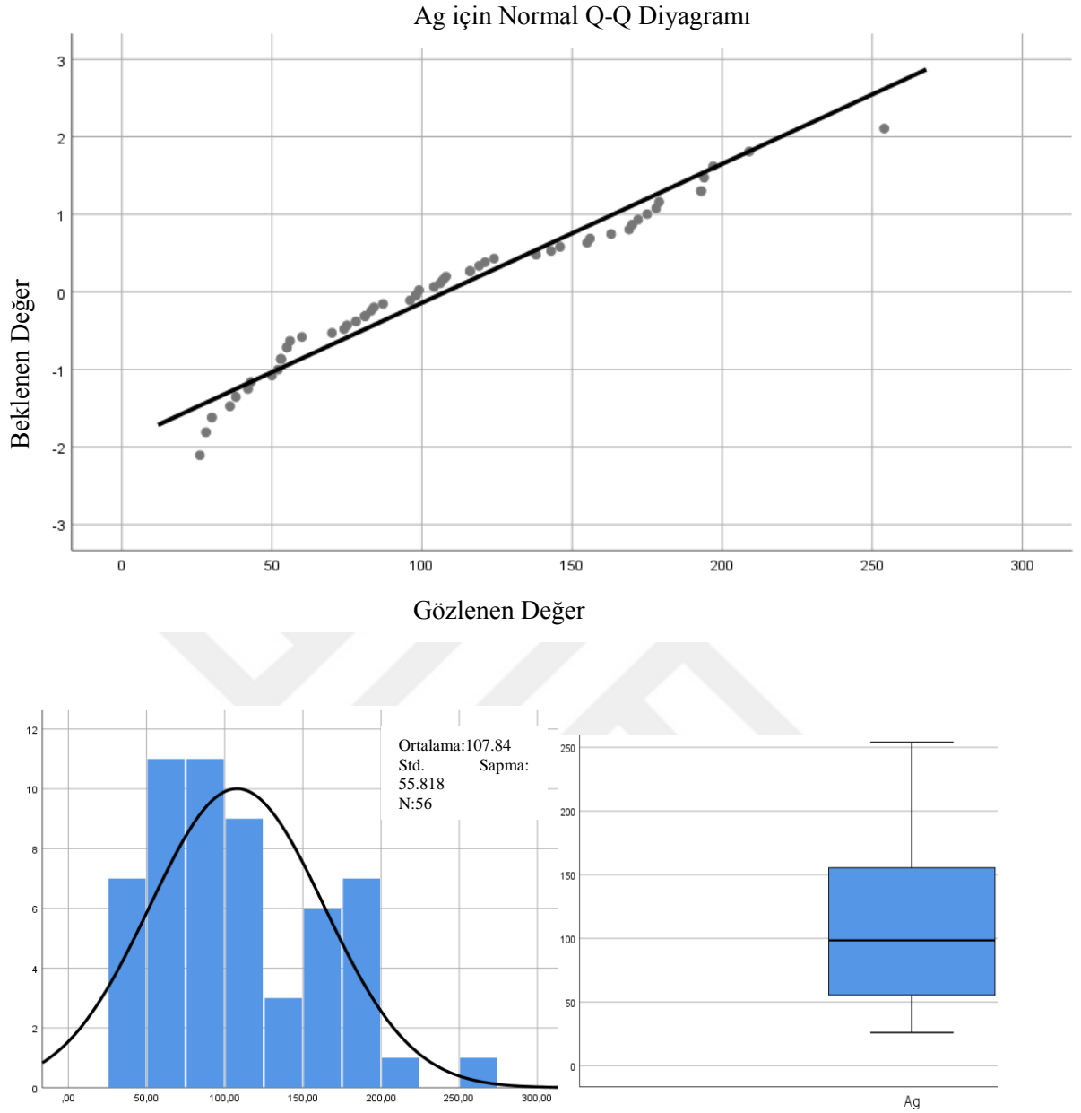
Şekil 3.26. Ag elemetine ait dağılım oranları, histogram ve kutu diyagramı.
