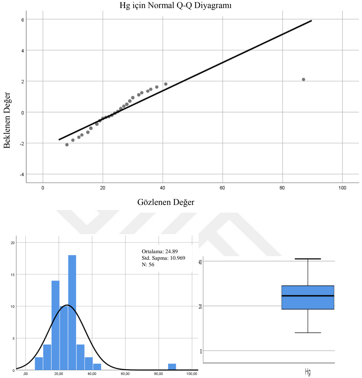
Şekil 3.42. Hg elemetine ait dağılım oranları, histogram ve kutu diyagramı.
