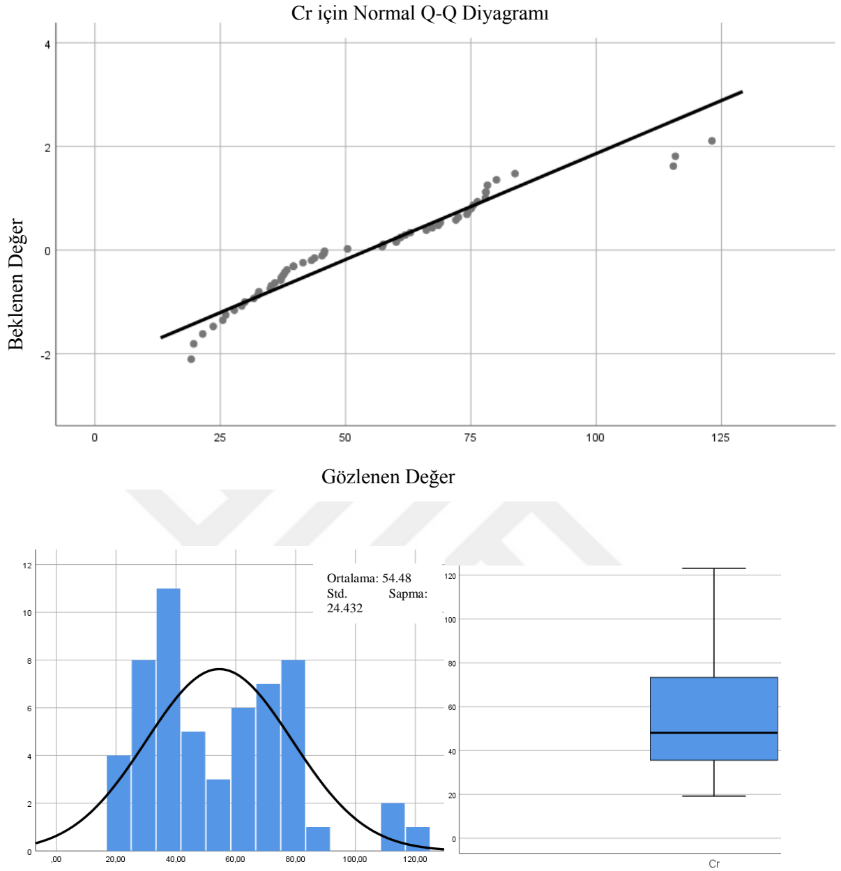
Şekil 3.39. Cr elemetine ait dağılım oranları, histogram ve kutu diyagramı.
