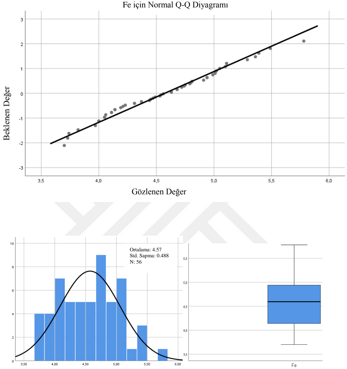
Şekil 3.30. Fe elemetine ait dağılım oranları, histogram ve kutu diyagramı.
