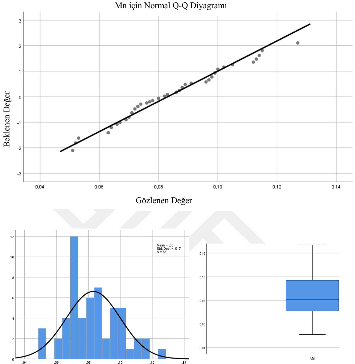
Şekil 3.29. Mn elemetine ait dağılım oranları, histogram ve kutu diyagramı.
