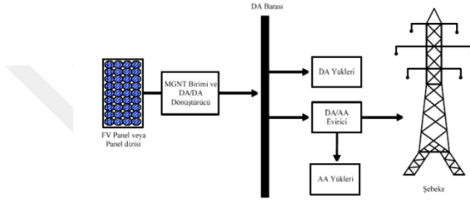
Şekil 3.8. Şebekeye bağlı FV sistemin şeması (Çakmak, 2012)
