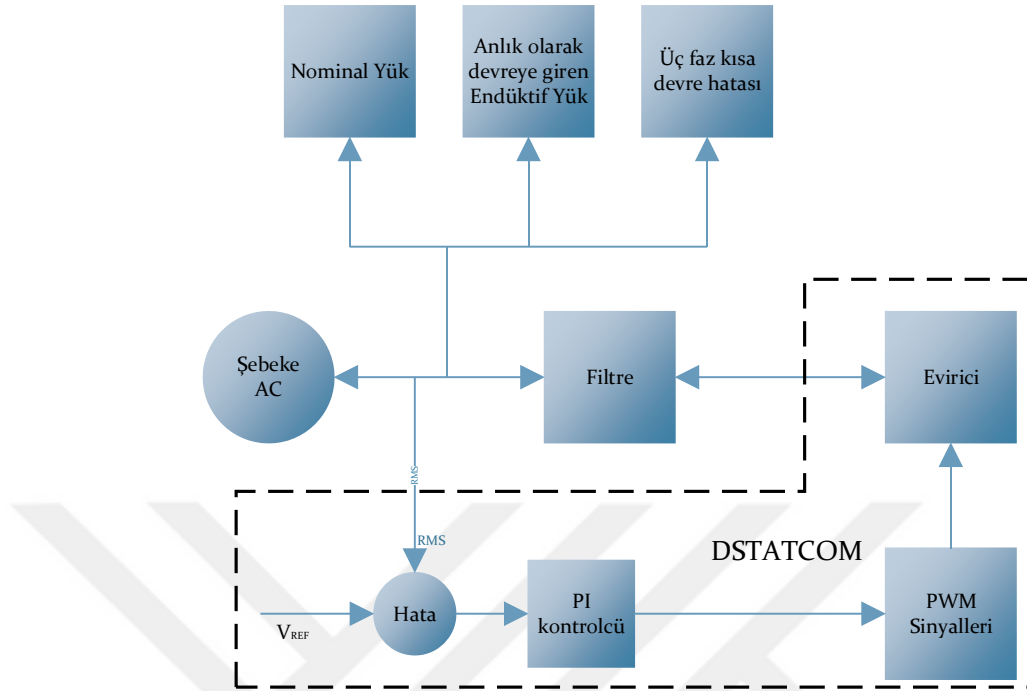
Şekil 5.2. DSTATCOM Sistemi ile Harmonik Filtrasyonu ve Güç Kalitesi İyileştirme Blok Diyagramı
