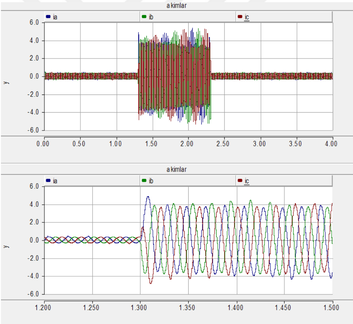
Şekil 5.10. dstatcom devrede iken üç fazlı yük akımının grafiği
