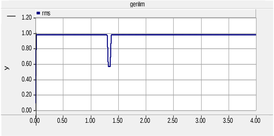
Şekil 5.12. Yük Trafında Üç Faz Kısa Devre Arızası RMS Grafiği
