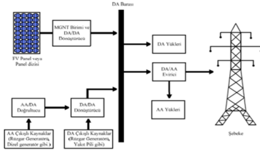
Şekil 3.9. Hibrit FV sistemin bağlantı şeması (Çakmak, 2012)
