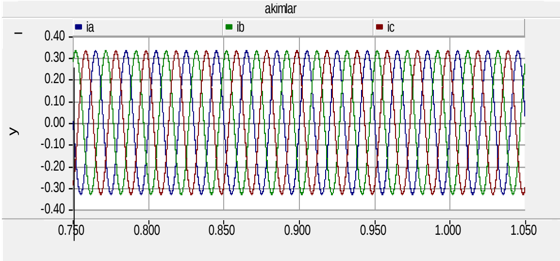
Şekil 5.3. Faz Akımları
