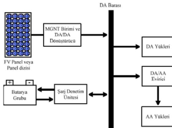
Şekil 3.7. Şebekeden bağımsız FV sistemin şeması (Çakmak, 2012)
