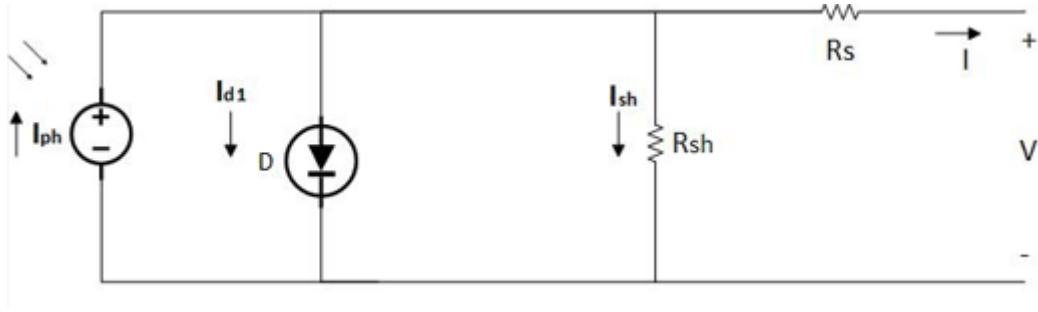
Şekil 3.4. Tek diyot modeli
