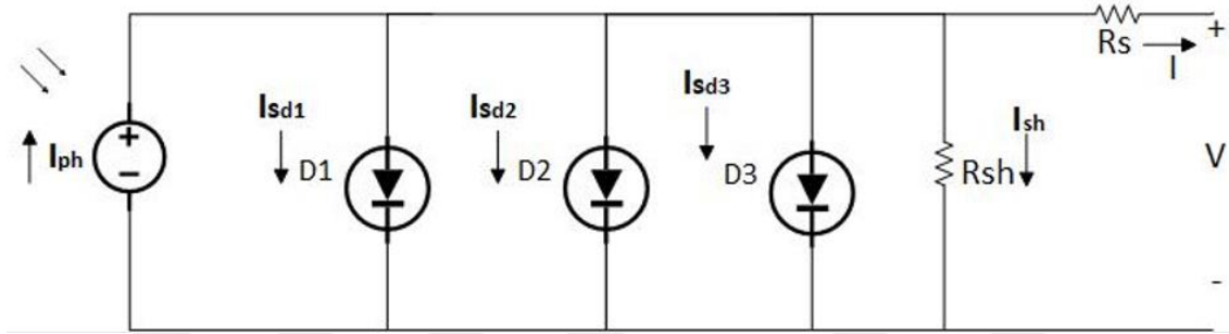
Şekil 3.6. Üç Diyot Modeli
