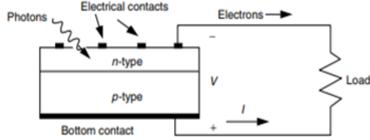
Şekil 3.3. Foton etkisi ile oluşan elektrik akımı (Quaschnig, 2014)
