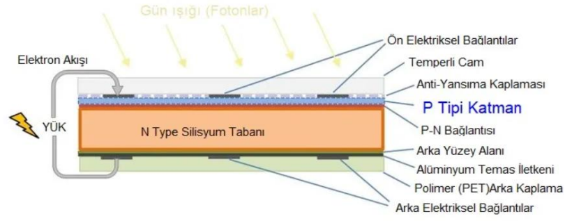
Şekil 2.7. FV P-N hücreleri.
