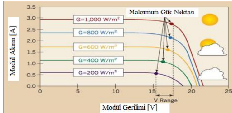
Şekil 3.4. Güneş radyasyonunun FV hücrelerinin gerilimi ve akımı üzerindeki etkisi.
