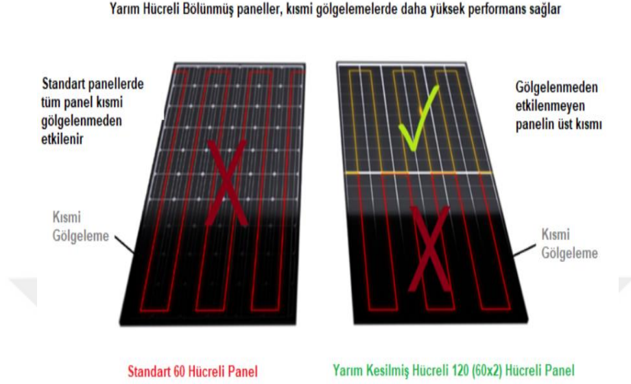
Şekil 2.8. Bölünmüş hücreli güneş paneli [40].
