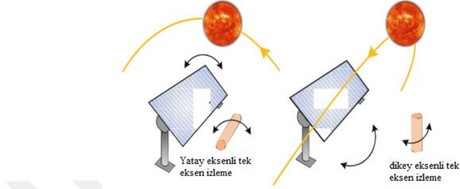
Şekil 3.11. Tek eksenli güneş takip sistemi [81].
