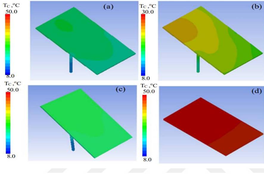
Şekil 3.21. Farklı eğim açıları için modül yüzeyindeki sıcaklık : (a) 15°, (b) 15°, (c) 35° [34].
