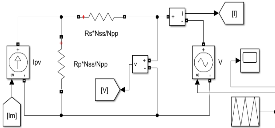
Şekil 3.14. Güneş hücresinin eşdeğer devresi.
