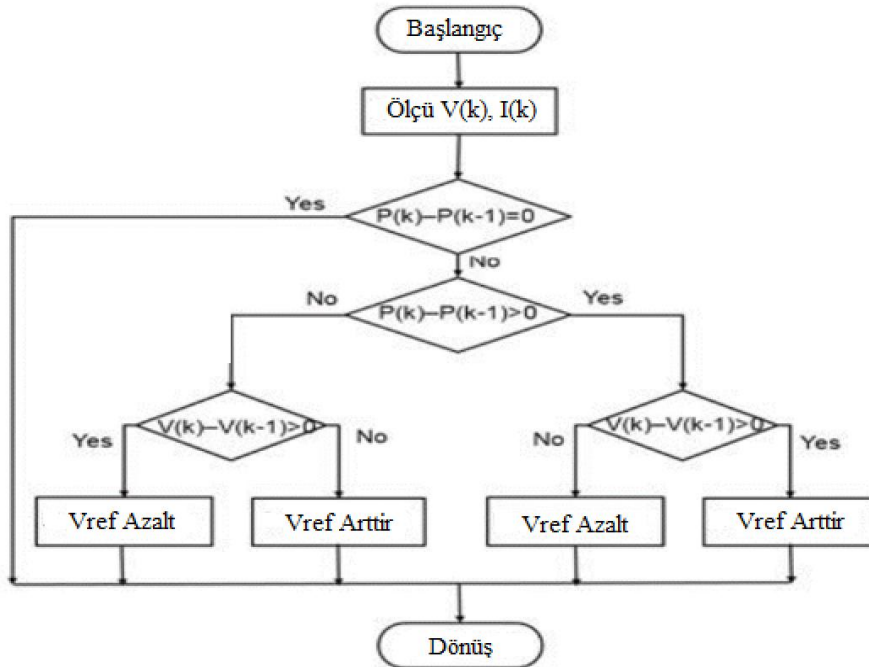
Şekil 3.9. Pertürbasyon ve gözlem algoritmaları diyagramı [23].
