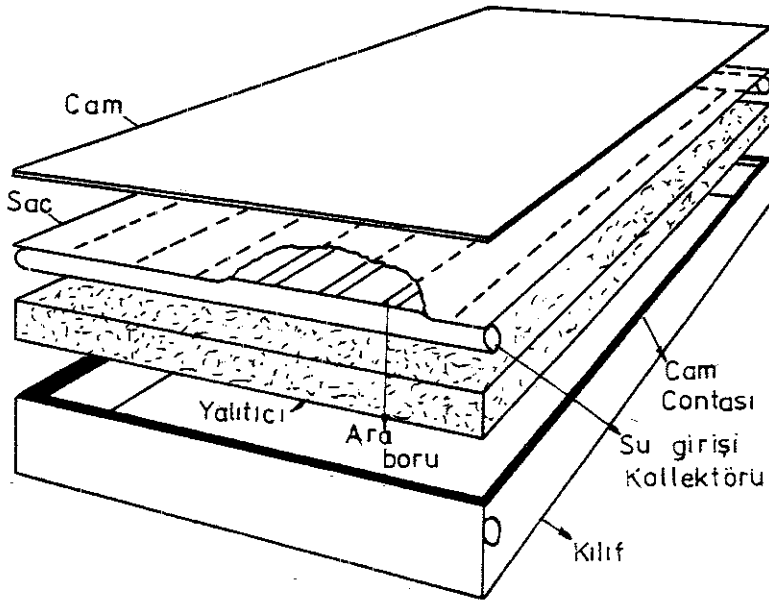
Şekil 4. Güneş kollektörü
