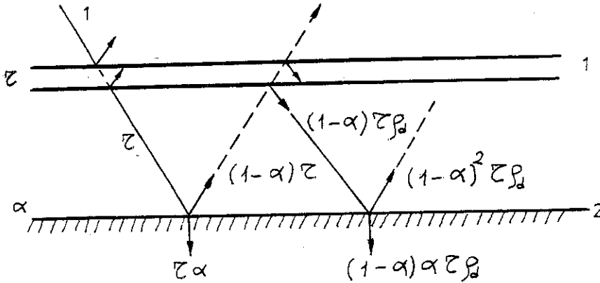
Şekil 7. Güneş ışınının camdan geçmesi ve yansması ile absorberde yutulması ve yansması.
