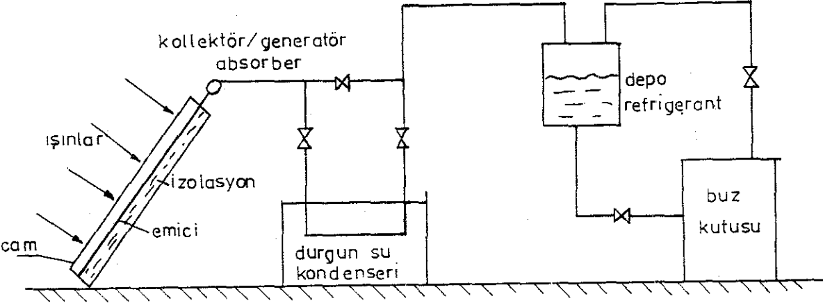
Şekil 33. Kesikli absorpsiyon sistemi şeması (6).
