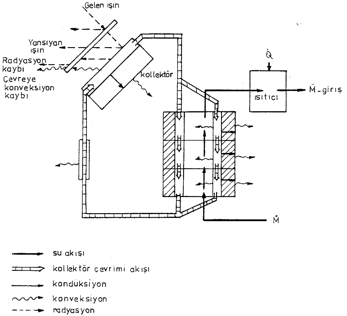
Şekil 12.Genel kollektör kayıpları.
