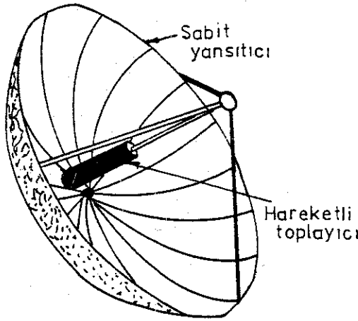
Şekil 18. Yoğun toplayıcı
