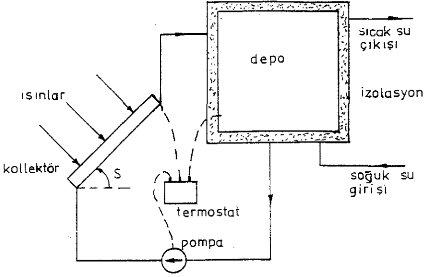
Şekil 14. Zoraki dolaşımlı sistemin şematik görünüşü
