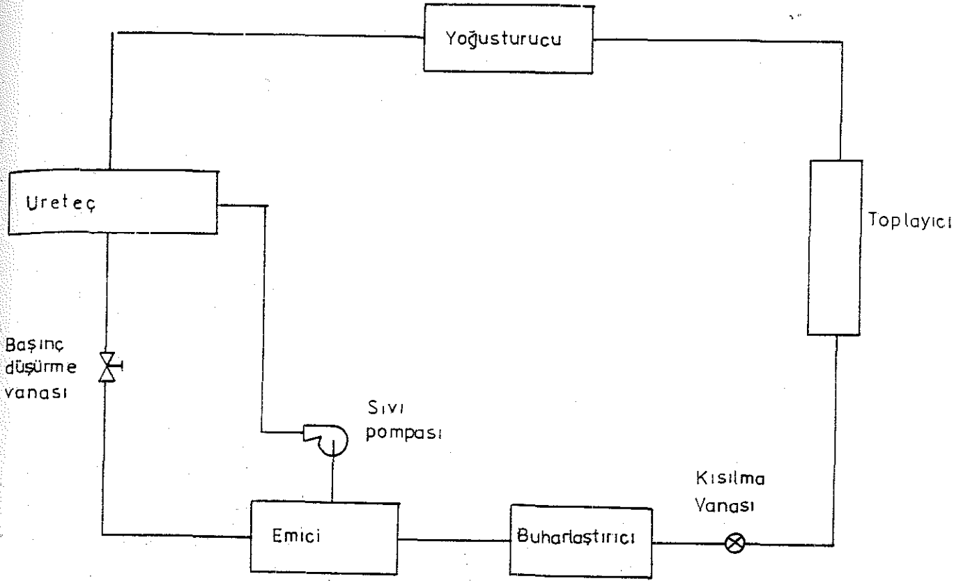
Şekil 29. Basit absorpsiyonlu soğutma çevrimi
