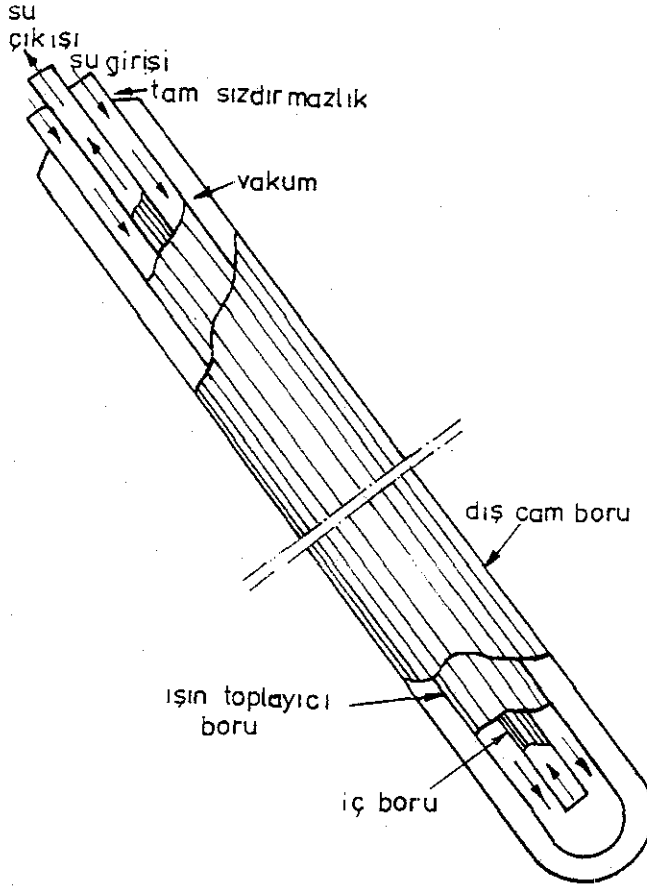
Şekil 20. Vakum borulu toplayıcılar
