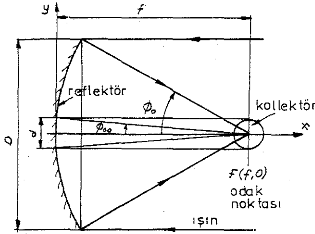
Şekil 17. Silindirik-parabolik reflektör-kollektör sistemi
