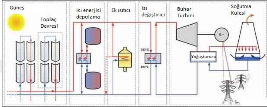
Şekil 4.3 Parabolik oluk topplaç güneş santrali
