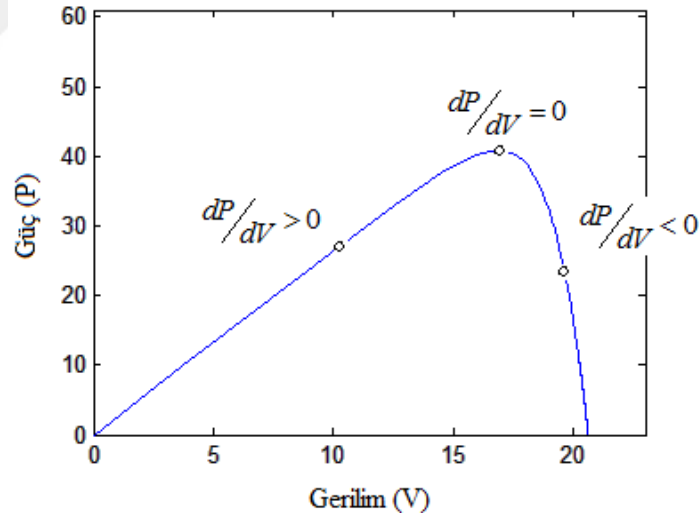
Şekil 3.13 Fotovoltaiik panel güç eğrisi.
