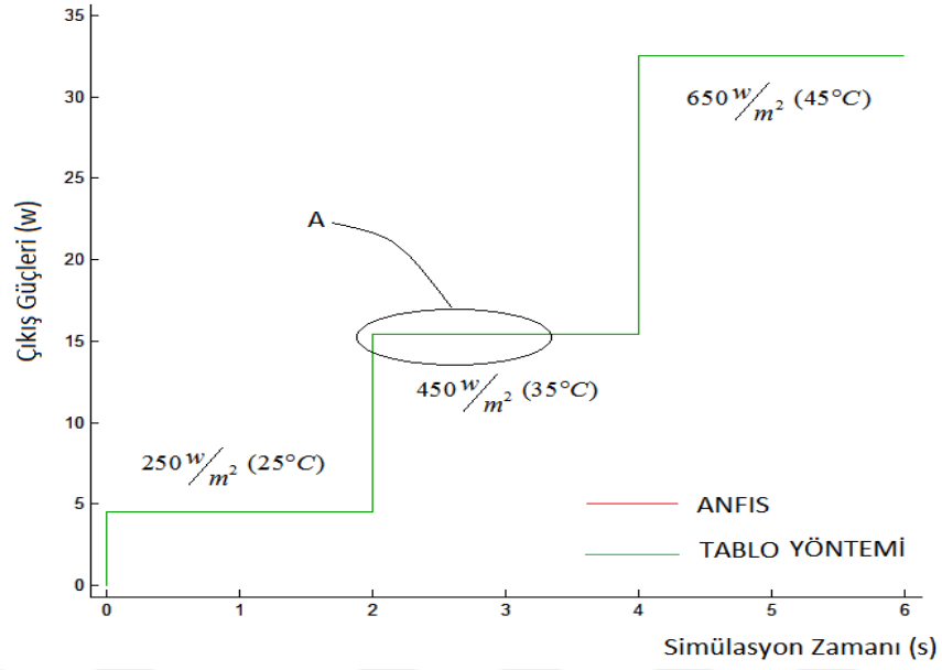
Şekil 4.14 ANFIS ile tablo yönteminin karşılaştırılması.
