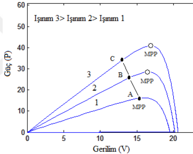
Şekil 3.10 Değişen ışınlam değerlerine karşılık, D&G algoritmasının MPP 'den sapması.
