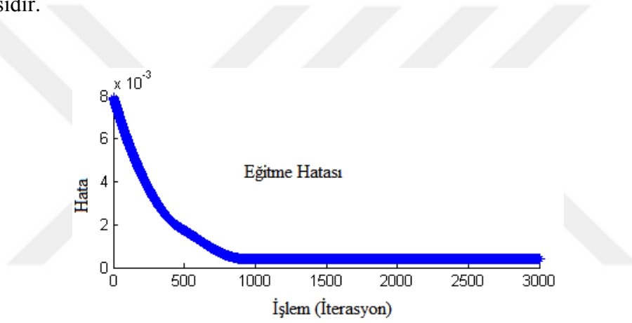
Şekil 4.11 Eğitim işlemi sonrası bulanık mantık sistemi hatası.
