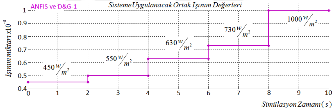
Şekil 4.17 Sistemlere uygulanan farklı ısıtım seviyeleri.
