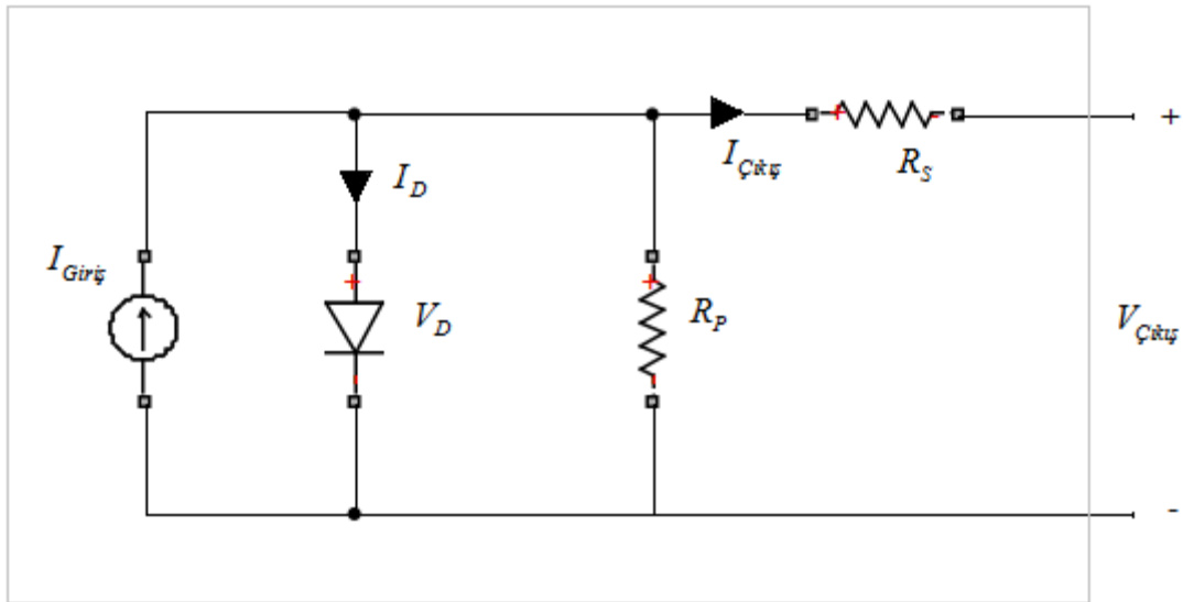
Şekil 3.2 Fotovoltaik güneş hücresi elektriki eş değer devresi (Katan et al. 1996).
