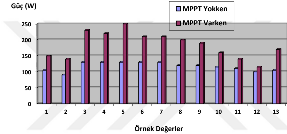
Şekil 3.8 MPPT bulunduran ve bulundurmeyan sistem karşılaştırması (Santos et al. 2006).
