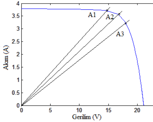
Şekil 3.4 Fotovoltaik pil I-V eğrisi üzerindeki çalışma bölgeleri ve MPP.
