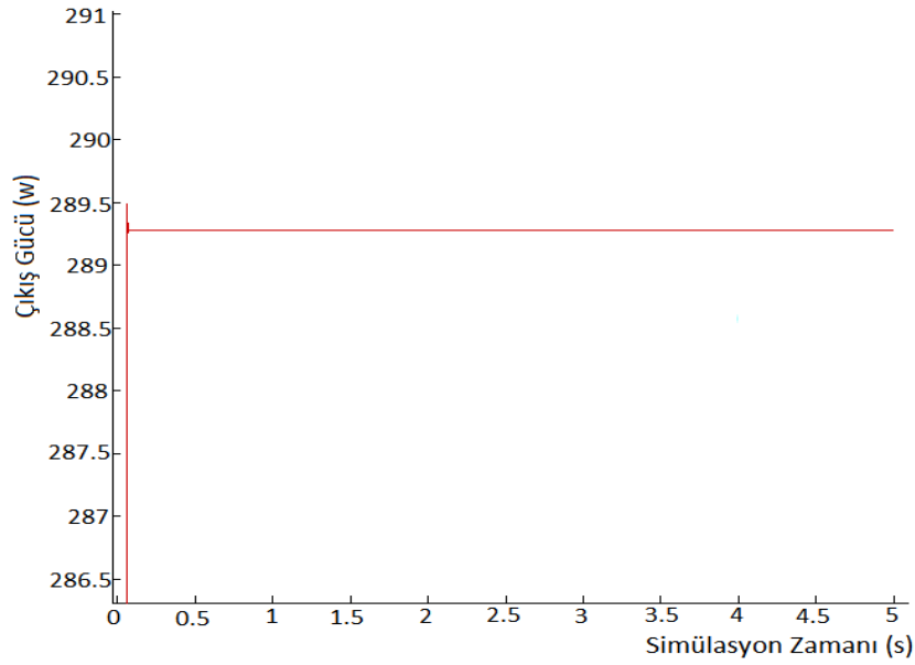
Şekil 4.7 DA-DA yükselten tip çevirici filtre edilmiş çıkış gücü (Duty cycle= 0.5).
