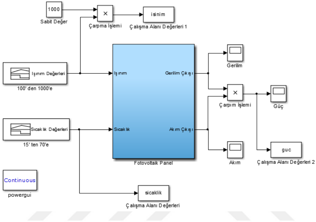
Şekil 3.19 60 Watt'lık panelden eğitim verilerinin alınması.
