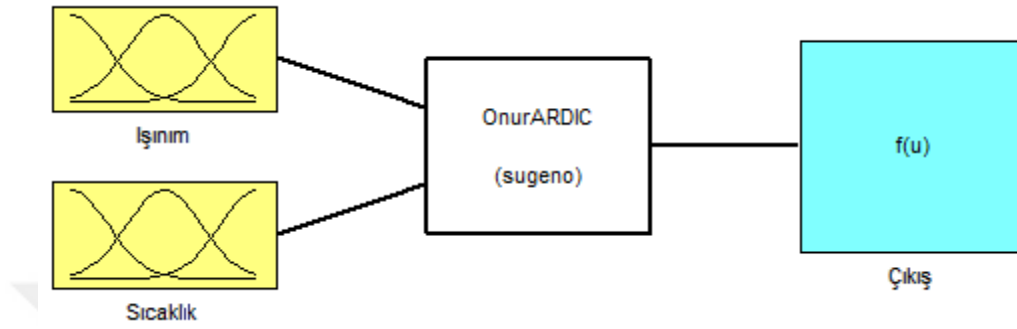
Şekil 3.21 Veriler yüklendikten sonra oluşan bulanık mantık sistemi.
