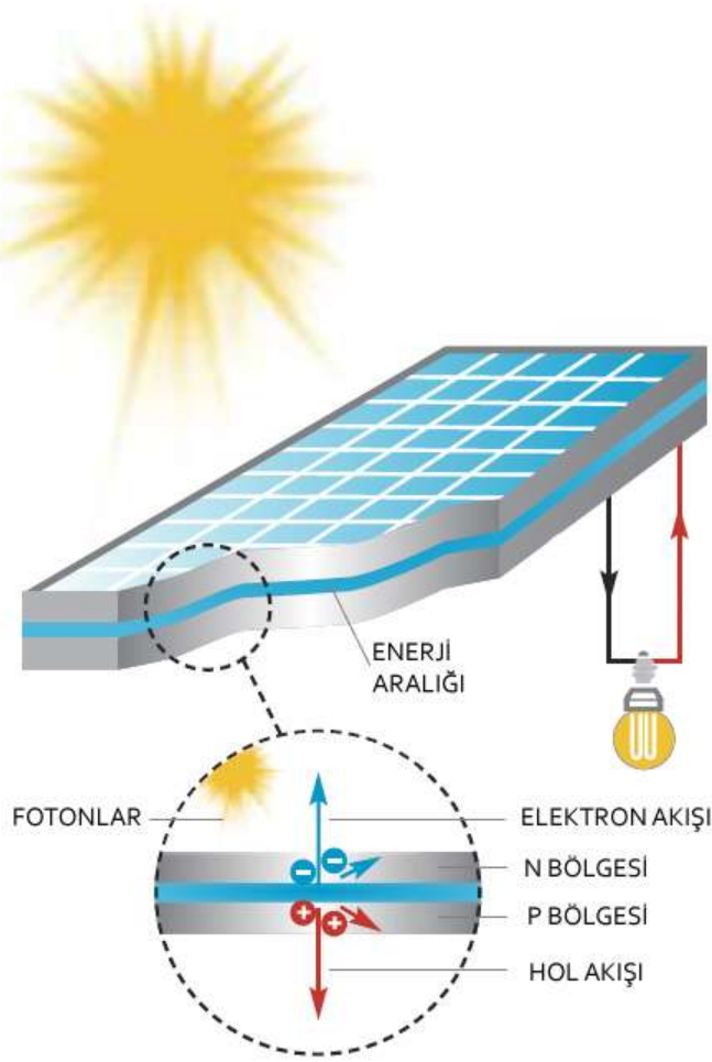
Şekil 2.3. Fotovoltaiik çalışma prensibi [20]
