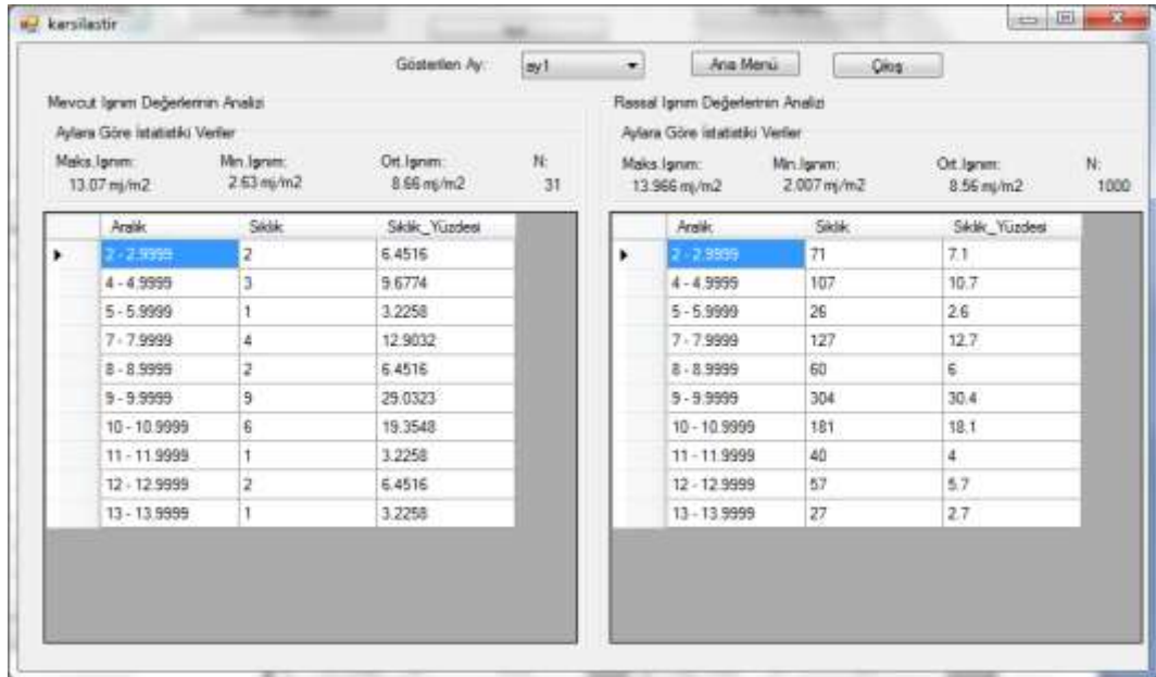
Şekil 5.13. Ocak ayı için benzetim sonucu elde edilen ışıını değeri analizi
