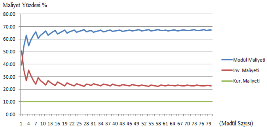
Şekil 5.32. Modül sayısına göre maliyet yüzdeleri
