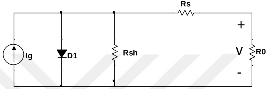
Şekil 3.1. Güneş pili eşdeğer devresi [34]
