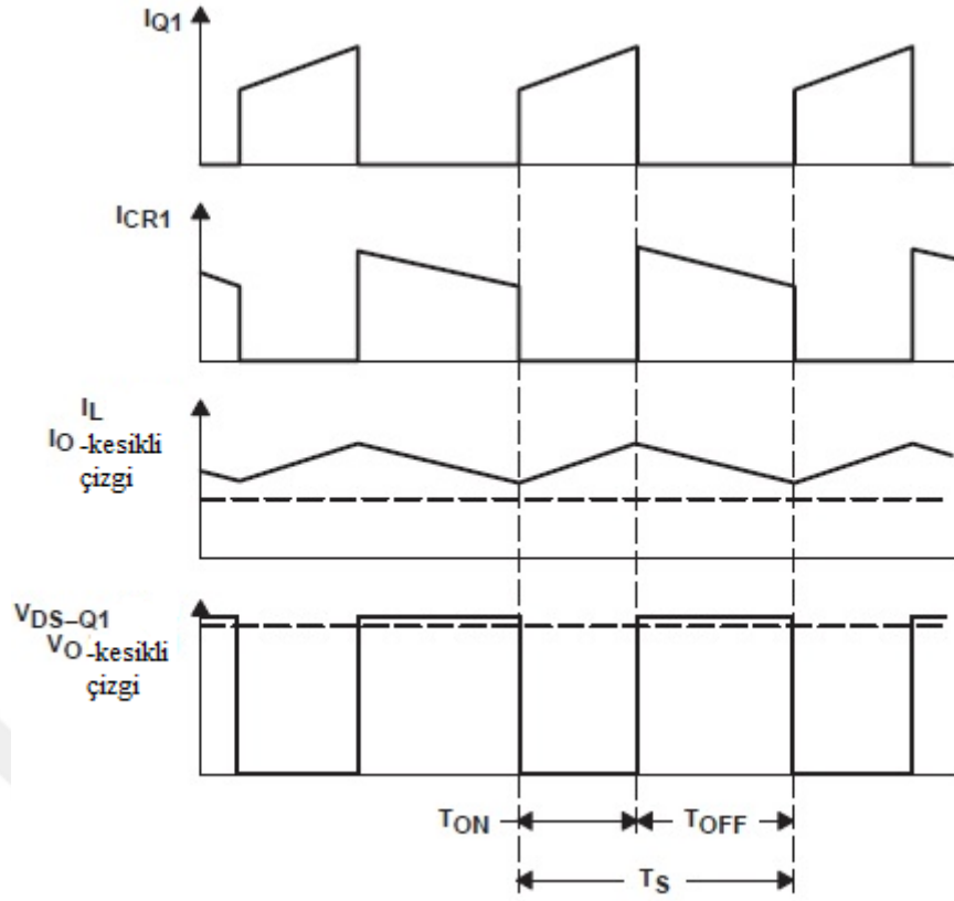
Şekil 3.9. Boost topolojisi dalga formları [38]
