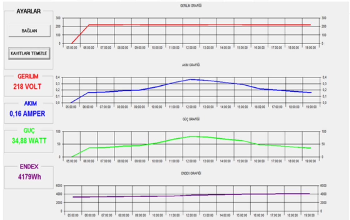
Şekil 4.9. Güneş takip sisteminin bağlı olmadığı panel çıktıları
