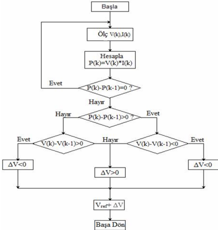
Şekil 2.2. Değiştir-gözle algoritması akış diyagramı [4]
