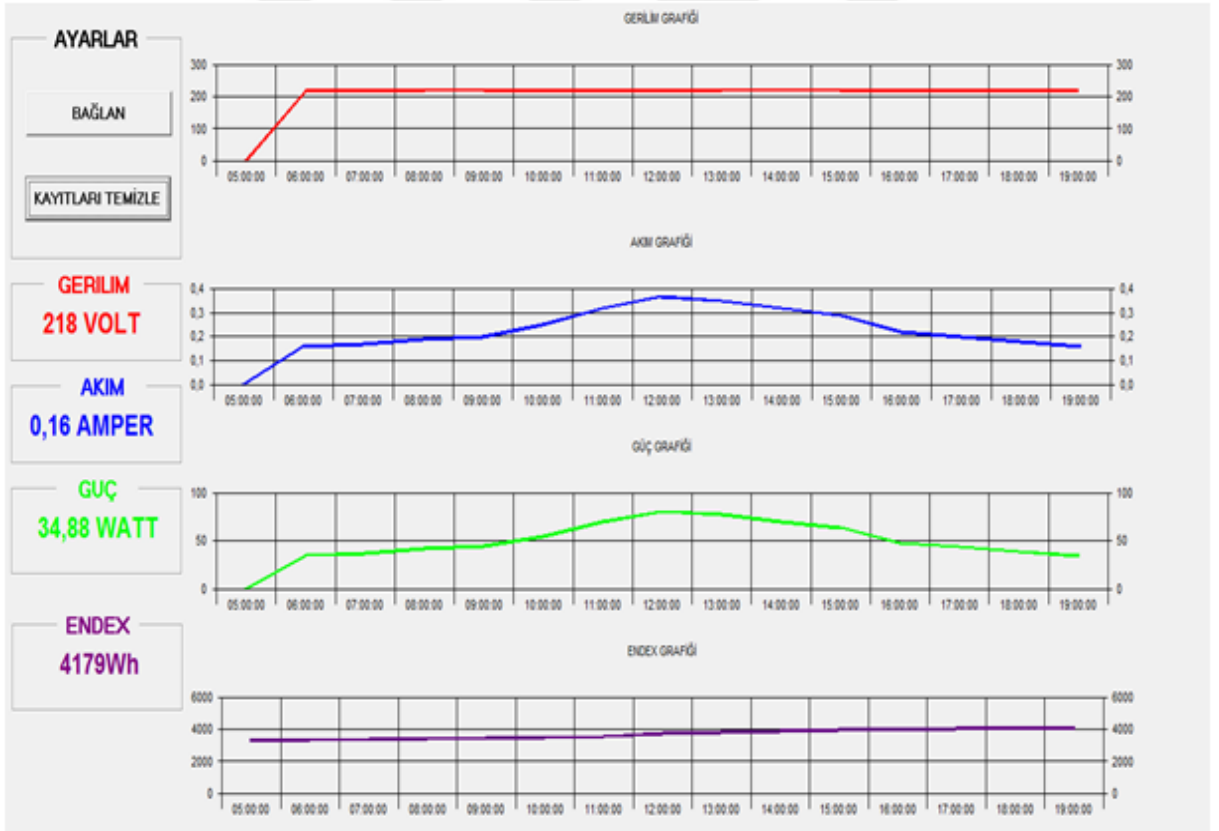
Şekil 4.12. Gölgesiz panele ait çıktılar
