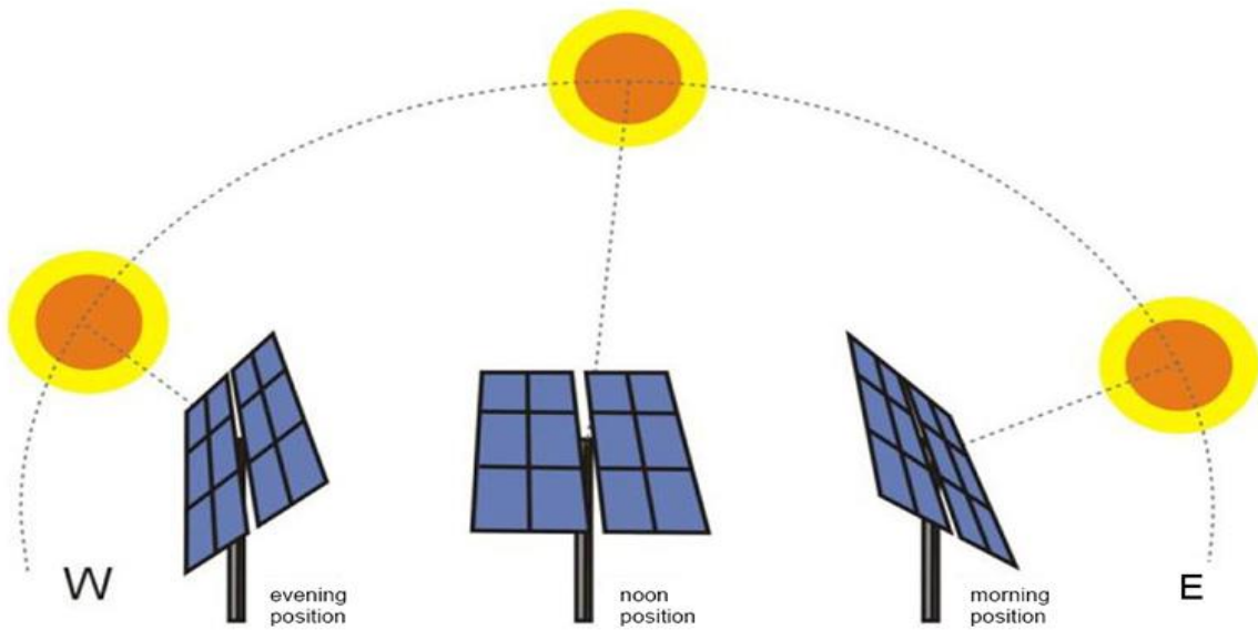
Şekil 2.26. Aktif kontrol sistemi [33]
