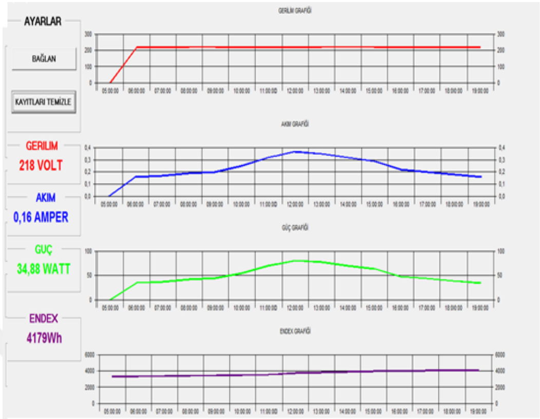
Şekil 4.3. Yüzeyi temiz panel çıktıları
