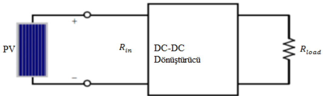
řekil 3.13. PV tarafından grlen empedans
