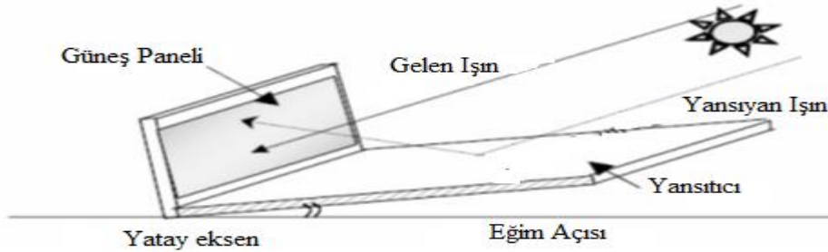
Şekil 2.18. Sabit panellerin yansıtıcı ile birlikte kullanımı [29]
