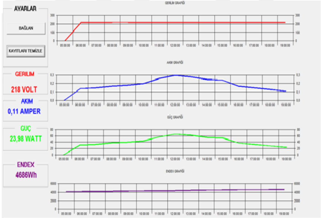
Şekil 4.4 Yüzeyi 10g tozla kaplı panel çıktıları
