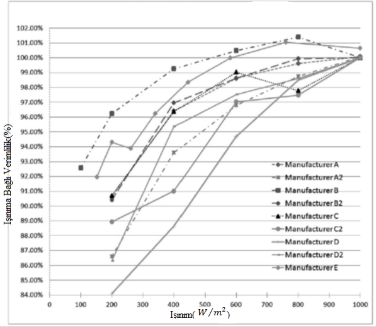
Şekil 2.13. Güneş hücrelerine ait 9 adet katalogun spektral verileri [15]
