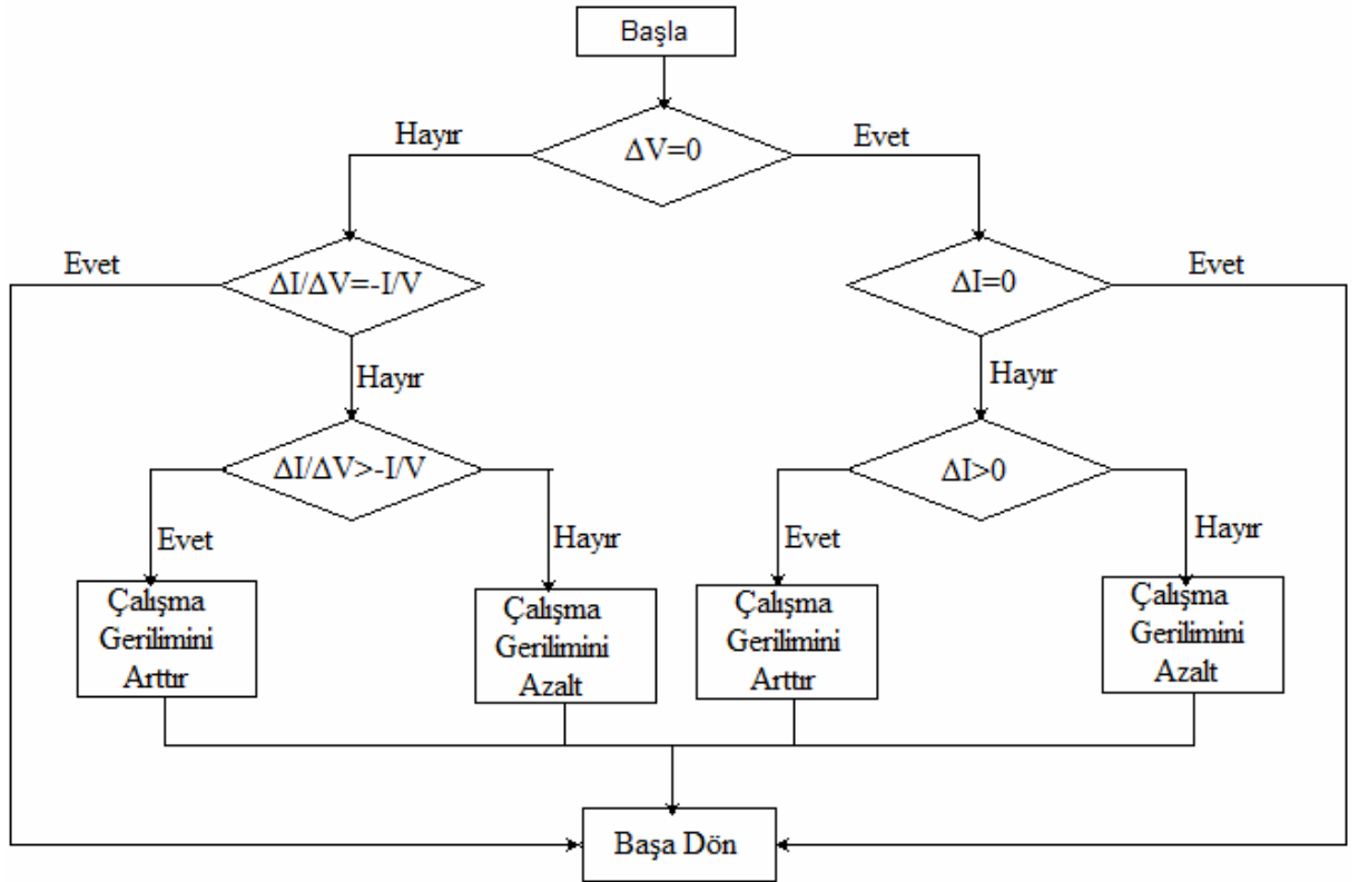
Şekil 2.4. Artan iletkenlik akış diyagramı [9]
