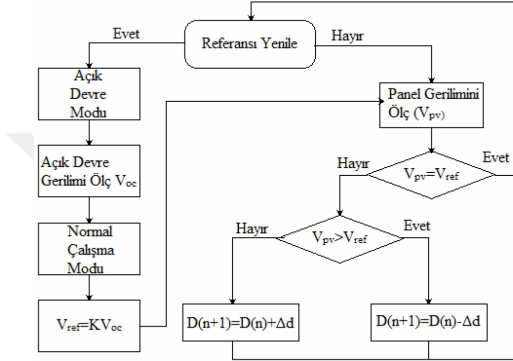
Şekil 2.5. Sabit gerilim algoritması akış diyagramı [9]
