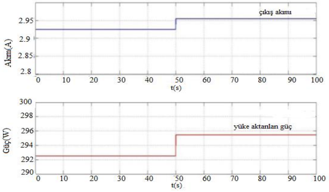
Şekil 4.15. MGNT olmadan yapılan ilk uygulama sonuçları
