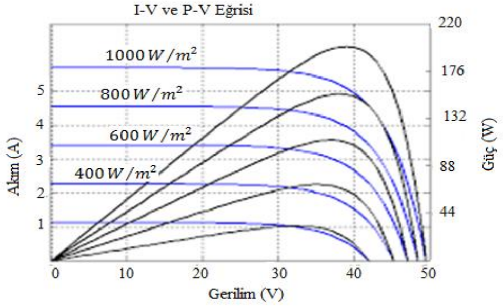
Şekil 3.3. Işınmının I-V ve P-V eğrisine etkisi [35]
