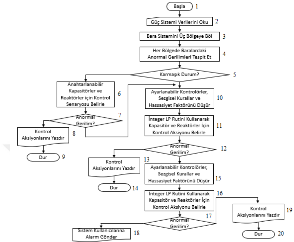
Şekil 2.5. Sonuç Motorunun Gerilim Regülasyonunu Gerçekleştirmek için Kullanılan Kontrol Algoritmasına ait Akış Şeması
