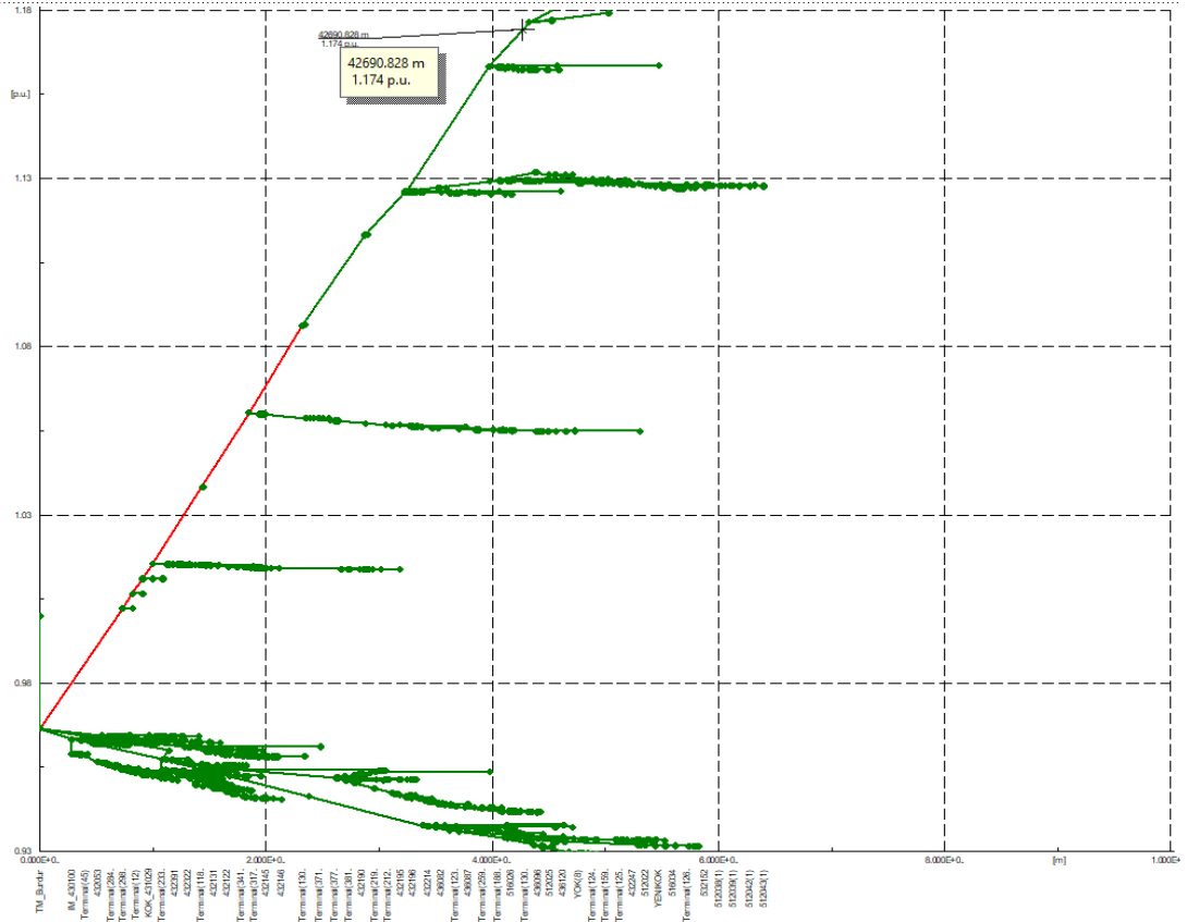
Şekil 4.26. İnverterlerin Endüktif Çalışması Durumunda Oluşan Gerilim Profili
