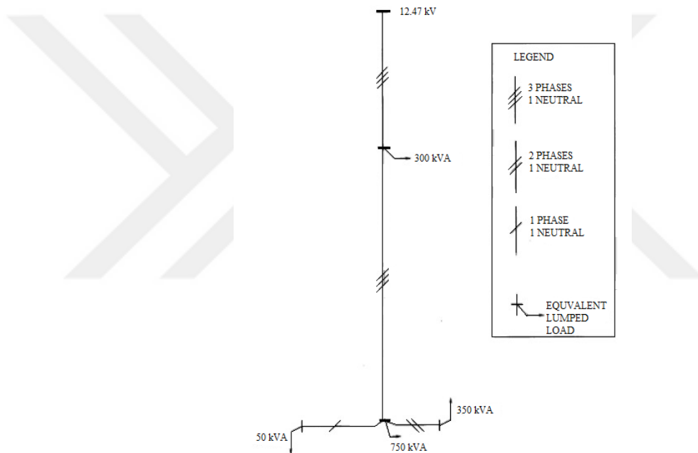
Şekil 3.4. Gerilim Düşümü Hesaplamasında Kullanılacak Sadeleştirilmiş Tek Hat Şeması
