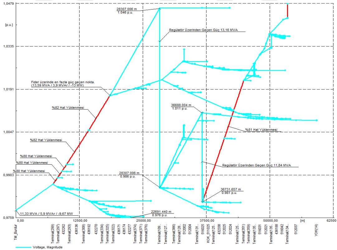
Şekil 4.8. Tümü GES'ler ve İki Oto Trafo Aktif Durumda Saat 12:00'de Oluşan Gerilim Profili
