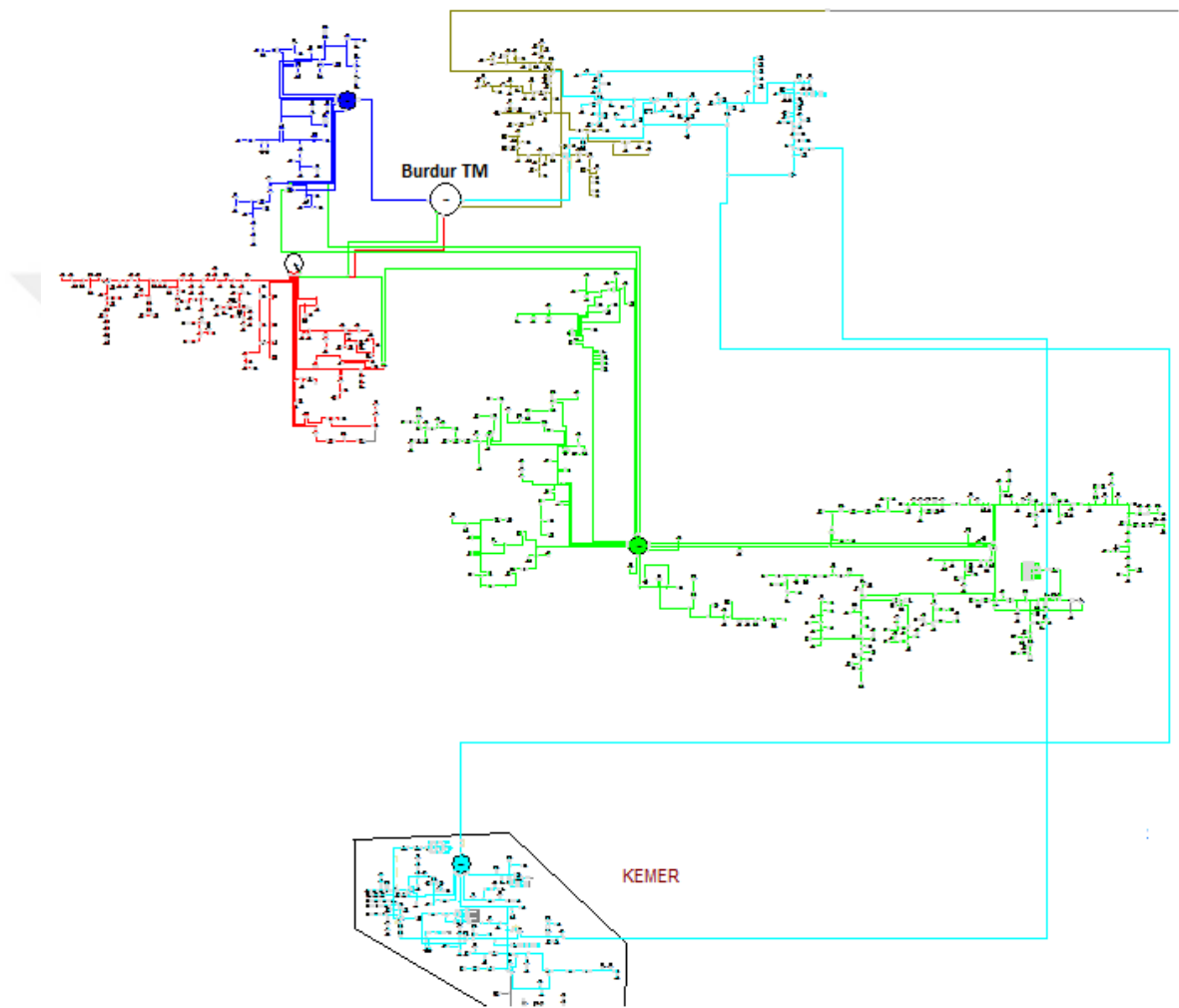
Şekil 3.6. Burdur TM DigSILENT PF Modeli
