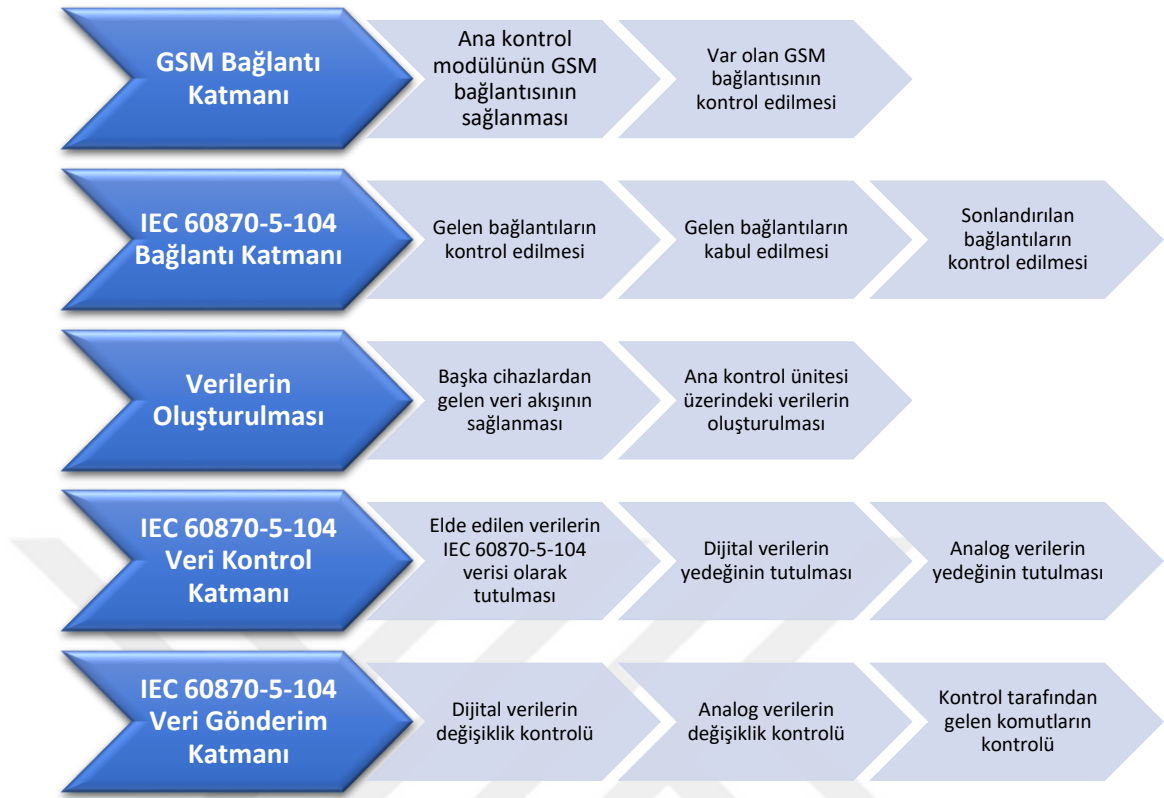
Şekil 3.10. Ana Kontrol Modülü IEC 60870-5-104 Yazılım Katmanları
