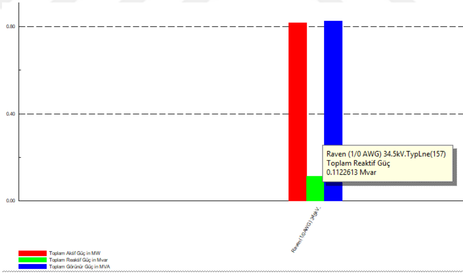
Şekil 4.22. Hat Üzerindeki Toplam Aktif, Reaktif ve Görünür Güçler
