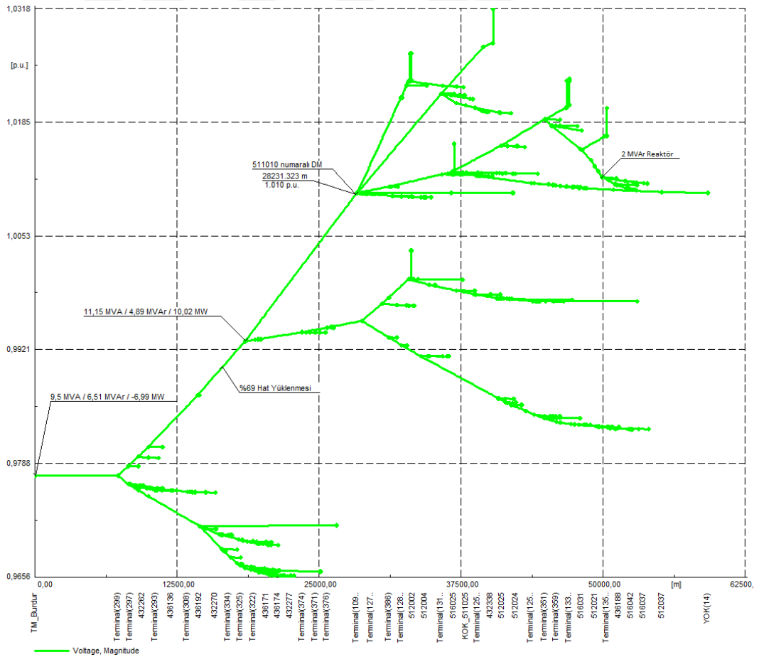
Şekil 4.19. Alternatif Durumda GES Üretimleri %80 ile Sınırlandırılmış ve 2 MVar Reaktör0 Aktif Durumdayken Oluşan Gerilim Profili
