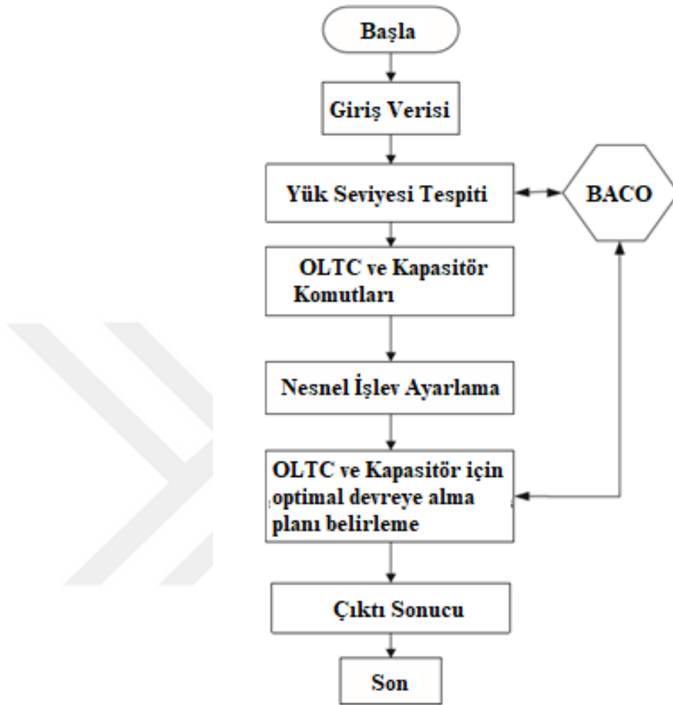
Şekil 2.7. Volt/VAR Kontrol Algoritması Akış Şeması
