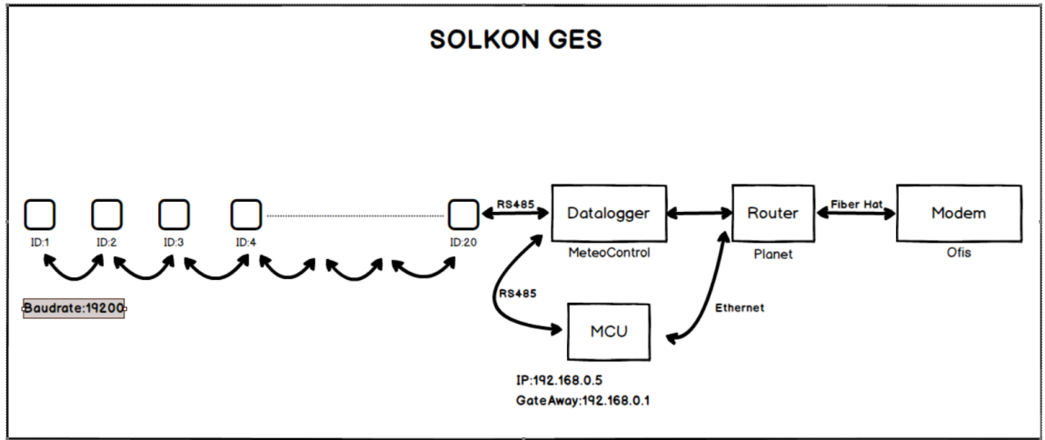
Şekil 3.9. Sistem Yapısı
