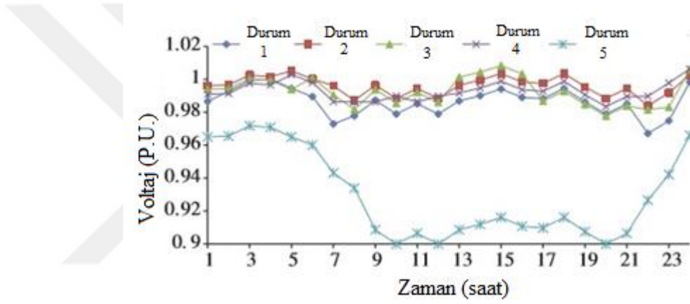
Şekil 2.8. IEEE 33-Baralık Şebekesinde Gerçekleştirilen Simülasyon Sonucu 18. Baradan Elde Edilen Saatlik Gerilim Profili
