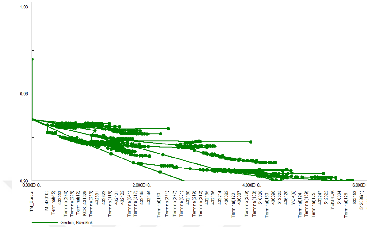
Şekil 4.21. Santraller Devrede Değilken Fiderin Gerilim Profili
