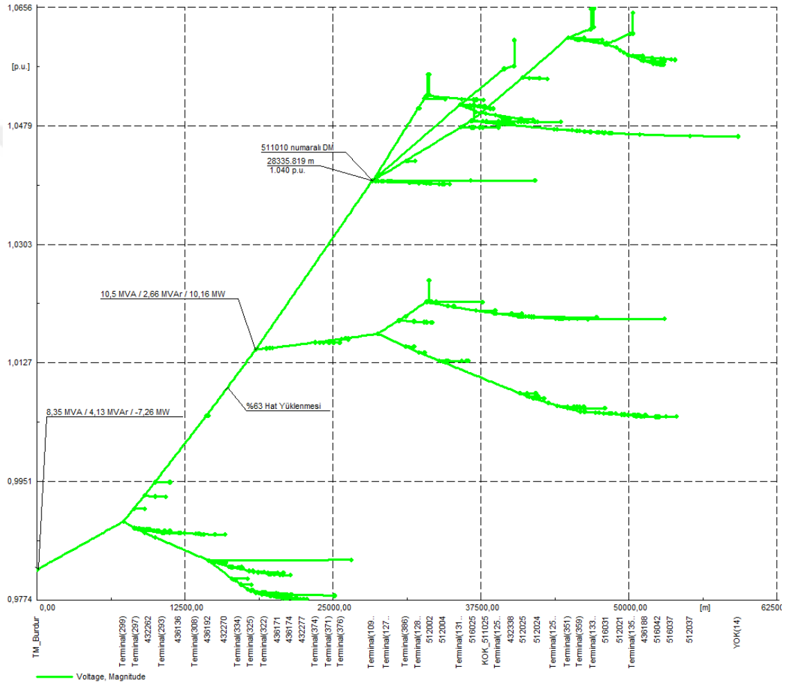
Şekil 4.18. Alternatif Durumda Tüm GES'lerin Üretimi %80 ile Sınırlandırılmış Durumda Saat 12:00'de Oluşan Gerilim Profili
