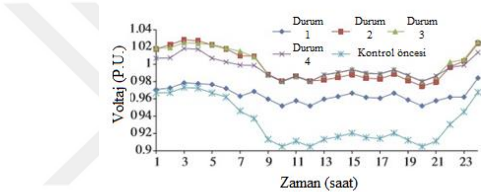
Şekil 2.10. IEEE 33-Baralılık Şebekesinde Gerçekleştirilen Simülasyon Sonucu 65. Baradan Elde Edilen Gerilim Profili
