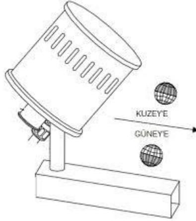
Şekil 6 Güneşlenme Zamanı Sensörü montaj şematigi [6].
