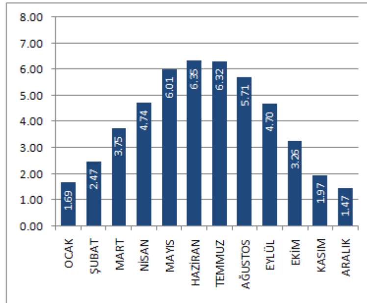
Şekil 16 Diyarbakır Global Radyasyon Değerleri (KWh/m 2 -gün) [12]
