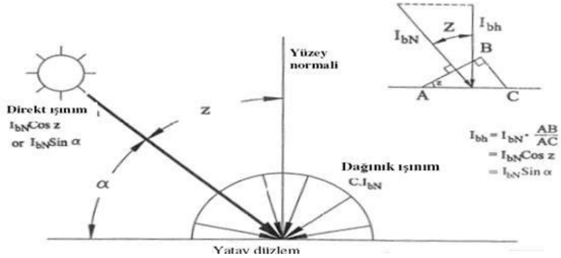
Şekil 3.19. Yatay bir düzlemde güneş ışıınımı
