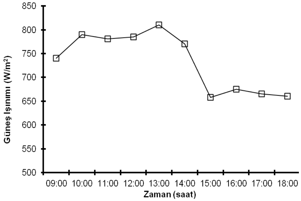
Şekil 4.41. 27/05/2012 tarihine ait hareketli düzlemsel kolektörüne ait güneş ışıınımlı değlerleri
