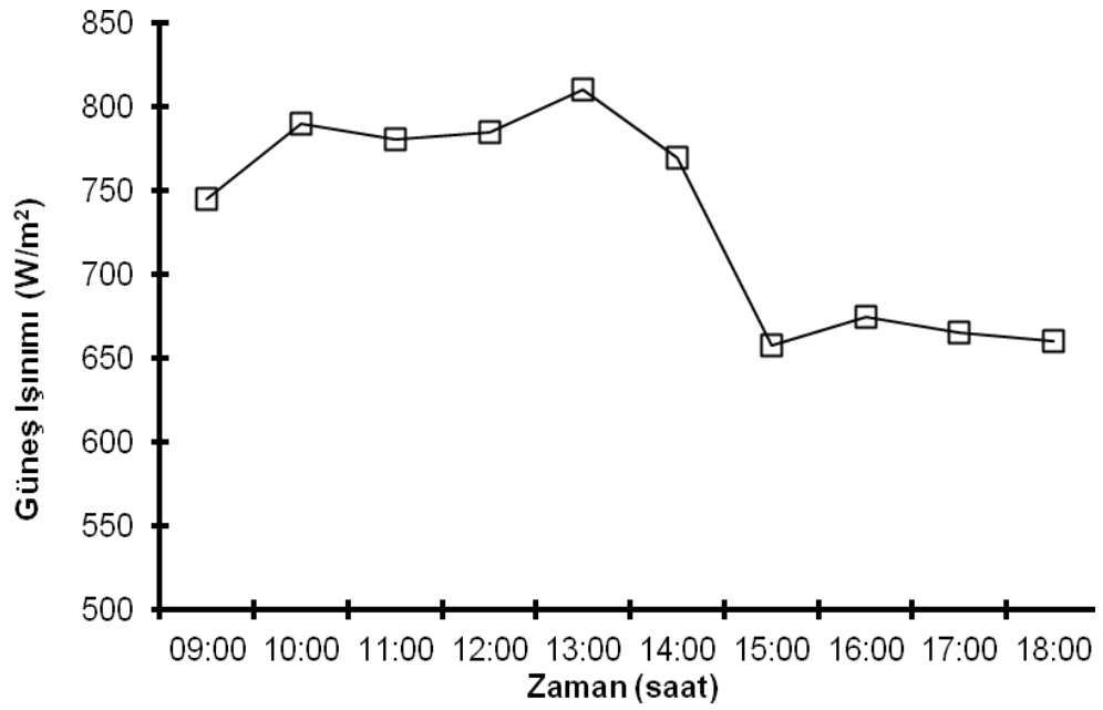
Şekil 4.35. 20/05/2012 tarihine ait hareketli düzlemsel kolektörüne ait güneş ışıınımlı değerleri
