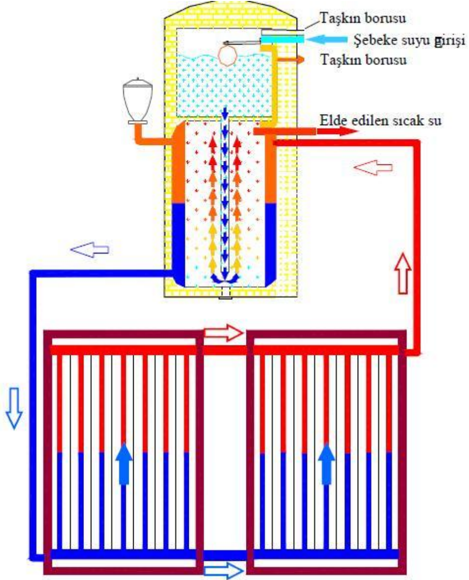
Şekil 2.11.b. Tabi dolaşımli güneş enerjisi şeması
