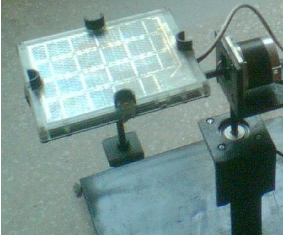
Şekil 3.18. Gerçekleştirilen kapalı döngü sistem
