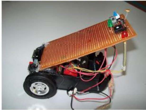
Şekil 4.25. Oyuncak araba güneş takip düzeneği yandan görünüş
