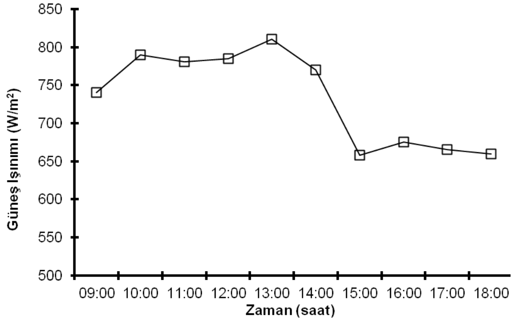
Şekil 4.38. 23/05/2012 tarihine ait sabit düzlemsel kolektörüne ait güneş ışıınımlı değlerleri
