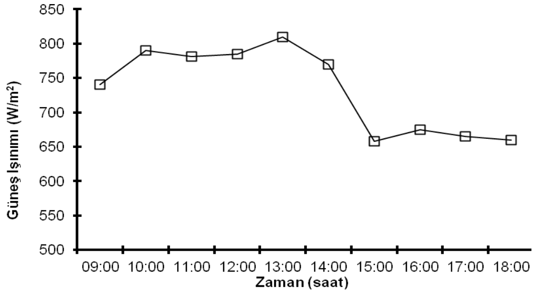
Şekil 4.32. 18/05/2012 tarihine ait sabit düzlemsel kolektörüne ait güneş ışınlımı değerleri
