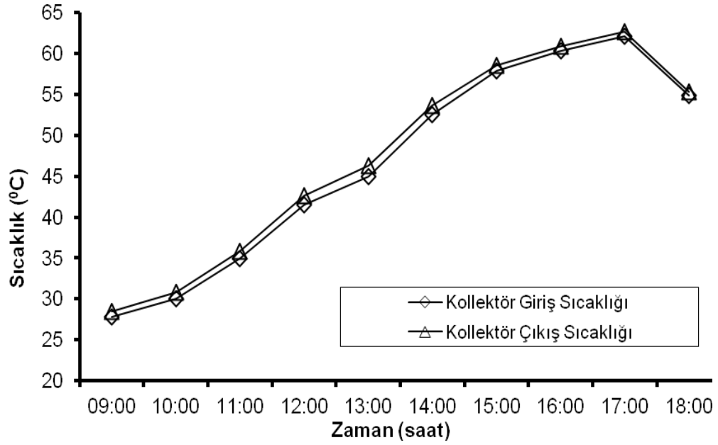
Şekil 4.39. 23/05/2012 tarihine ait sabit düzlemsel kolektörüne ait giriş sıcaklığı ve çıkış sıcaklığı karşılaştırılması.
