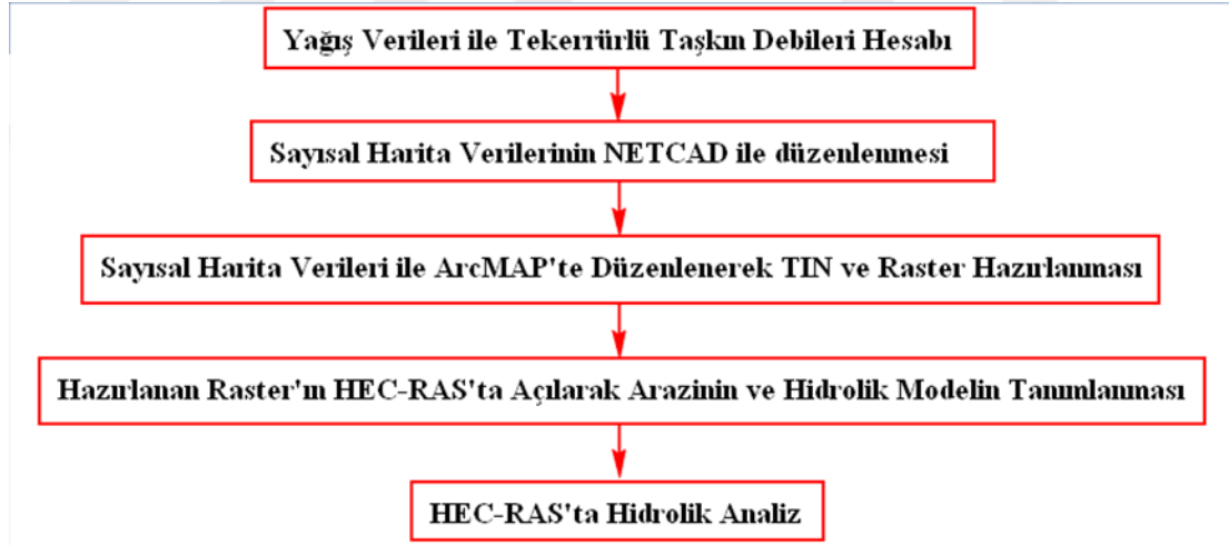
Şekil 6.2. Çalışma diyagramı
