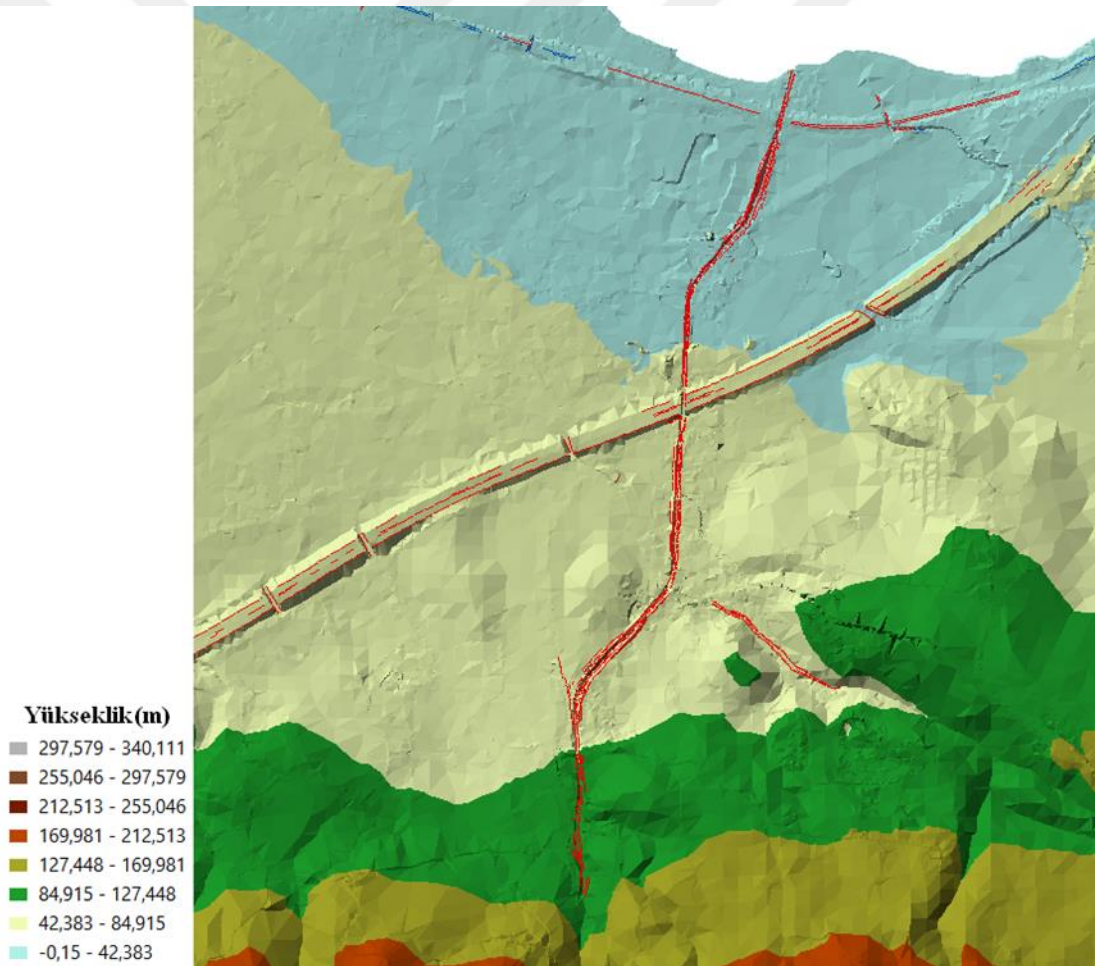
Şekil 6.4. TIN Verisine genel bakış
