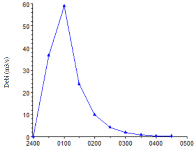
Şekil 6.1. Keçi Deresi Q500 taşkın hidrografi
