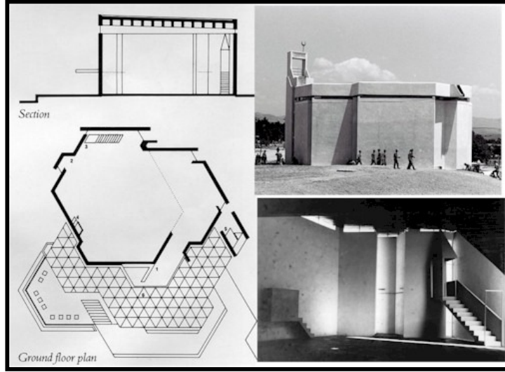
Şekil 3.58 Etimesgut Camii plan şeması, kesit ve görünüşler (www.arkitera.com)
