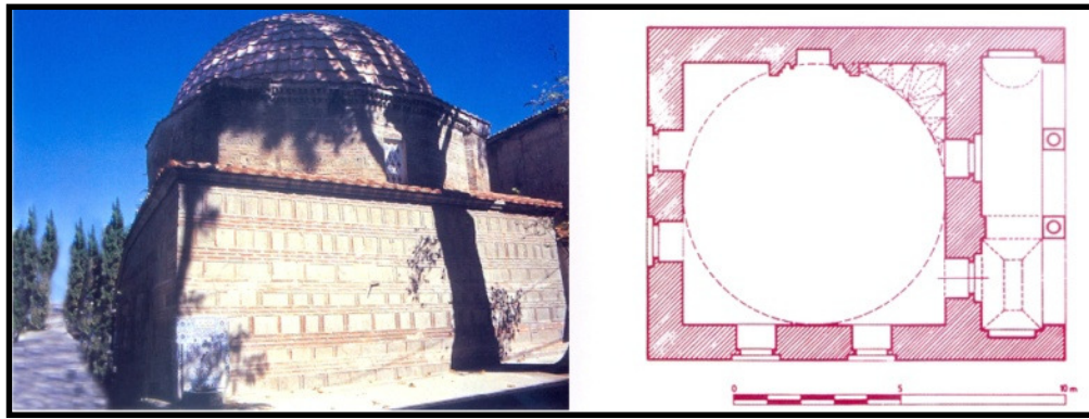
Şekil 3.31 Hacı Özbek Camii dış görünüş ve plan şeması (O. Aslanapa)
