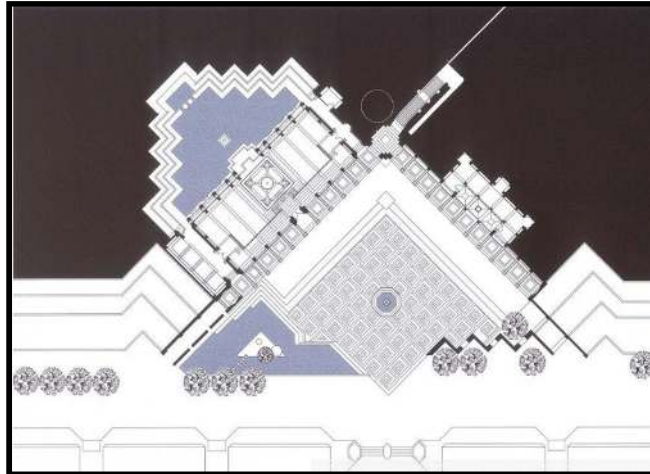
Şekil 4.18 TBBM Camii plan şeması (www.arkitera.com)
