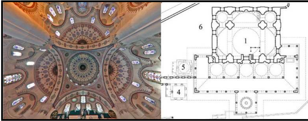
Şekil 3.43 Mihrimah Sultan Camii kubbe iç görünüşü ve plan şeması ( http://wowturkey.com )
