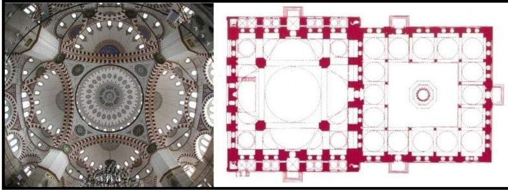
Şekil 3.45 Şehzade Camii kubbe iç görünüşü ve plan şeması (O. Aslanapa)
