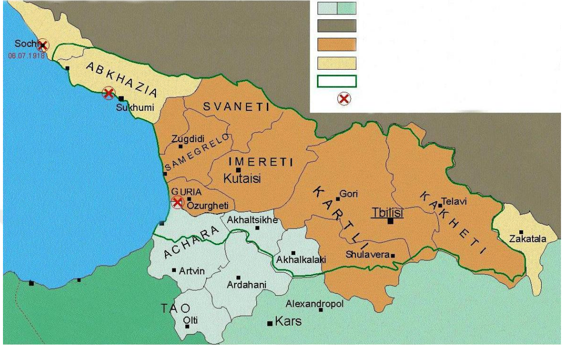
Resim4: GürcistanHaritasi
