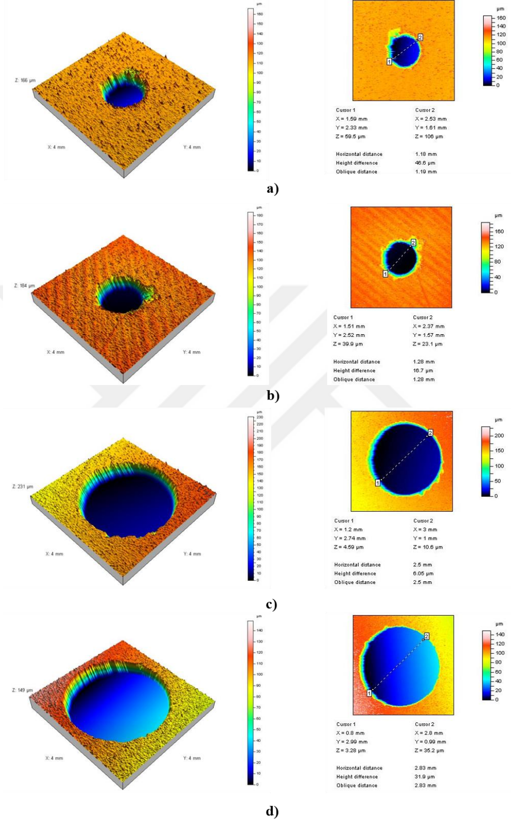
Şekil 5.34. 1350 °C’de 90 dk süre ile sinterlenmiş ve matkapla işlenmiş a) BN 5, b) BN 10, c) BN 15 ve d) BN 20 numunelerinin 3D profilometre görüntüleri
