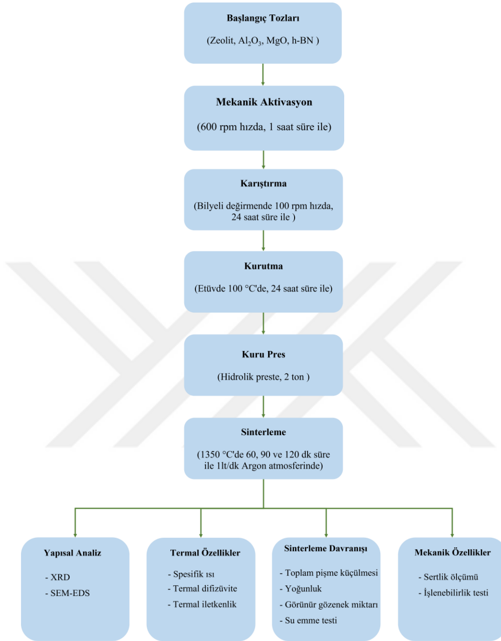
Şekil 4.1. Çalışma esnasında takip edilen işlemlerin şematik gösterimi
