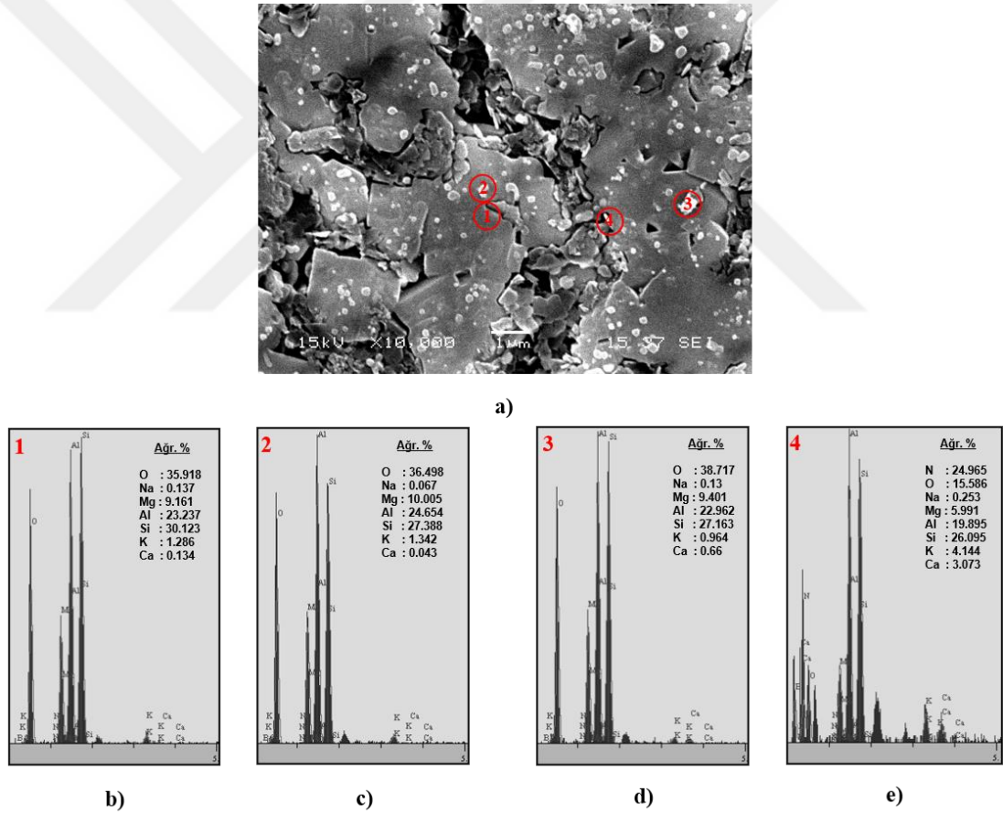
Şekil 5.18. 1350 °C'de 60 dk süre ile sinterlenmiş BN 5 numunesinin a) SEM mikrofrafisi, b) 1 numaralı, c) 2 numaralı, d) 3 numaralı ve e) 4 numaralı noktaların EDS analizi
