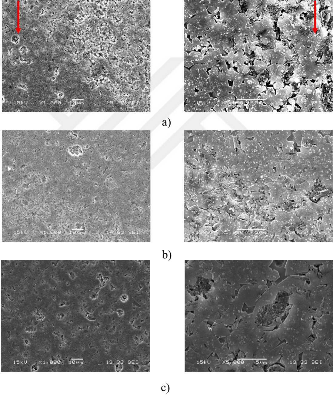
Şekil 5.14. 1350 °C'de a) 60, b) 90 ve c) 120 dk süre ile sinterlenmiş BN 5 numunesinin SEM mikrografları
