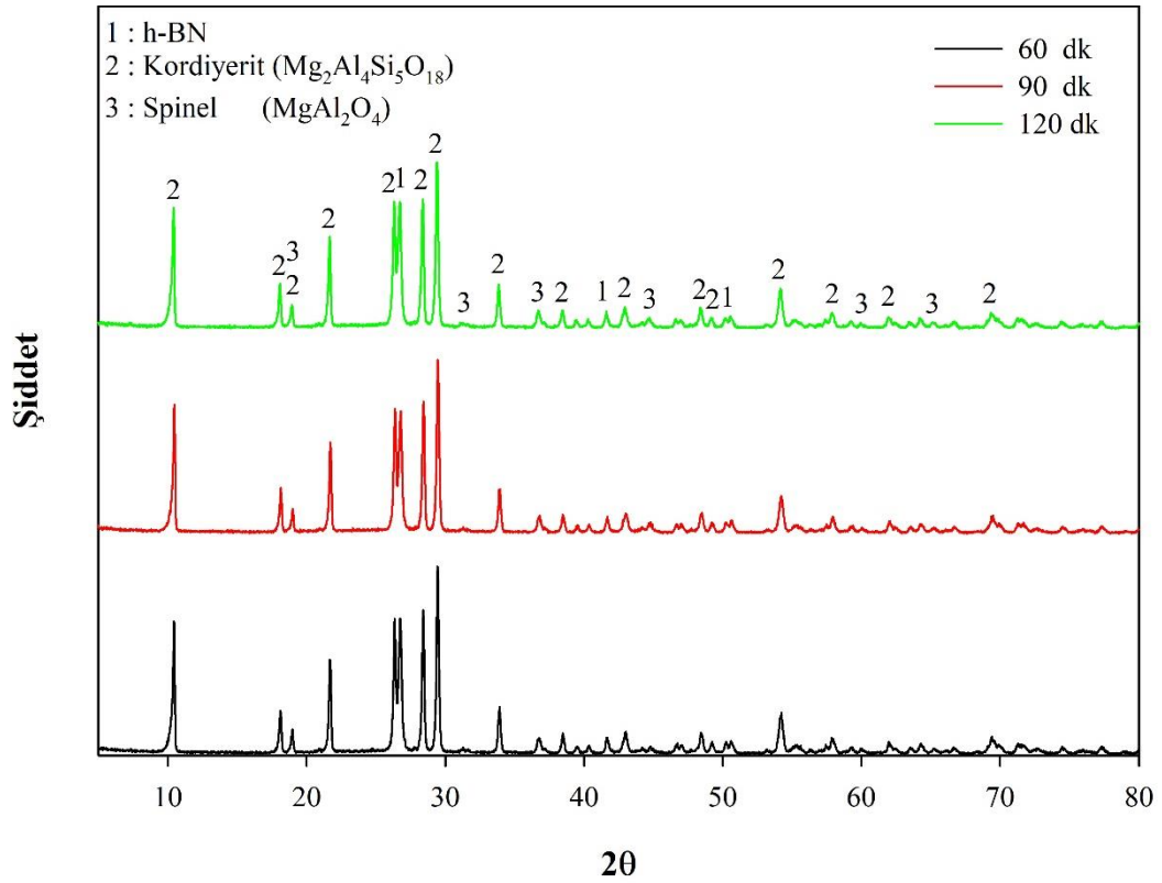
Şekil 5.8. Üç farklı sürede sinterlenmiş BN 20 numunesinin XRD paternleri
