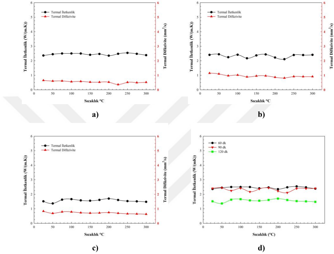
Şekil 5.27. 1350 °C’de a) 60 dk b) 90 dk c) 120 dk süre ile sinterlenmiş BN 5 numunesinin termal iletkenlik ve termal difüzyivite değişimi ve d) farklı sürelerde sinterlenmiş BN 5 numunesinin karşılaştırmalı termal iletkenlik grafiği
