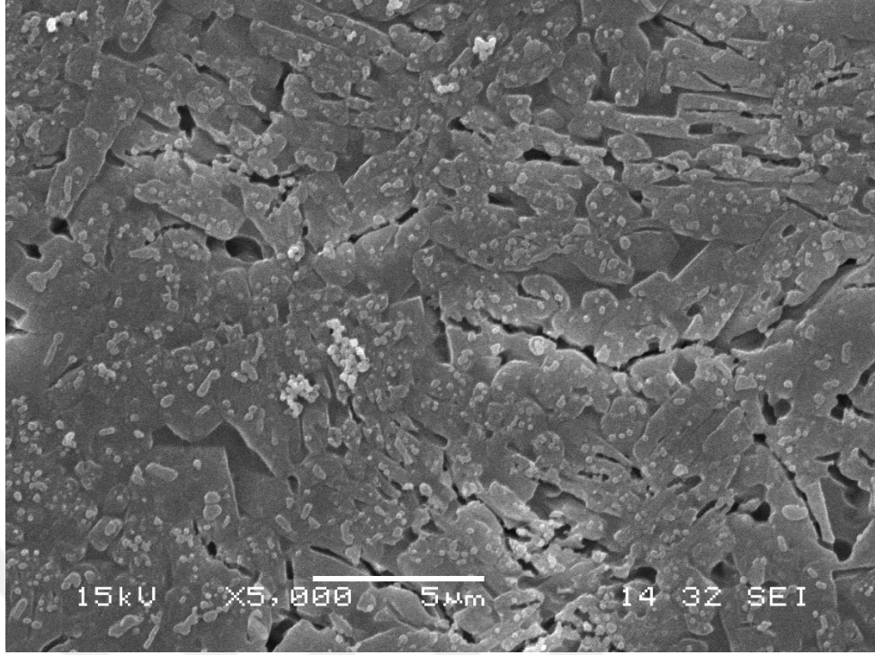
Şekil 5.9. 1350 °C’de 60 dk süre ile sinterlenmiş katkısız numunenin SEM mikrografı
