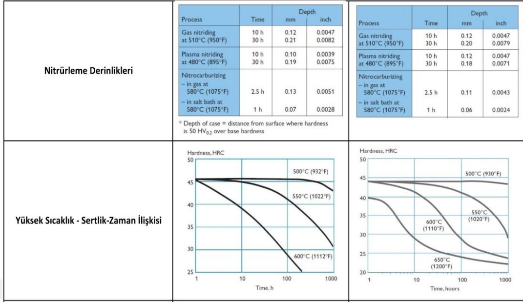
Şekil 4.3. (c) 1.2340 & 1.2344 Malzeme kıyaslaması – nitrüleme derinlikler ve sıcaklık sertlik zaman derinlikleri
