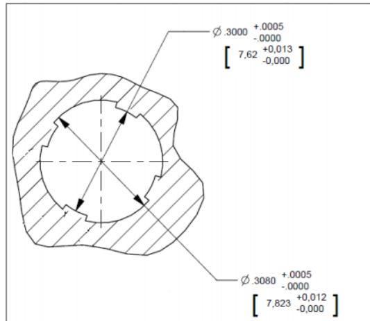
Şekil 3.3. Namlu Yiv-Set Geometrisi
