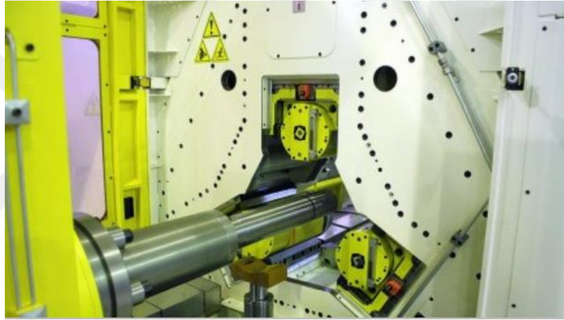
Şekil 3.9. Akıtarak sıvama tezgahı
