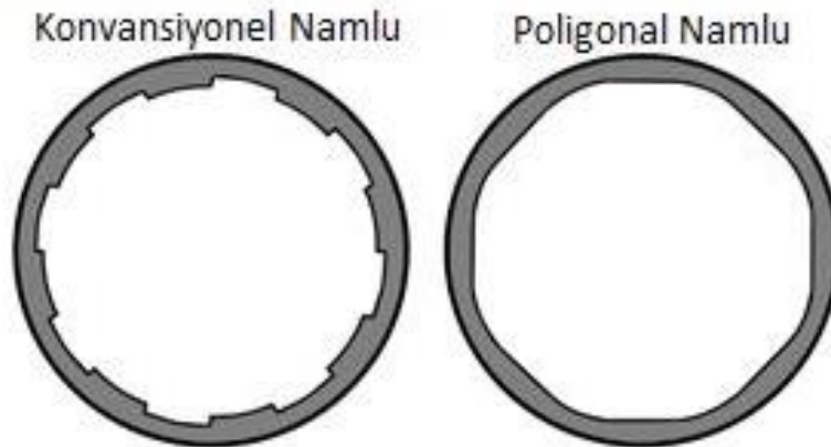
Şekil 2.7. Konvansiyonel namlu ve poligonal namlu geometrileri
