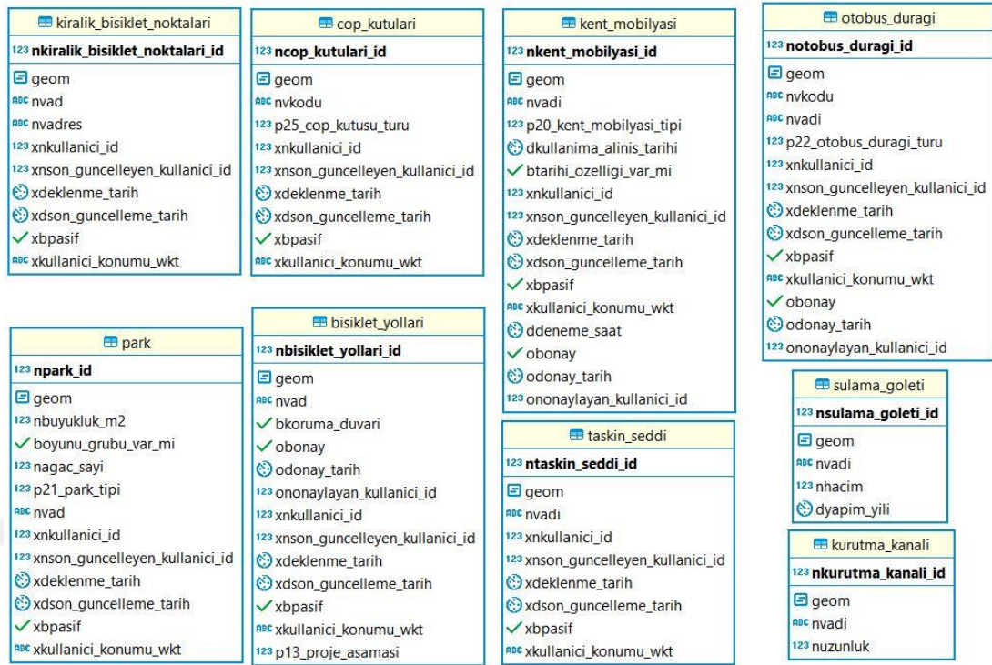
Şekil 3.3. Çalışma içinde oluşturulan örnek veri setlerinin veri modeli.
