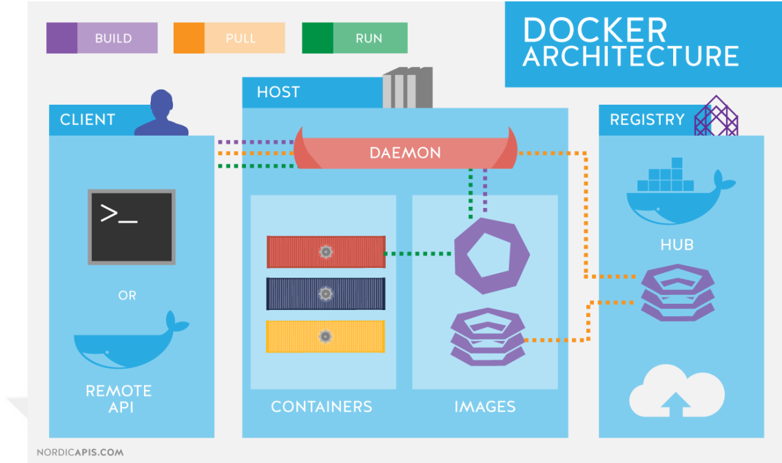
Şekil 2.22. Docker Mimarisi [34]
