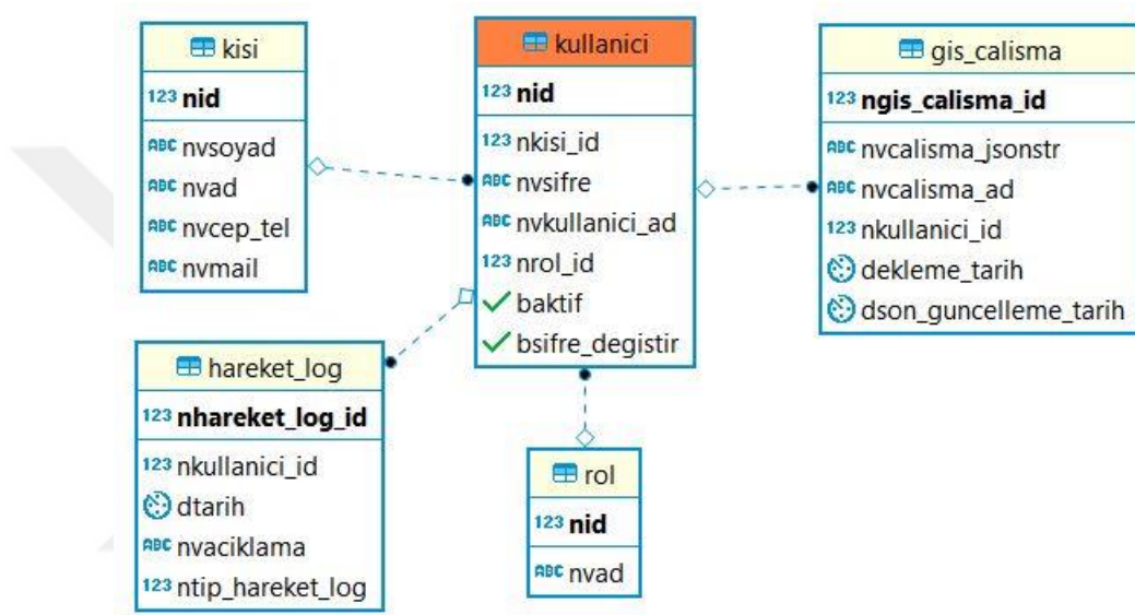
Şekil 3.7. Kullanıcı, kişi, yedek, çalışma, rol tabloları varlık ilişki diyagramı.
