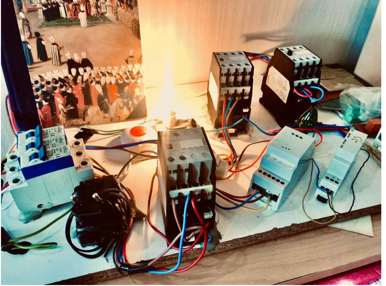
Pek çok unvanının yanında ayrıca mühendis olan Hasan Tahsin Feyizli'nin, üç fazlı motorların yanmasını önlediği, Tubitak tarafından patentini aldığı ve Avrupa ülkelerine gönderilen icadı.
