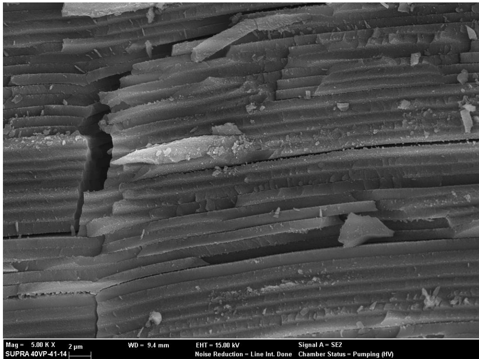
HC-17 yüksek büyütme SEM görüntüsü
