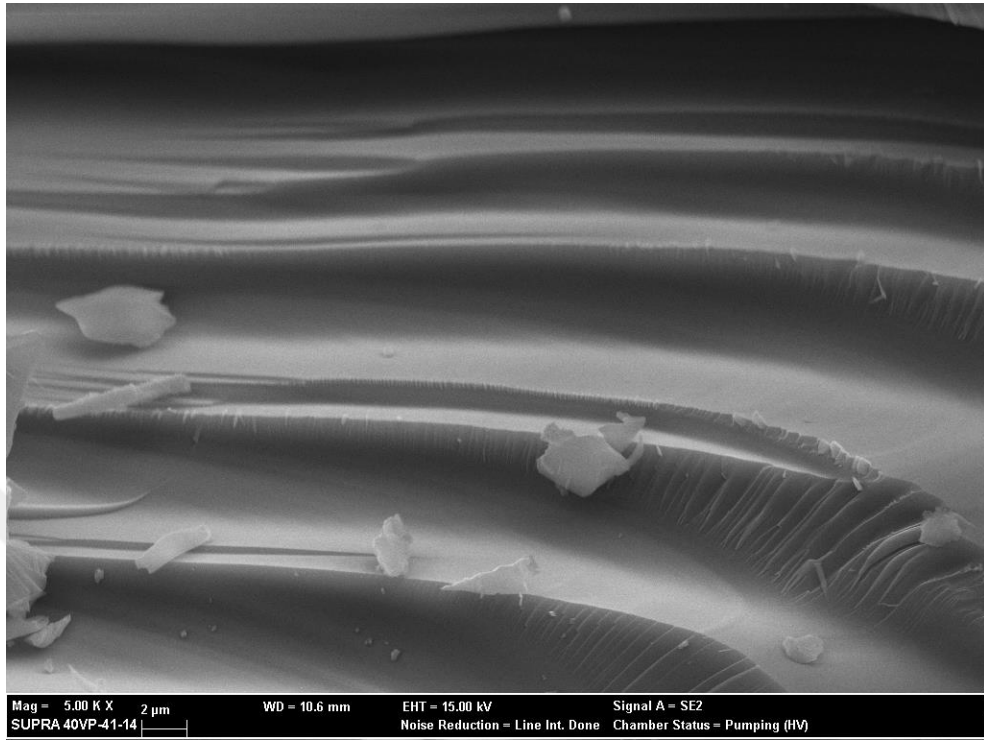
HC-12b yüksek büyütmeli SEM görüntüsü
