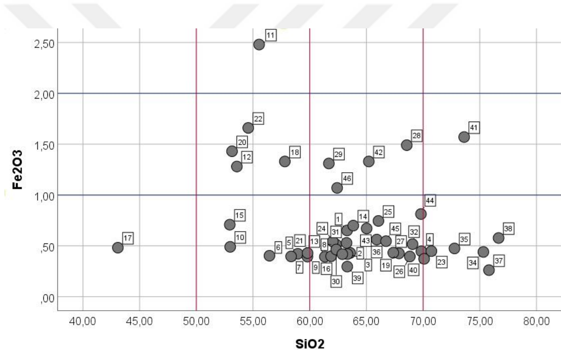
Şekil 6. 6. PED-XRF analiz sonuçlarına göre camlardaki Fe_2O_3 - SiO_2 içeriklerinin dağılım grafiği.
