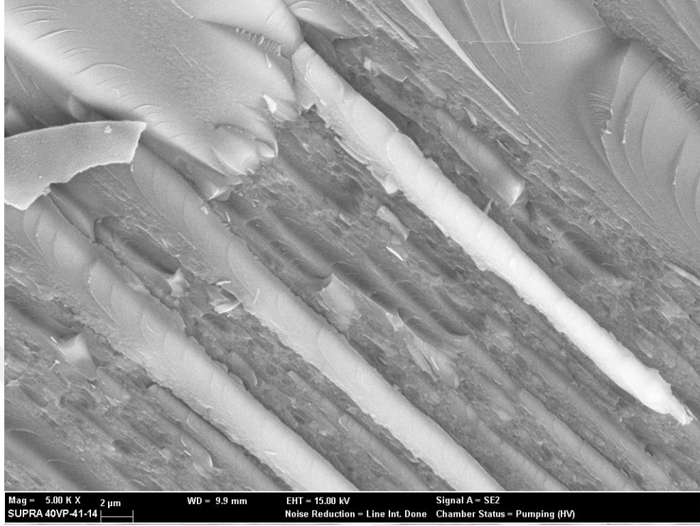
HC-2b yüksek büyötmeli SEM göröntüsü
