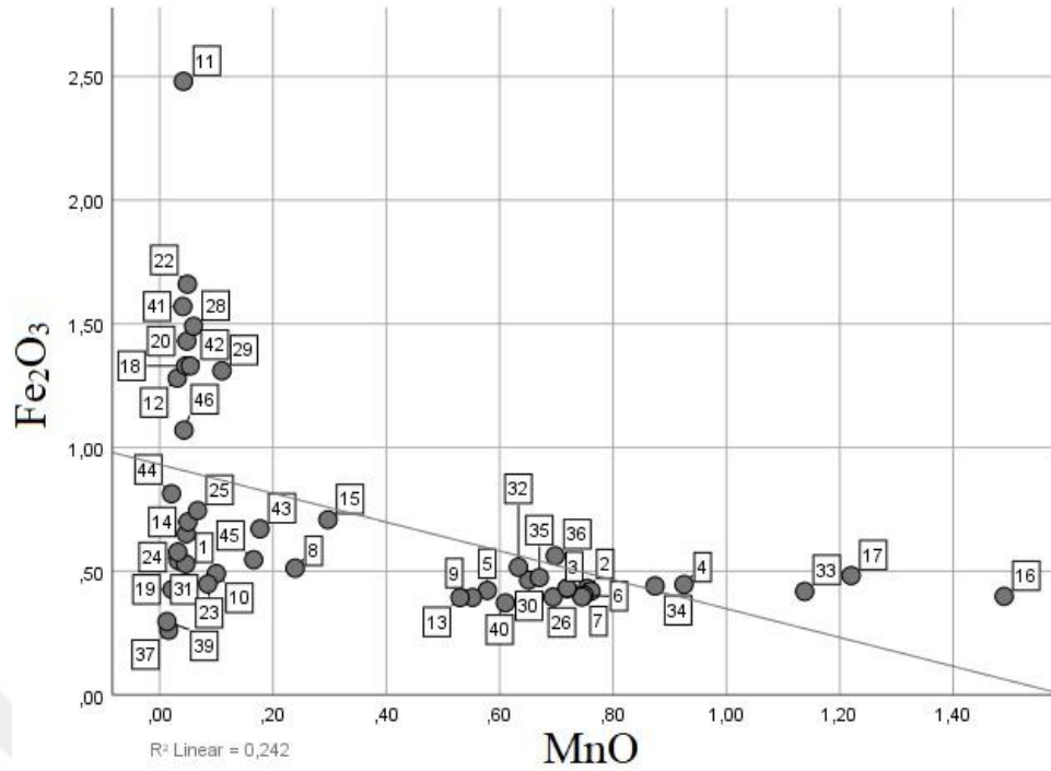
Şekil 6. 7. PED-XRF analiz sonuçlarına göre camlardaki \text{Fe}_2\text{O}_3 – MnO dağılım grafiği.
