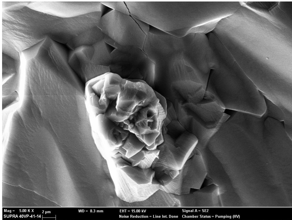
HC-20c yüksek büyütmeli SEM görüntüsü
