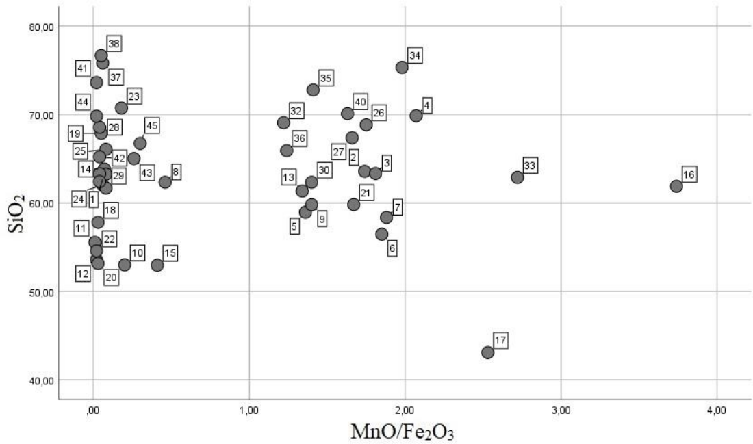
Şekil 6. 7. PED-XRF analiz sonuçlarına göre camlardaki \text{Fe}_2\text{O}_3 – MnO dağılım grafiği.
