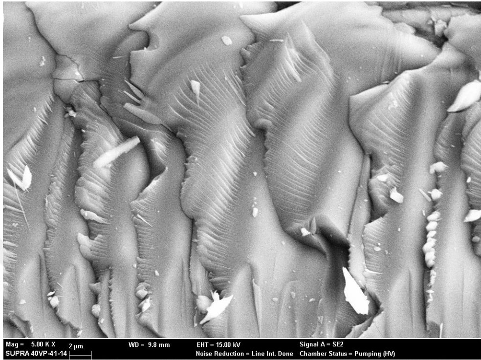
HC-16b yüksek büyütme SEM görüntüsü
