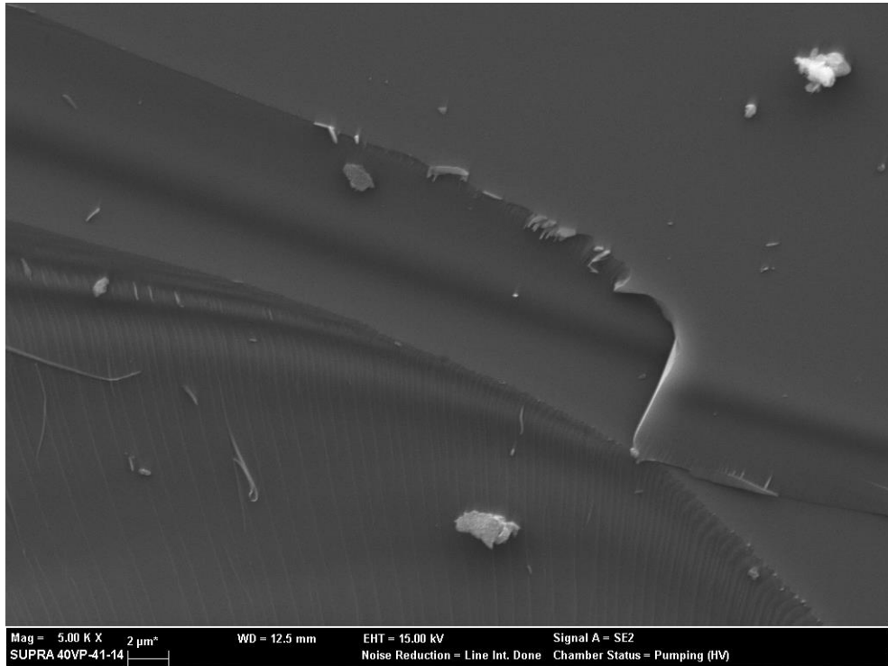
HC-13a yüksek büyütmeli SEM görüntüsü
