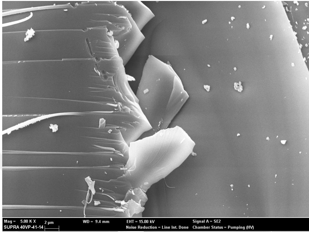
HC-21a yüksek büyütmeli SEM görüntüsü
