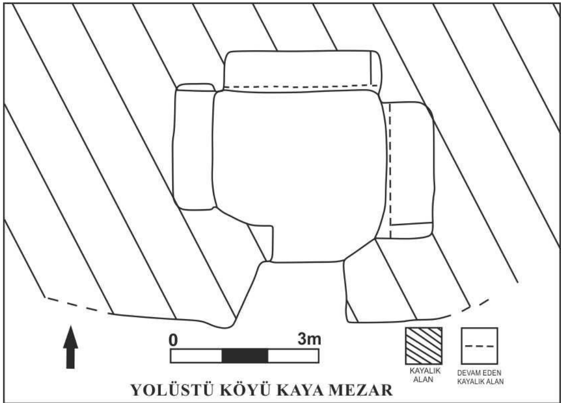
Çizim 3.11: Yolüstü Köyü Kaya Mezar Planı
