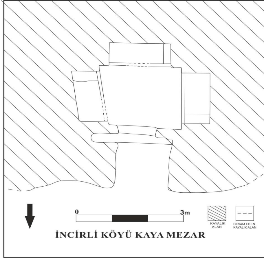
Çizim 3.9: İncirli Köyü Kaya Mezar Planı
