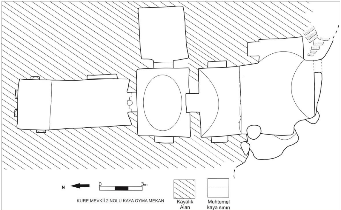
Çizim 5.5: Kure Mevkii 2 No'lu Kaya Oyma Mekân planı
