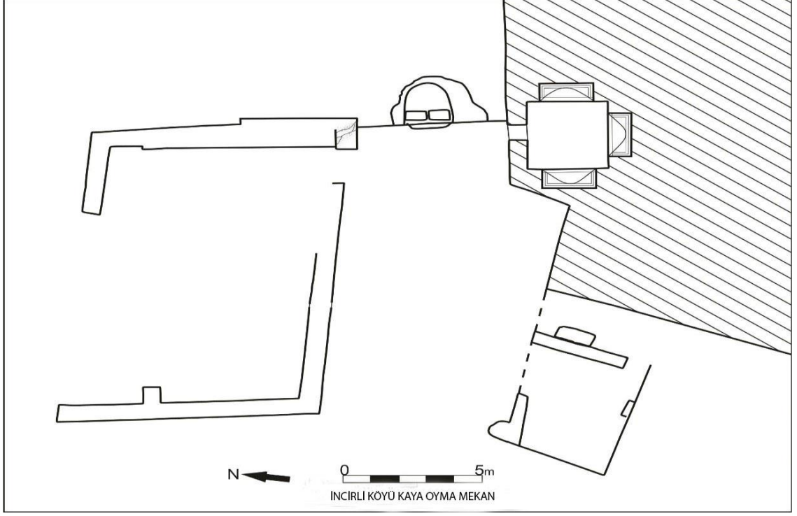
Çizim 3.3: İncirli Köyü Kaya Oyma Mekân planı
