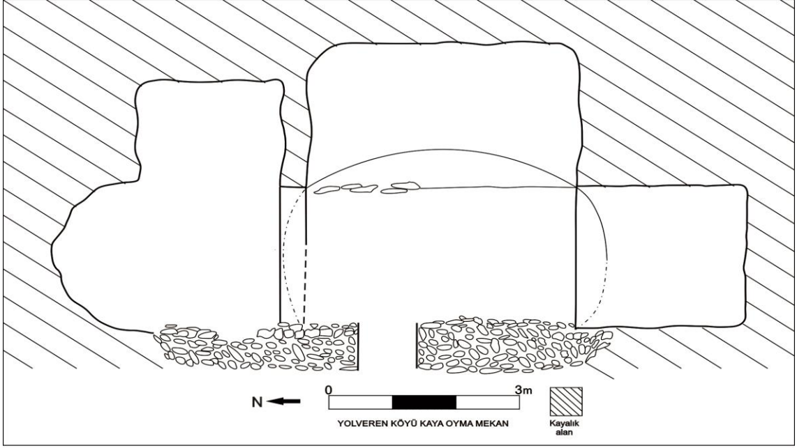
Çizim 3.7: Yolveren Köyü Kaya Oyma Mekân planı
