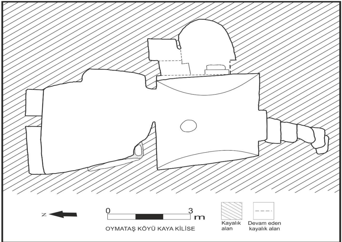
Çizim 3.12: Oymataş Köyü Kaya Kilisesi planı
