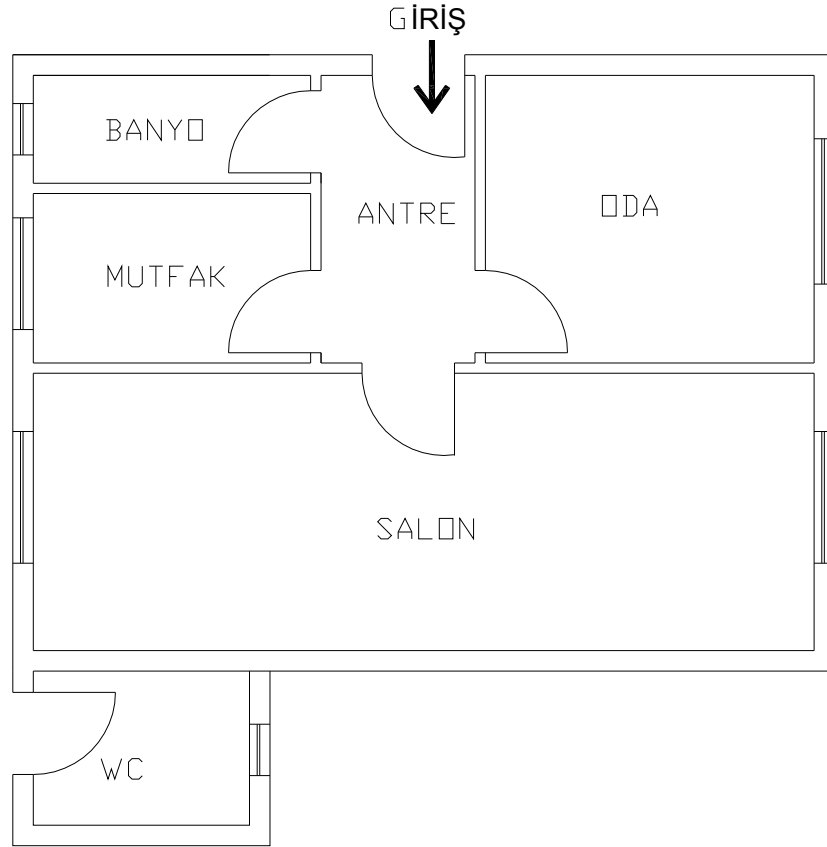
Şekil 19: Hasankeyf İlçe merkezinde 1967 yılında Devlet tarafından 245 adet yapılan afet evlerinden birinin konut planı
