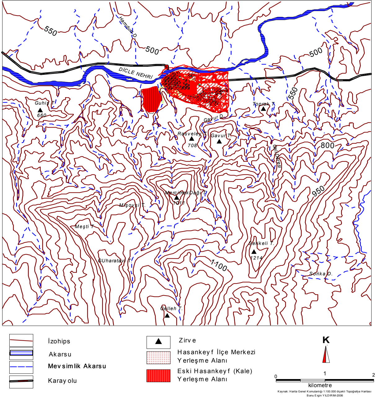
ŞEKİL :2 HASANKEYF VE YAKIN ÇEVRESİNİN TOPOĞRAFYA HARİTASI
