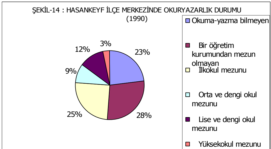
Şekil 14: Hasankeyf İlçe Merkezinde Okur Yazarlık Durumu(2000)
