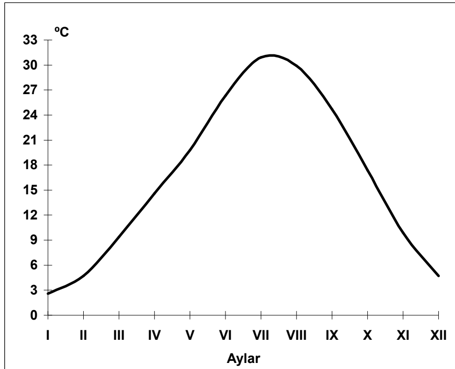
Şekil 4: Batman'da Aylık Ortalama Sıcaklık Grafiği
