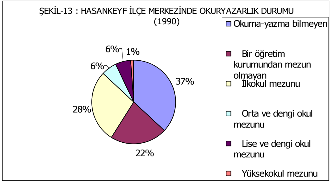
Şekil 13: Hasankeyf İlçe Merkezinde Okur Yazarlık Durumu(1990)
