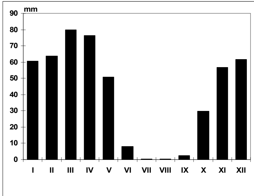
Şekil 5: Batman'ın Aylık Ortalama Yağış Grafiği (mm)
