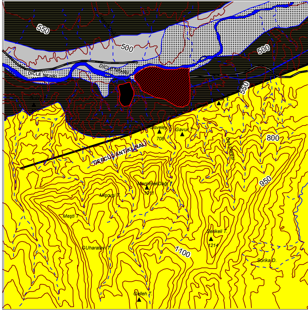
ŞEKİL : 3 HASANKEYF VE YAKIN ÇEVRESİNİN JEOLojİ HARİTASI
