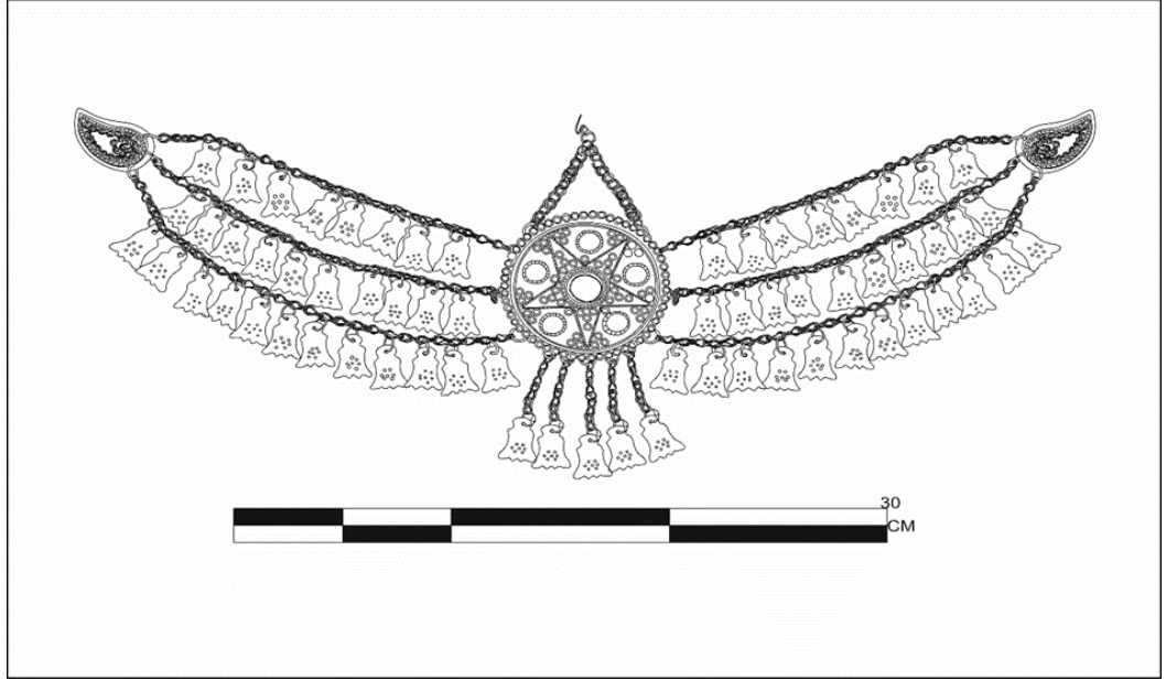
Çizim 5.7: Katalog 5.1.7'deki gerdanlığın çizimi
