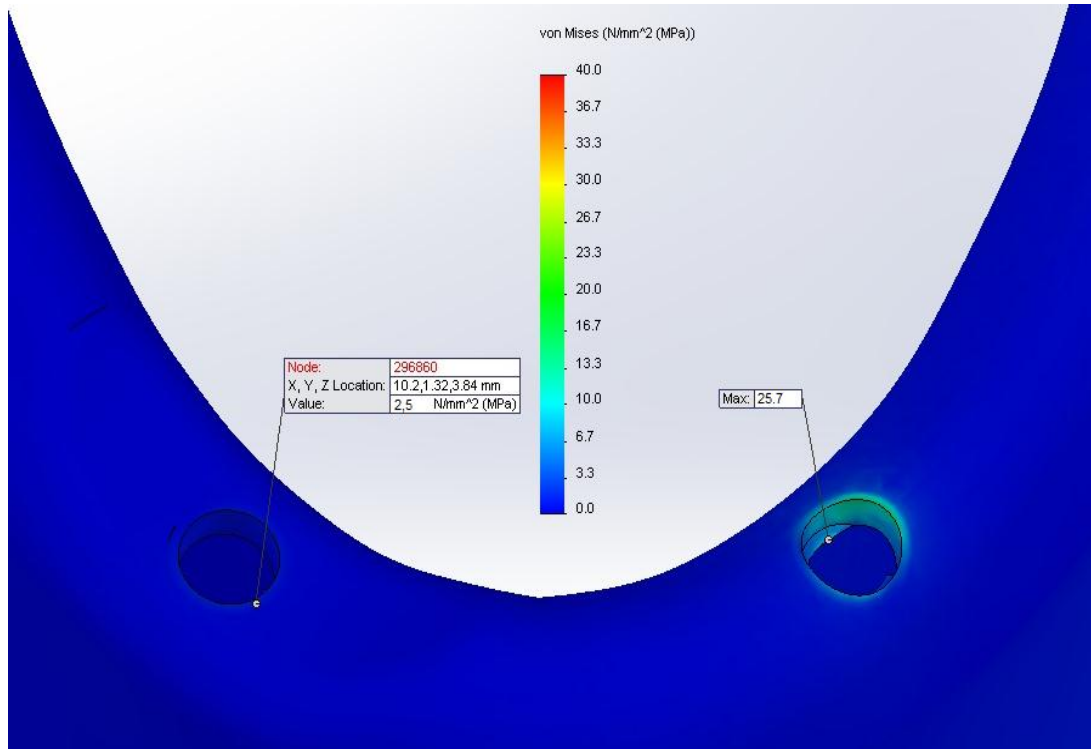
Şekil 55. Sol bölgeden uygulanan 150 N'luk yüklemenin 2,5 mm damak dolgu modelinde sert kemikte oluşturduğu von – Mises gerilme dağılımı
