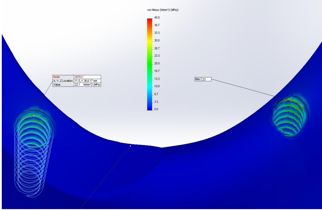
Şekil 91. Sağ ve sol bölgelerden uygulanan toplam 300 N'luk yüklemenin 4,5 mm damak dolgu modelinde yumuşak kemikte oluşturduğu von – Mises gerilme dağılımı
