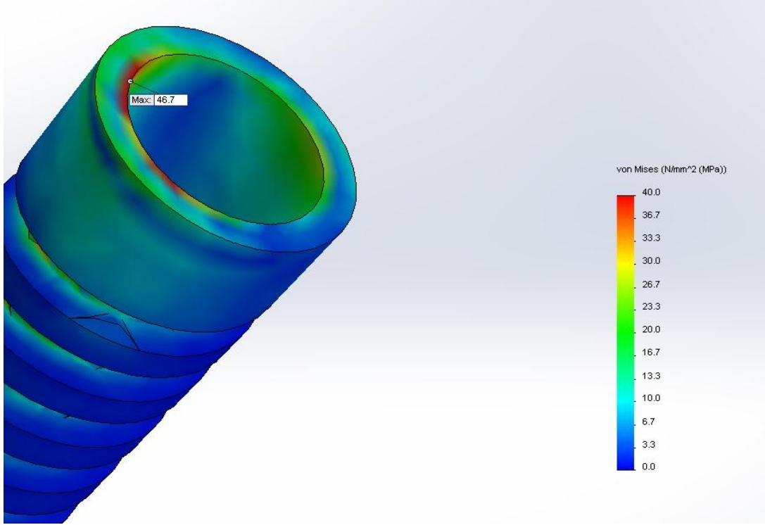
Şekil 70. Sol bölgeden uygulanan 150 N'luk yüklemenin 2,5 mm damak dolgu modelinde sol implanta oluşturduğu von – Mises gerilme dağılımı
