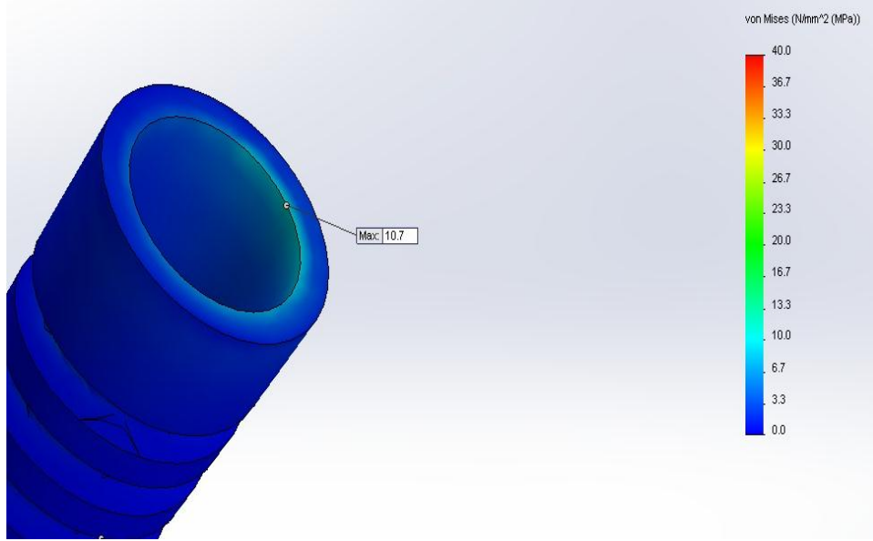
Şekil 40. Sağ bölgeden uygulanan 150 N'luk yüklemenin 2,5 mm damak dolgu modelinde sol implant üzerinde oluşturduğu von – Mises gerilme dağılımı
