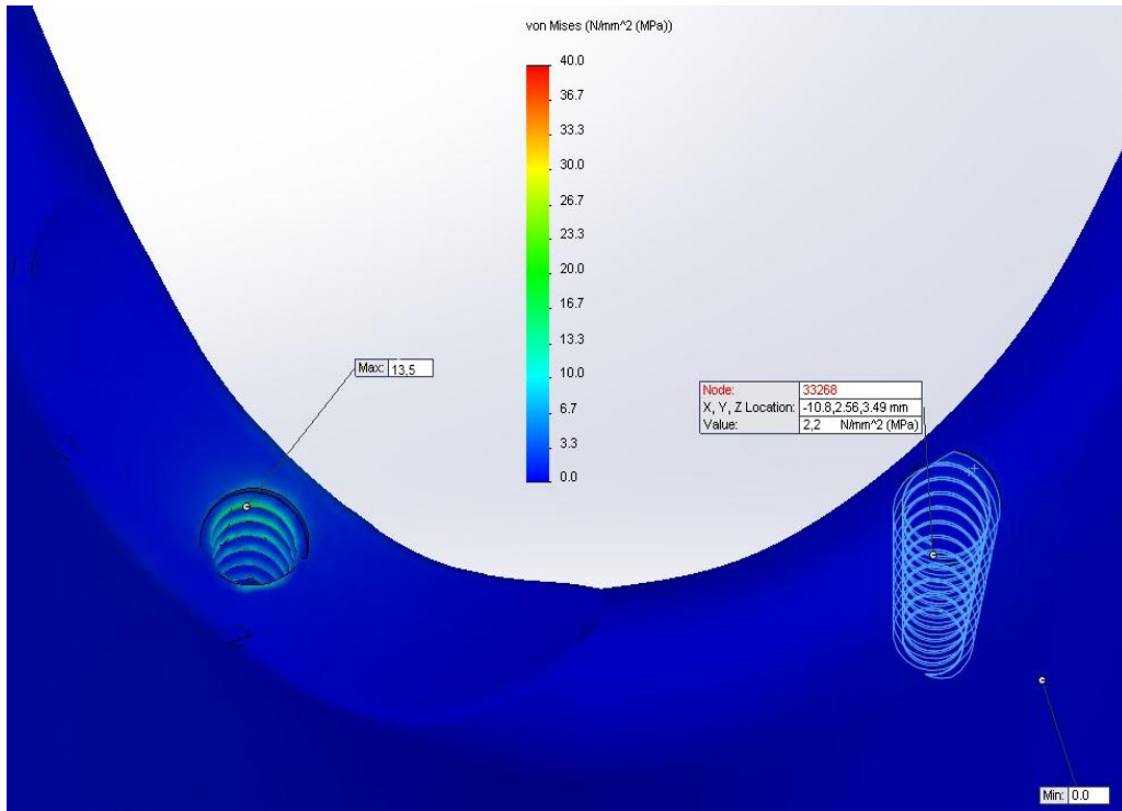
Şekil 31. Sağ bölgeden uygulanan 150 N'luk yüklemenin 2,5 mm abutment dolgu modelinde yumuşak kemikte oluşturduğu von – Mises gerilme dağılımı
