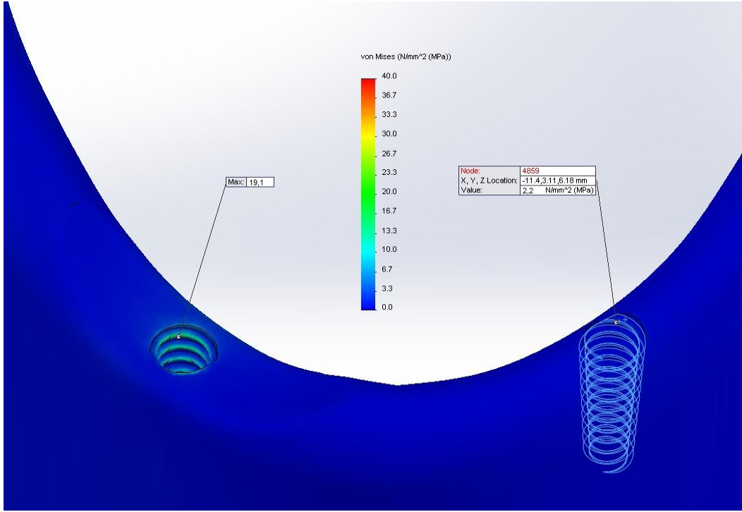
Şekil 32. Sağ bölgeden uygulanan 150 N'luk yüklemenin 2,5 mm damak dolgu modelinde yumuşak kemikte oluşturduğu von – Mises gerilme dağılımı
