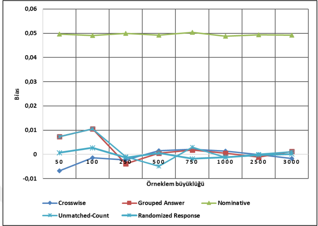
Şekil 4.83. Hassas soru yöntemlerine ait P=0,1 karşılaştırma grafiği
