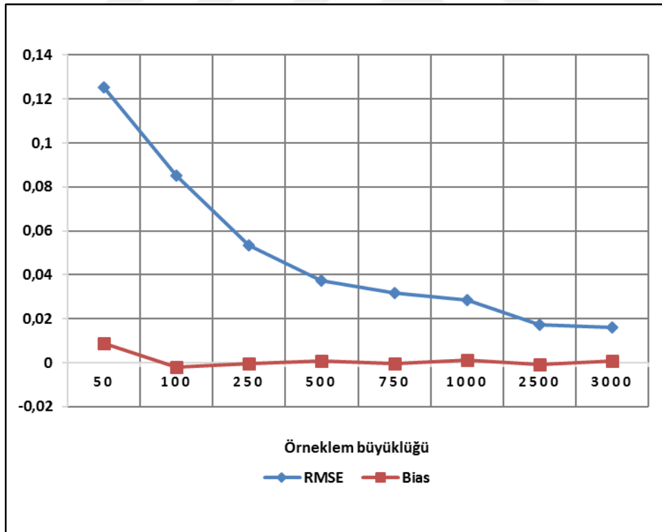
Şekil 4.54. Çapraz yöntemine ait P=0,005 grafiği
