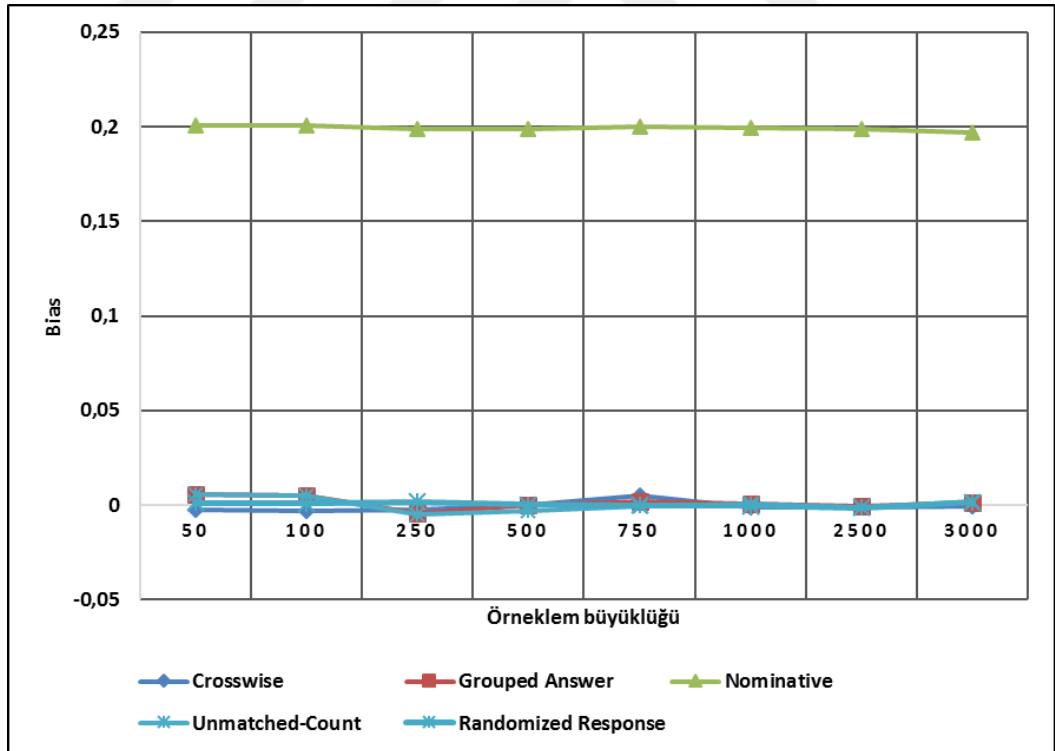
Şekil 4.86. Hassas soru yöntemlerine ait P=0,4 karşılaştırma grafiği
