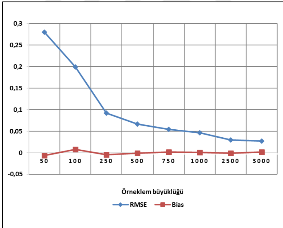
Şekil 4.48. Gruplandırılmış cevap yöntemine ait P=0,5 grafiği
