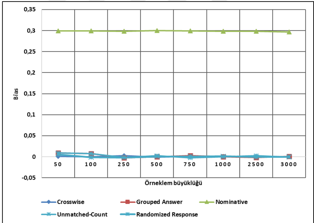
Şekil 4.88. Hassas soru yöntemlerine ait P=0,6 karşılaştırma grafiği
