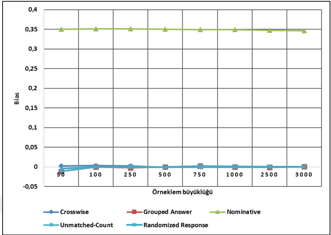
Şekil 4.89. Hassas soru yöntemlerine ait P=0,7 karşılaştırma grafiği
