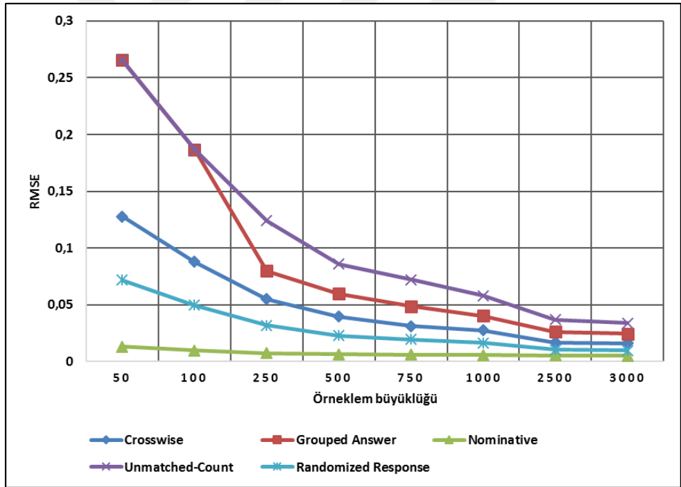
Şekil 4.68. Hassas soru yöntemlerine ait P=0,01 karşılaştırma grafiği
