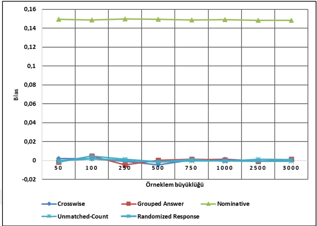
Şekil 4.85. Hassas soru yöntemlerine ait P=0,3 karşılaştırma grafiği
