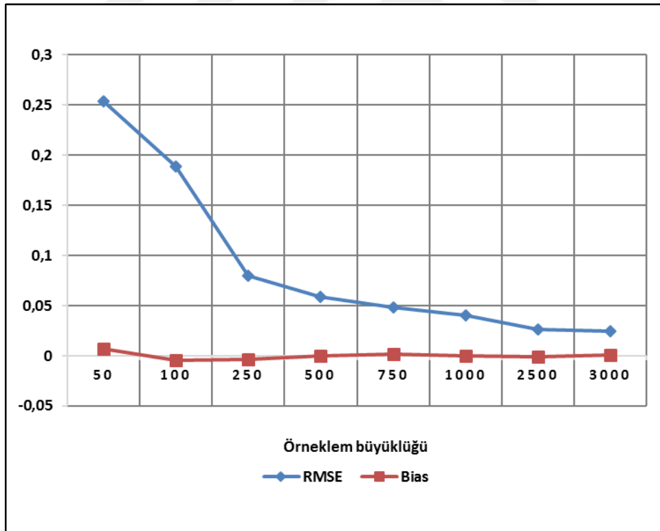
Şekil 4.40. Gruplandırılmış cevap yöntemine ait P=0,001 grafiği
