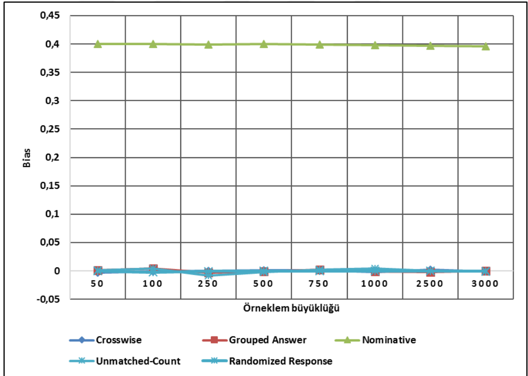
Şekil 4.90. Hassas soru yöntemlerine ait P=0,8 karşılaştırma grafiği
