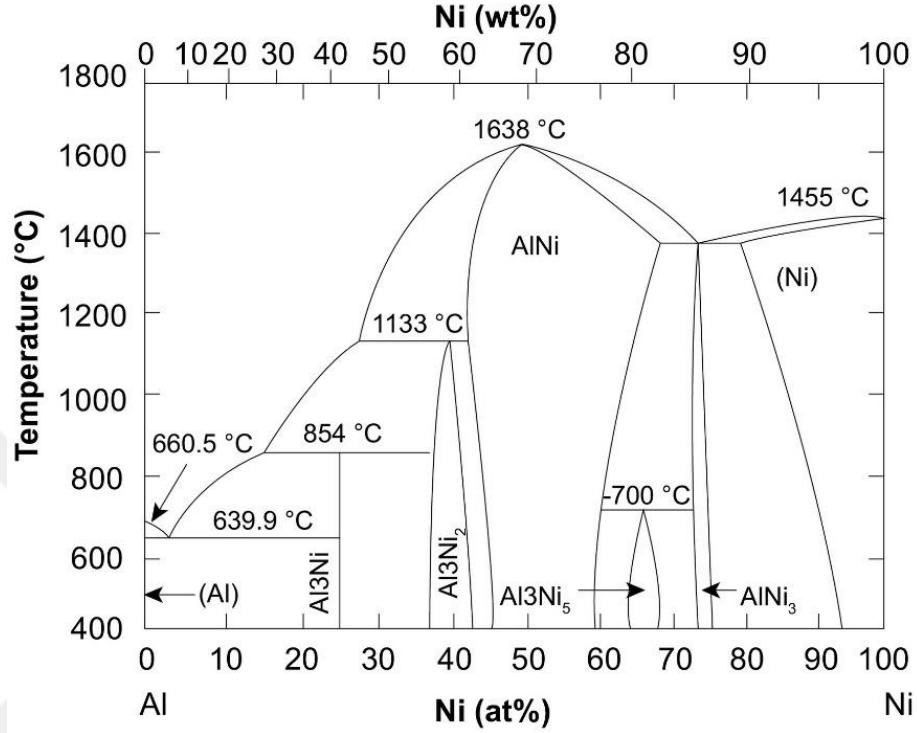
Şekil 2.12. Ni-Al denge diyagramı. [34,35]
