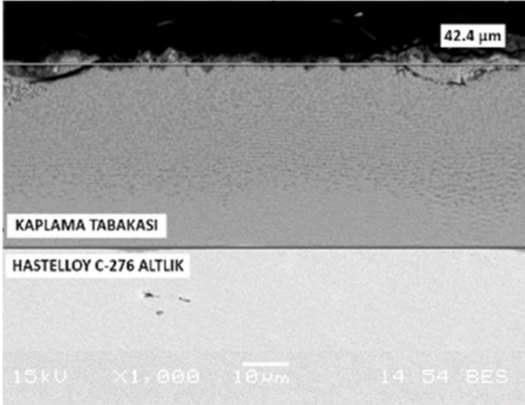
Şekil 5.28. 700°C’de 6 saat alüminyumlanan alaşımın SEM görüntüsü.
