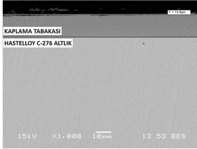
Şekil 5.12. 650°C’de 2 saat alüminyumlanan alaşımin SEM görüntüsü.
