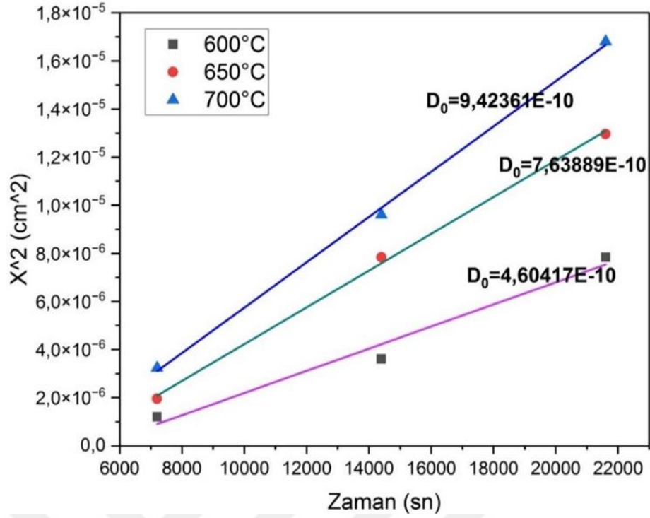
Şekil 5.40. Hastelloy C-276 alaşımasının (x 2 -t) diyagramı.
