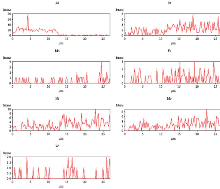
řekil 5.4. 600°C 2 saat alüminyumlanan Hastelloy C-276 alařımının çizgi analizi.
