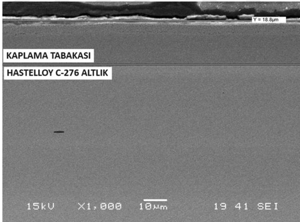
Şekil 5.21. 700°C’de 2 saat alüminyumlanan alaşımın SEM görüntüsü.
