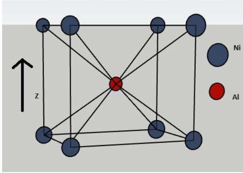
Şekil 2.11. NiAl (B2) kristal yapısı. [55]
