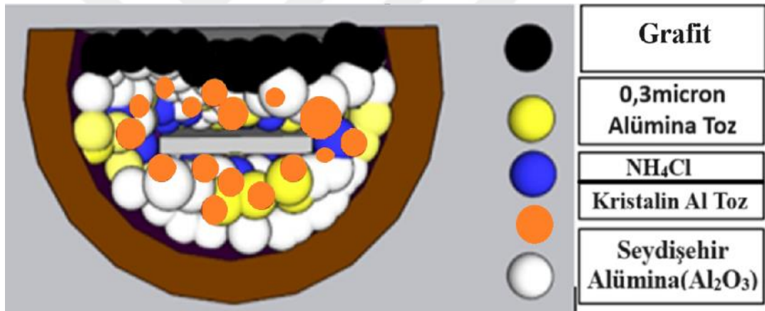
Şekil 4.7. Kutu karışımı ve numunenin kutu içerisindeki yerleşimi.
