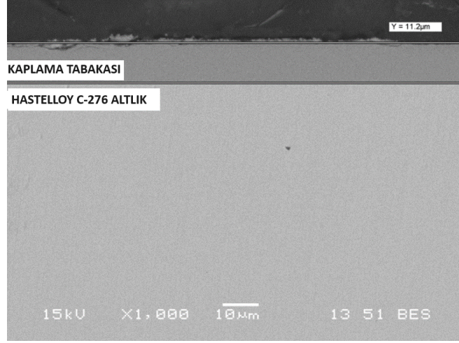
Şekil 5.2. 600°C 2 saat alüminyumlanan alaşımanın SEM görüntüsü.
