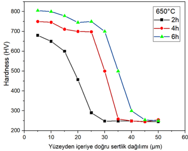
Şekil 5.37. 650°C’ de farklı sürelerde alüminyumlanan Hastelloy C-276 alaşımlarının yüzeyden itibaren mesafeyle sertlik değişimi.
