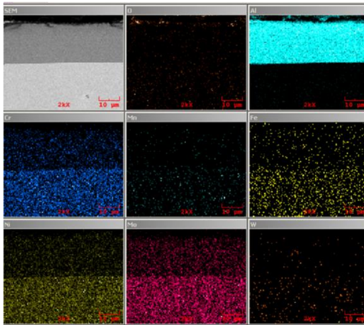
Şekil 5.8. 600°C 4 saat alüminyumlanan Hastelloy C-276 alaşımının MAP analizi.
