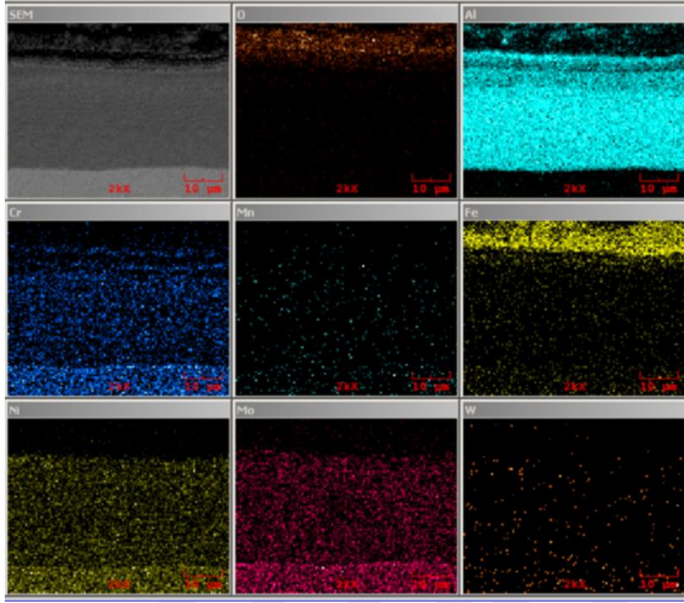
Şekil 5.27. 700°C 4 saat alüminyumlanan Hastelloy C-276 alaşımının MAP analizi.
