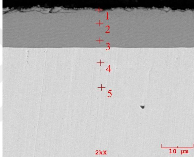
Şekil 5.2. 600°C 2 saat alüminyumlanan alaşımanın SEM görüntüsü.
