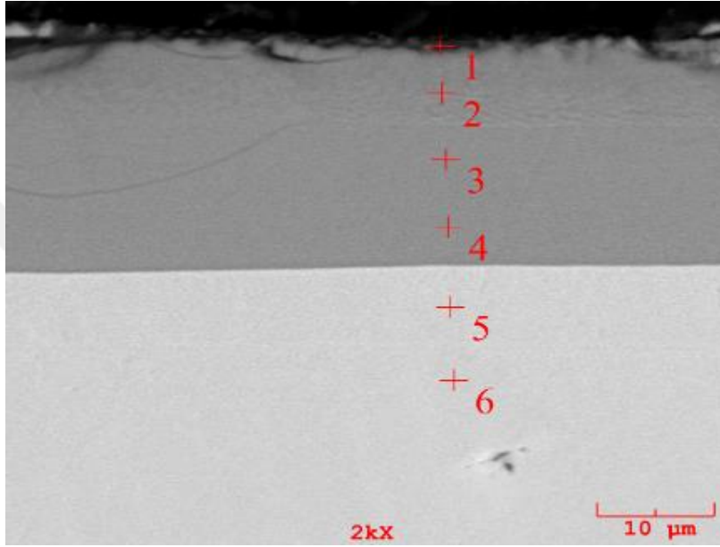
Şekil 5.7. Al kaplı Hastelloy C-276'nın 600° C'de 4 saatlik SEM-EDS analizi.
