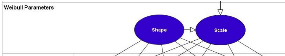
Figure 32 Weibull Parameter Nodes
