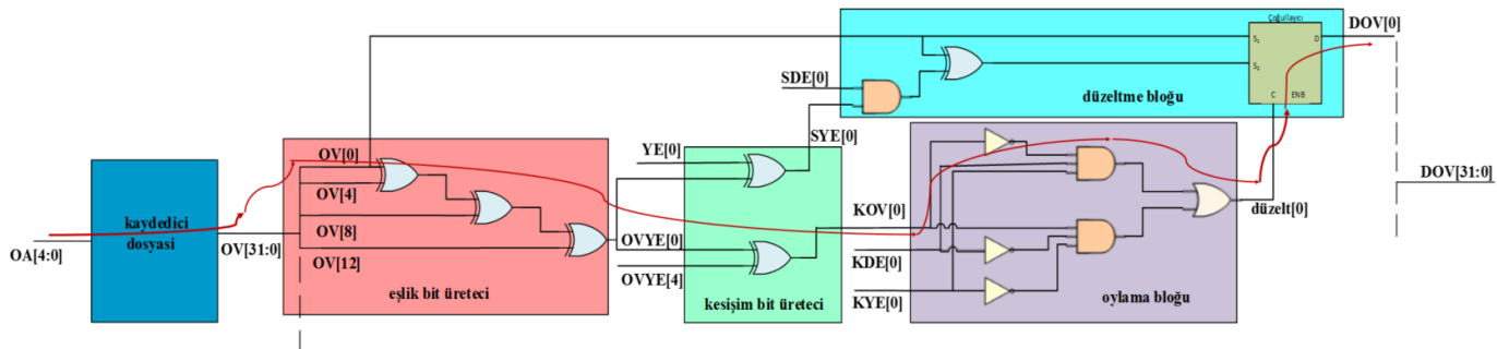
Şekil 6.6: KodSeti yöntemi için kritik yol.
