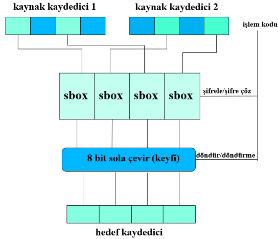
Şekil 5.8: sbbox4s, isbox4s ve sbox4r komutlarının işlevi.
