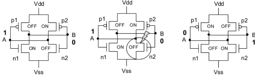
Şekil 2.3: SRAM bellek hücresine partikül çarpması.
