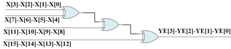
Şekil 6.9: KodSeti-4 için gereken XOR zinciri.
