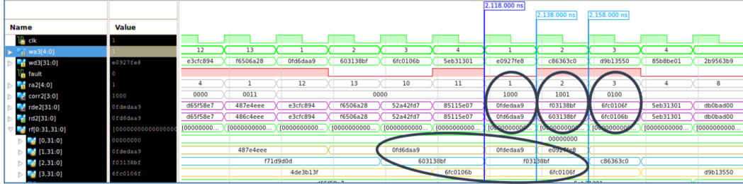
Şekil 6.1: Kaydedicilere gelen geçici hataların düzeltilme işlevi.
