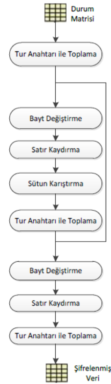
Şekil 5.7: AES algoritmasının blok yapısı.
