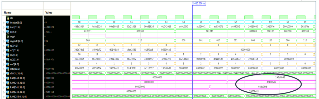
Şekil 5.13: Şifrelenmiş mesajın simülasyon sonucu.
