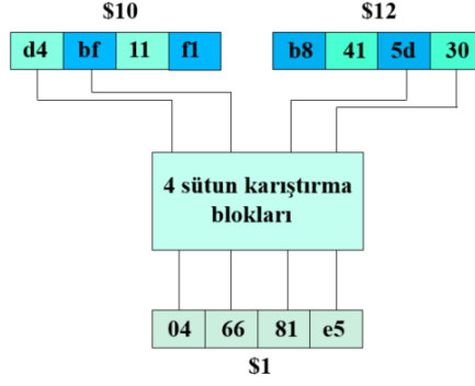
Şekil 5.11: mixcol4s komut işlev örneği
