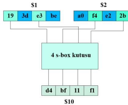
Şekil 5.10: sbox4s komut işlev örneği.
