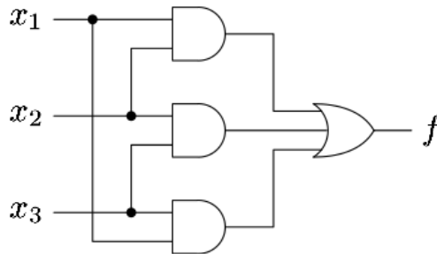
Şekil 4.3: Oylama devresi.
