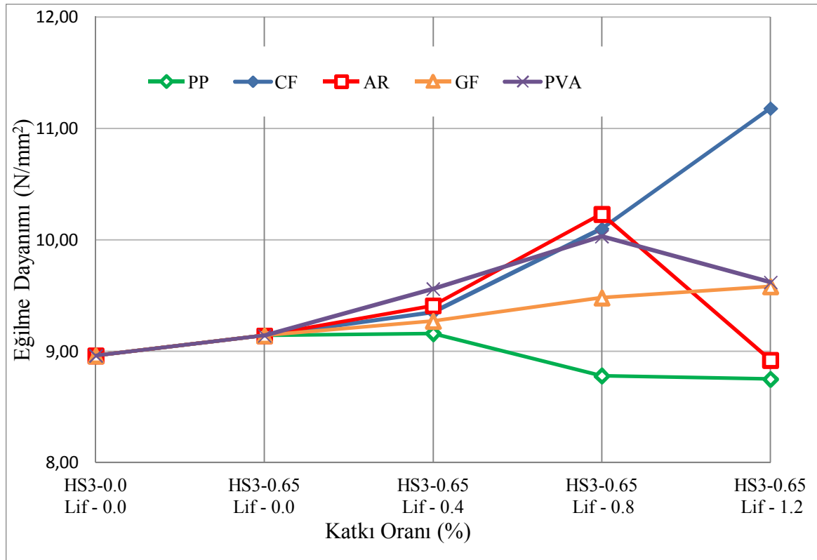
Şekil 3.19. Lif katkılı harçların eğilme dayanımı
