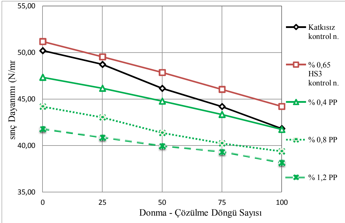
Şekil 3.22. Donma-çözölme etkisindeki numunelerde PP lifi oranı ile basınç dayanımı arasındaki ilişki
