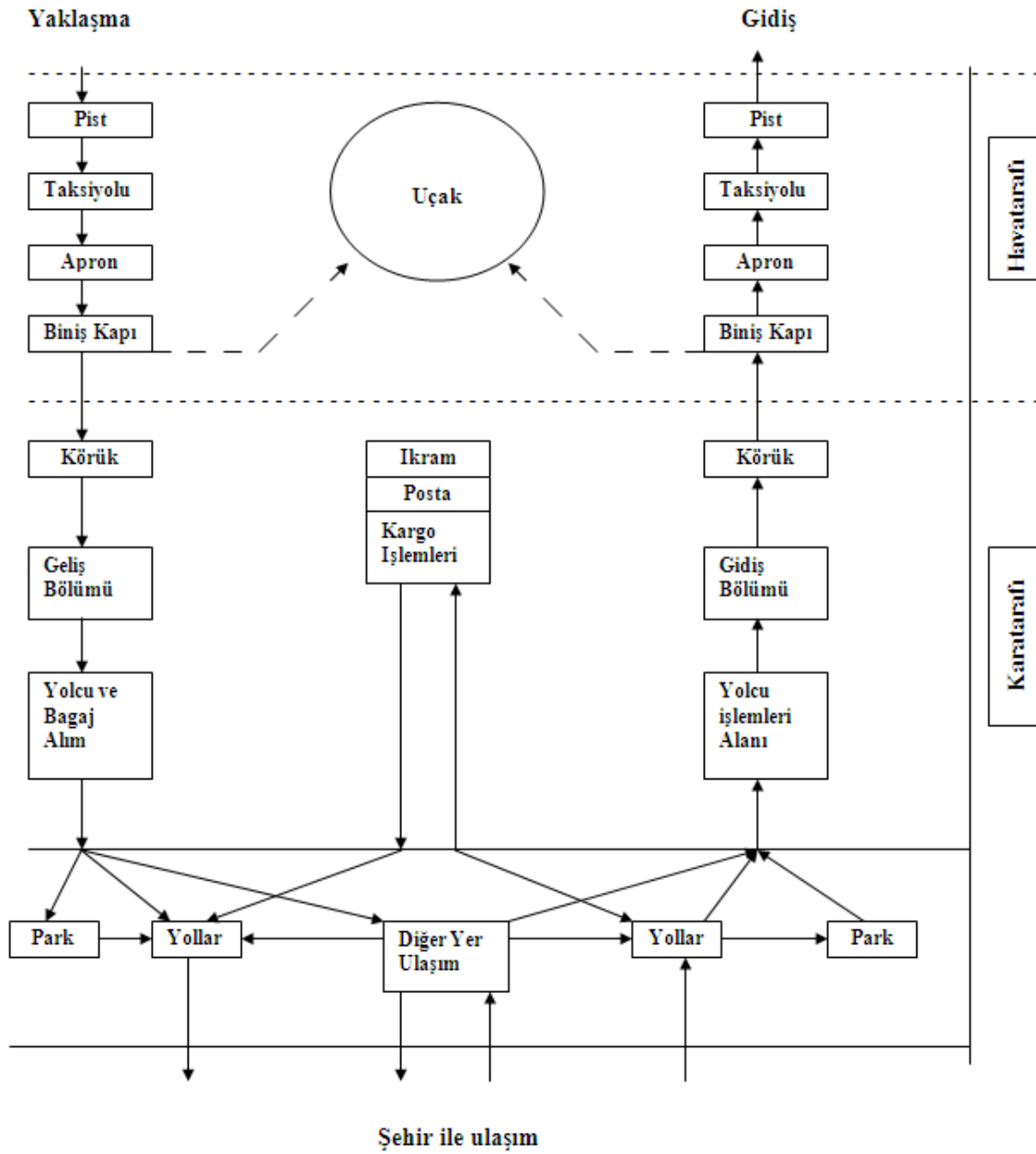
Şekil 2. Havaalanı Sistemi
