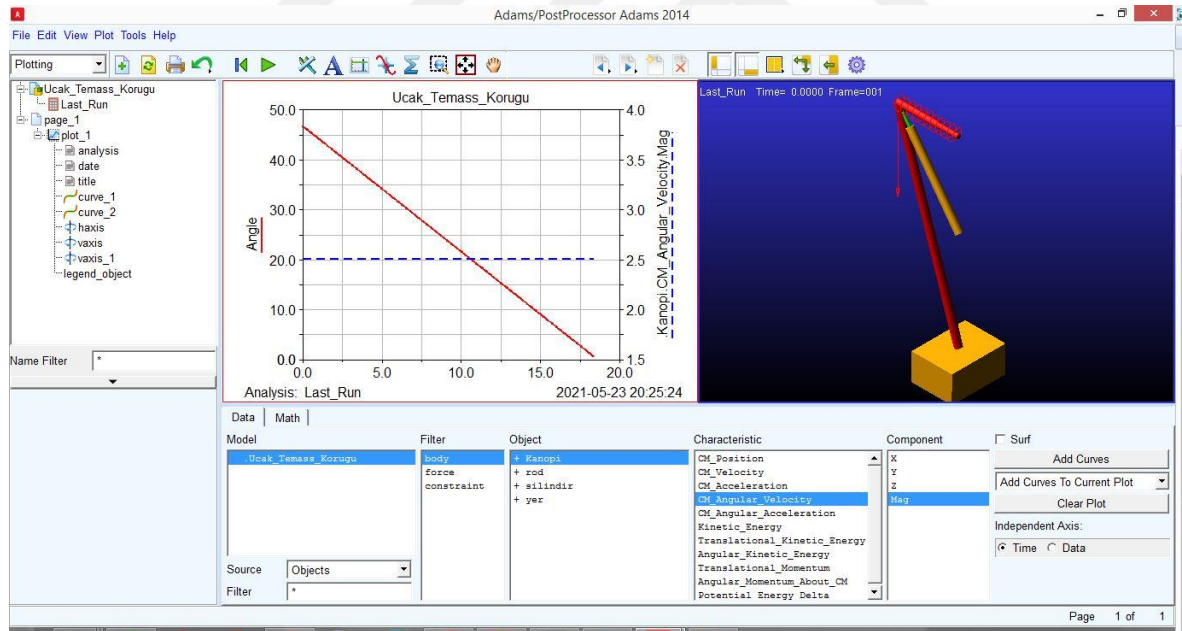
Şekil 3.6. Açı ve açısal hızın aynı grafik üzerinde değişimi
