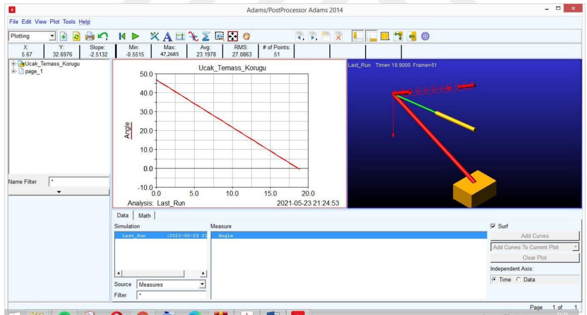
Şekil 3.2. Uçak Temass Körüğü açısız değişim
