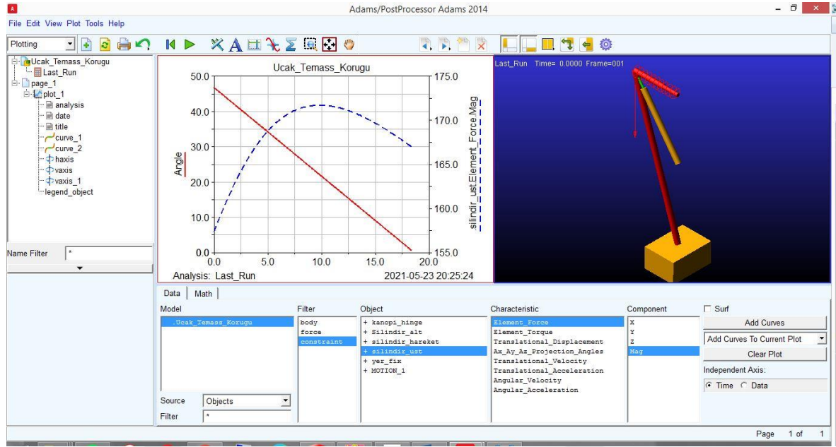
Şekil 3.7. Açısal değişimi ve silindire binen yük karşılaştırılması
