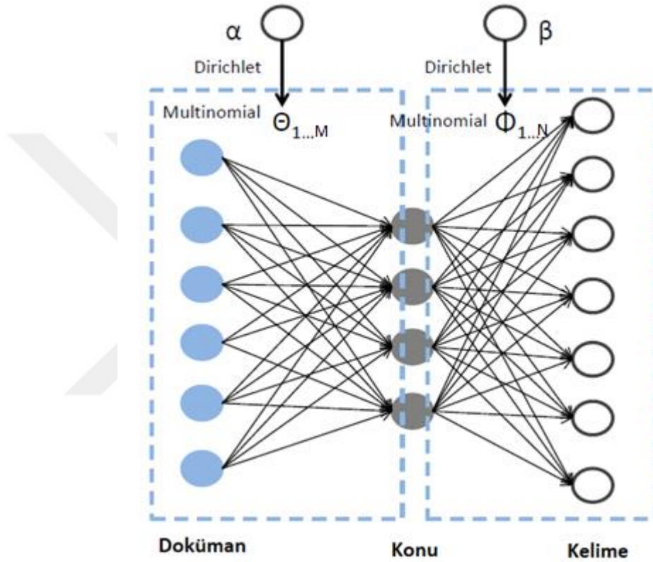
Şekil 3.5. GDA algoritması doküman-konu, konu-kelime eşleştirmesi (Zhao, 2015)
