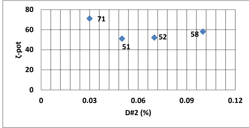
Şekil 6.82. Farklı miktarlarda D#2 ilavesiyle ζ-potansiyelindeki değişim
