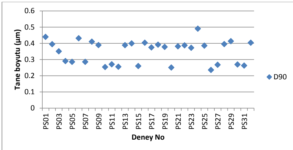
Şekil 6.30. Planetary değirmen su sistemi tane boyut analiz sonuçları a) D10, b) D50, c) D90
