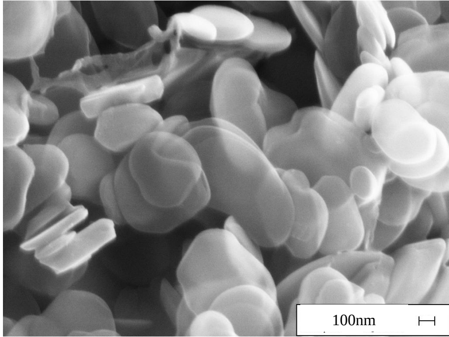
Şekil 6.58. A36-I numunesine ait ikincil elektron SEM görüntüleri
