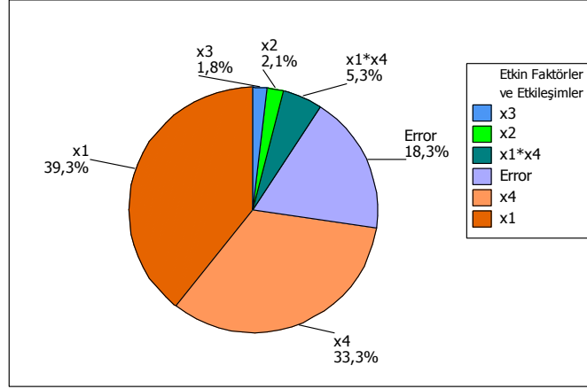
Şekil 6.22. Atritor değirmen deney tasarımında faktörler, etkileşimler ve hataların ortalama D90 yanıtına olan etkilerinin yüzdesel dağılımı
