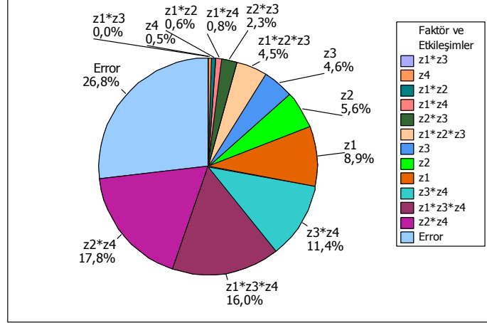
Şekil 6.32. Planatery değirmen deney tasarımında faktörler, etkileşimler ve hataların ortalama D90 yanıtına olan etkilerinin yüzdesel dağılımı
