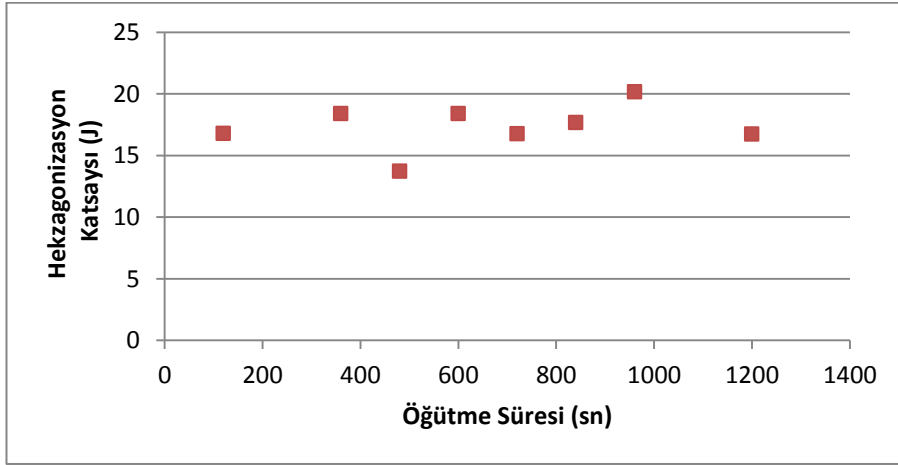
Şekil 6.72. Planetary değirmen kuru öğütme sisteminde öğütme süresine bağlı olarak tBN yapısında kristalinitedeki değişim
