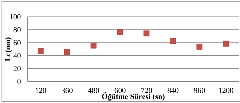
Şekil 6. 74. Planatery değirmne kuru öğütme sisteminde öğütme süresine bağlı olarak hBN numunelerinin Lc değerlerindeki değişim
