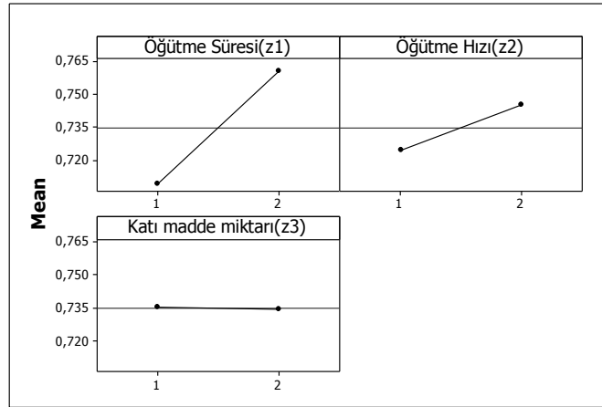
Şekil 6.18. Bilyalı değirmen yaşı öğütme izopropil alkol ortamı için ana etki grafiği
