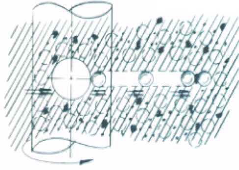
Şekil 4.10. Atritör değirmen öğütme prensibi
