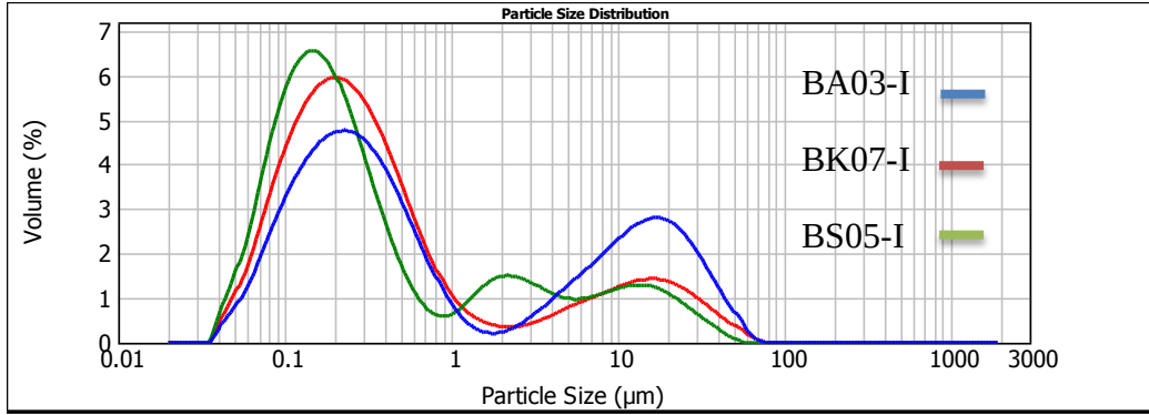
Şekil 6.48. Bilyalı değirmen bazı numunelere ait tane boyut dağılım grafikleri
