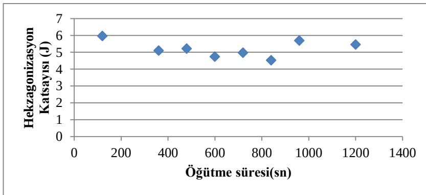
Şekil 6. 75. Planatery değirmne kuru öğütme sisteminde öğütme süresine bağlı olarak hBN yapısında kristalinitedeki değişim
