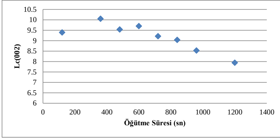
Şekil 6.71. Planetary değirmene kuru öğütme sisteminde öğütme süresine bağlı olarak tBN yapıda Lc ‘deki değişim
