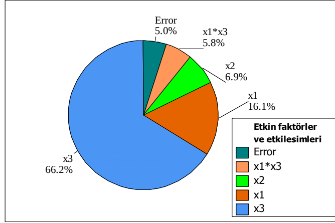
Şekil 6.27. Planetary değirmen kuru öğütme sisteminde faktör ve etkileşimlerin dağılımları
