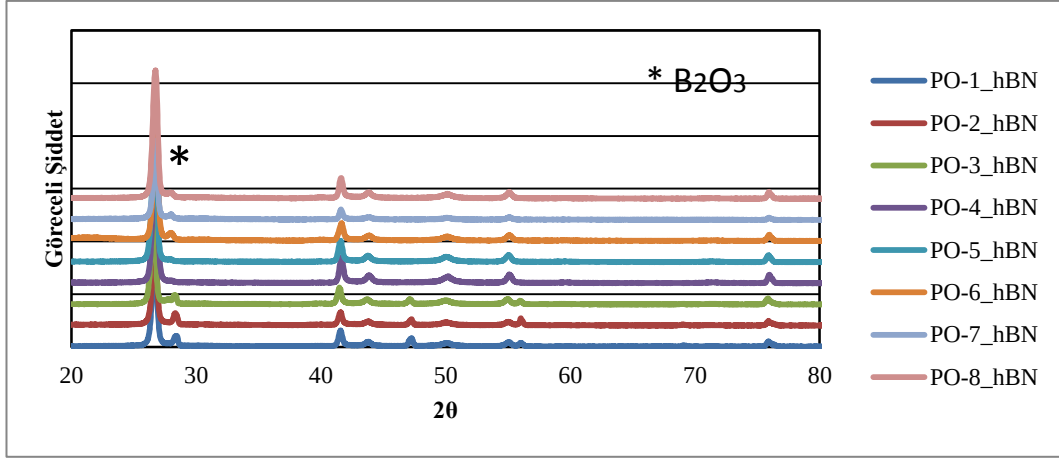
Şekil 6.73. Planatery değirmende kuru öğütme sisteminde farklı öğütme sürelerinde öğütülmüş numunelere ait x ışınları paterni
