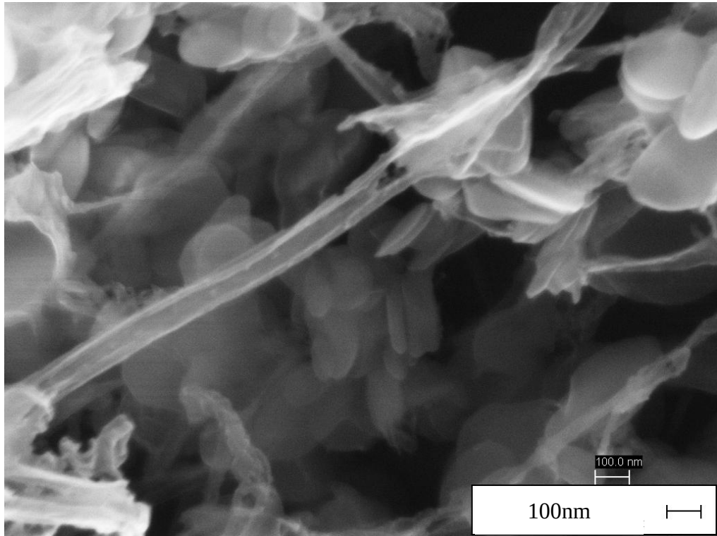
Şekil 6.62. A52-I numunesine ait SEM görüntüsü a) BNNT ler, 15000x b) BNNT 180000x
