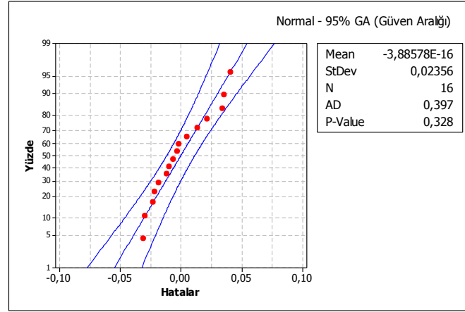
Şekil 6.11. Bilyalı değirmen kuru öğütme sistemi hataların normal dağılım eğrisi (Normalite testi)
