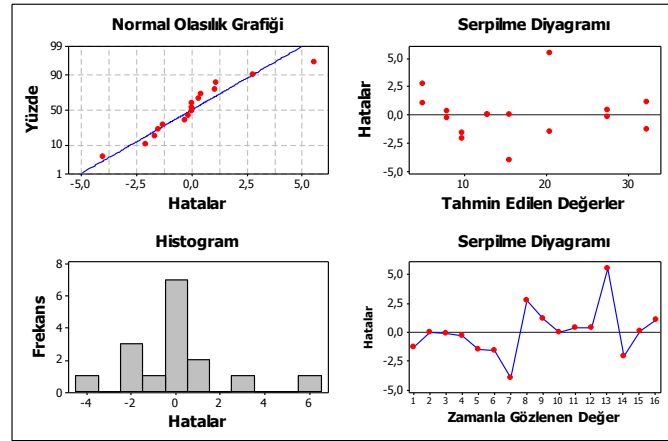
Şekil 6.28. Planetary değirmen kuru öğütme sistemi için hata analizi (yeterlik testi)
