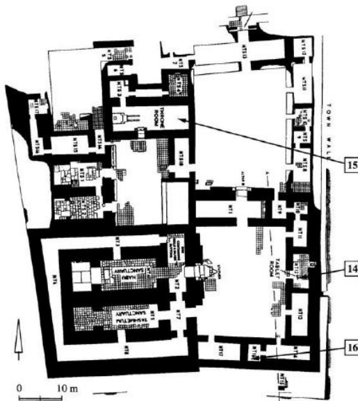
Şekil 2.8: Nimrud Nabu Tapınağı Arşiv ve Kütüphaneleri
