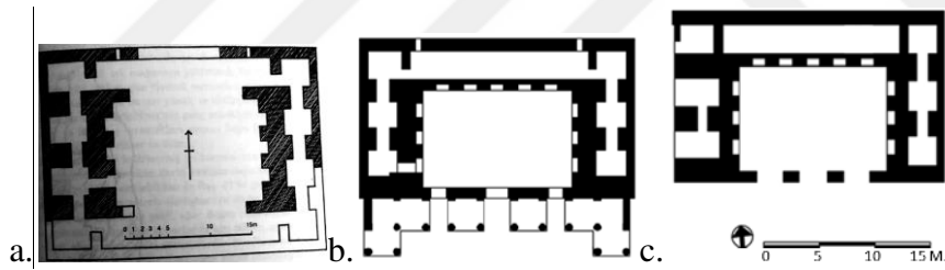
Şekil 3.44: Nysa Gymnasium Kütüphanesi Plan Önerileri, a. Diest'in Planı b. Hoephner'in Planı, c. İdil'in Planı
