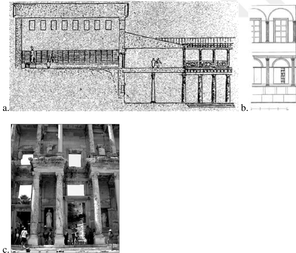
Resim 4.4: Kütüphane Yapılarında Pencereler, a. Pergamon Kütüphanesi Plan Kesiti Pencere Görünümü Rekonstrüksiyonu, b. Pergamon Asklepios Kütüphanesi Pencere ve Nişleri Gösteren Rekonstrüksiyon, c. Ephesos Celsus Kütüphanesi Pencere Açıklıkları
