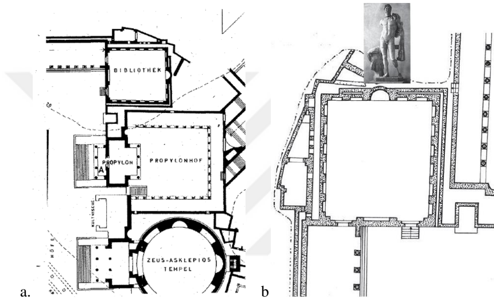
Şekil 3.49: Pergamon Asklepion Kütüphanesi Planı ve Plan Kesiti
