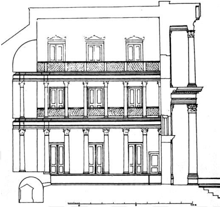
Şekil 3.25: Ephesos Celsus Kütüphanesi'nde Mezar Yerini Gösteren Bir Kesit Çizimi
