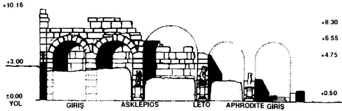
Şekil 3.34: Kremna Kütüphanesi'nin Yapı Kesiti
