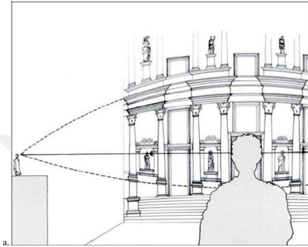
Şekil 3.27: Ephesos Celsus Kütüphanesi, a. Hueber'in Kütüphane Cephesi İllüzyonunu Gösteren Kroki, b. Burrell'in Kütüphane ve Çevresini Gösteren Çizimi
