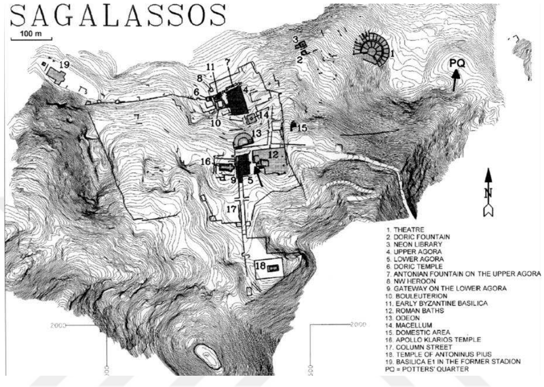
Şekil 3.35: Sagalassos Kent Planı
