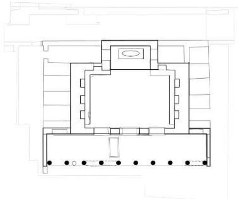
Şekil 3.45: Nysa Gymnasium Kütüphanesi Gerçek Plan Şekli Önerisi
