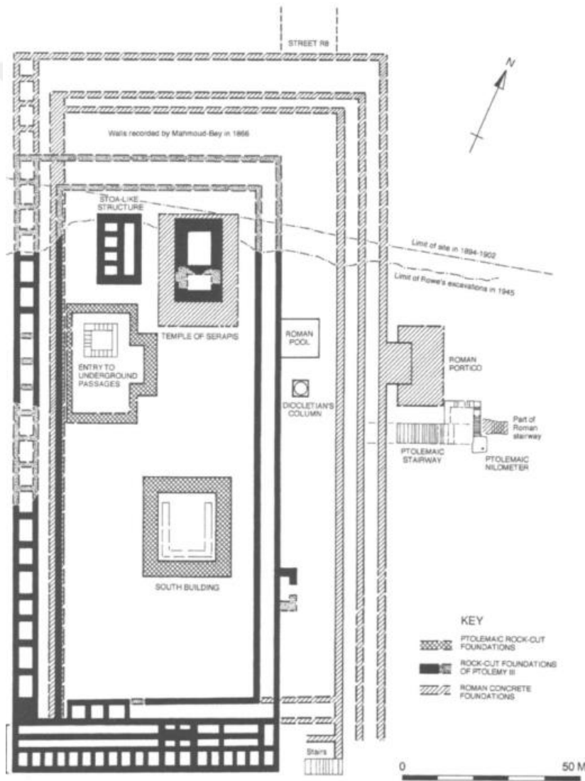
Şekil 3.3: İskenderiye Serapis Tapınağı Planı
