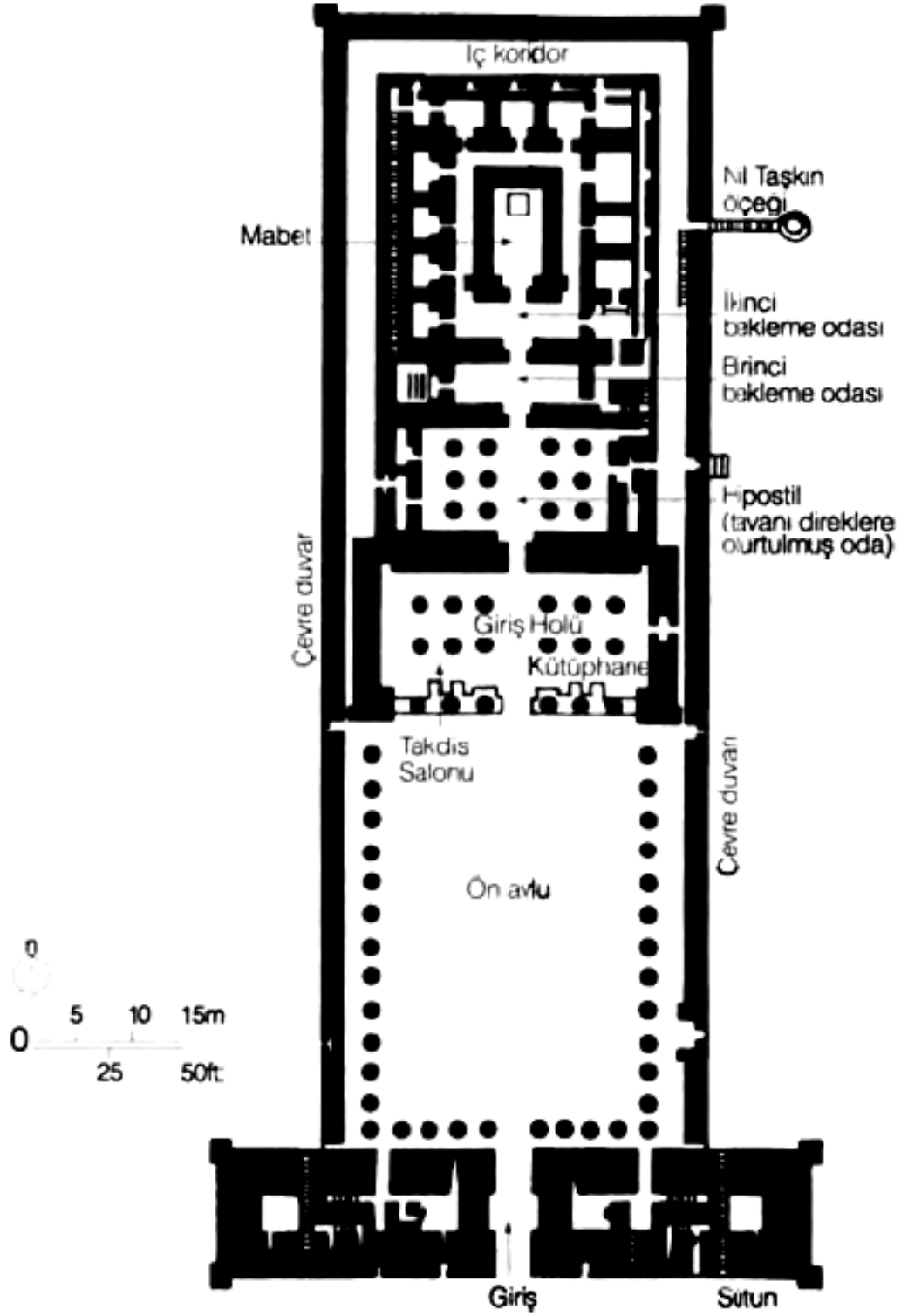
Şekil 2.14: Edfu Horus Tapınağı Planı (MÖ 237-212)
