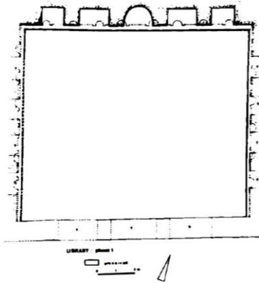
Şekil 3.37: Sagalassos Neon Kütüphanesi'nin 1. Evre Planı (MS 120 Sonrası)
