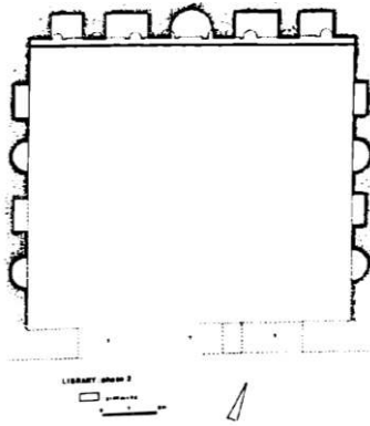
Şekil 3.38: Sagalassos Neon Kütüphanesi'nin 2. Evre Planı (MS 2. yy. Sonu)
