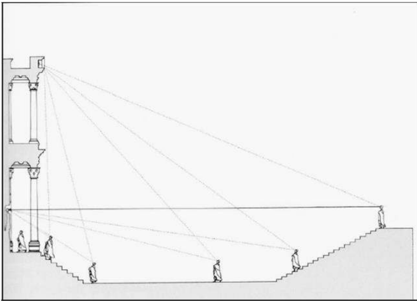
Şekil 3.26: Ephesos Celsus Kütüphanesi Gözlemcinin Görsel Konisini Gösteren Taslak
