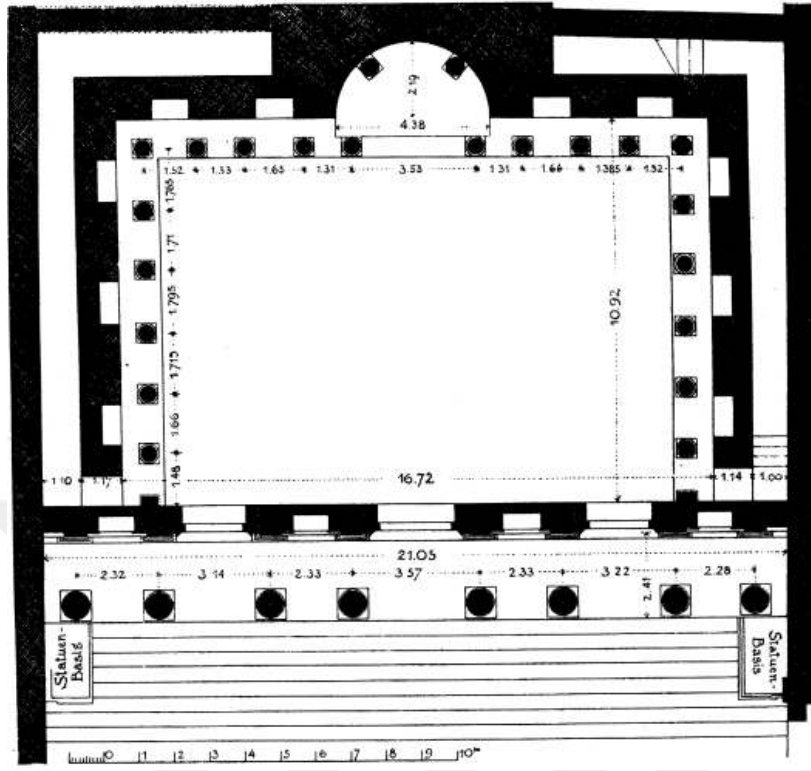
Şekil 3.21: Ephesos Celsus Kütüphanesi Planı
