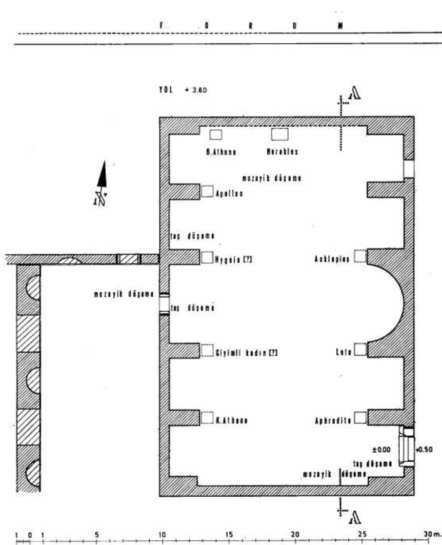
Şekil 3.32: Kremna Kütüphanesi (Q Yapısı) Planı
