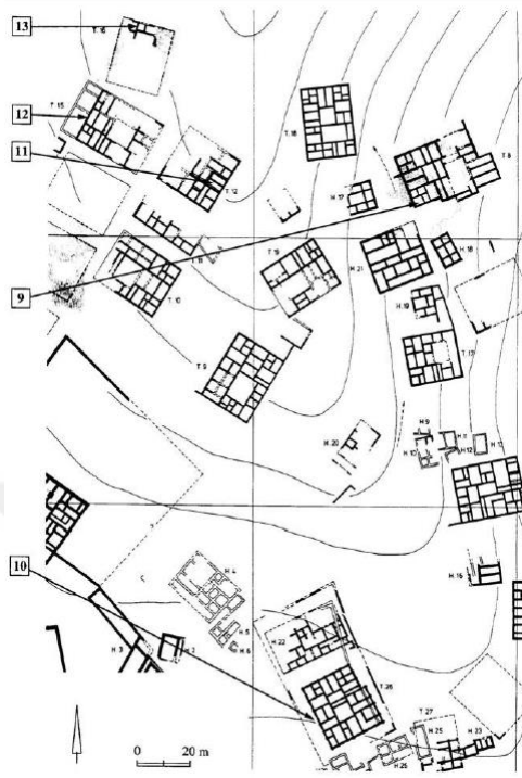
Şekil 2. 17: Hattuşa Kenti Yukarı Şehir Tapınak Alanı Detay; 8, 12, 15, 16 ve Olası 26 Numaralı Tapınaklarda Bulunan Arşiv ve Kütüphaneler
