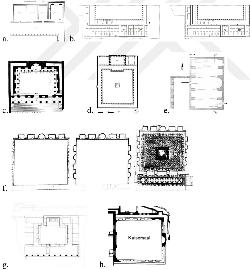
Şekil 4.1: Tez Çalışmasında İncelenen Mimari Kalıntıları Mevcut Hellenistik Dönem ve Roma Dönemine Ait Küçük Asya Kütüphaneleri'nin Plan Karşılaştırılması, a. Pergamon Kraliyet Kütüphanesi, b. İskenderiye Serapis Kütüphanesi, c. Ephesos Celsus Kütüphanesi, d. Side M Binası Kütüphanesi e. Kremna Kütüphanesi, f. Sagalassos Neon Kütüphanesi, g. Nysa Kütüphanesi, h. Pergamon Asklepion Kütüphanesi
