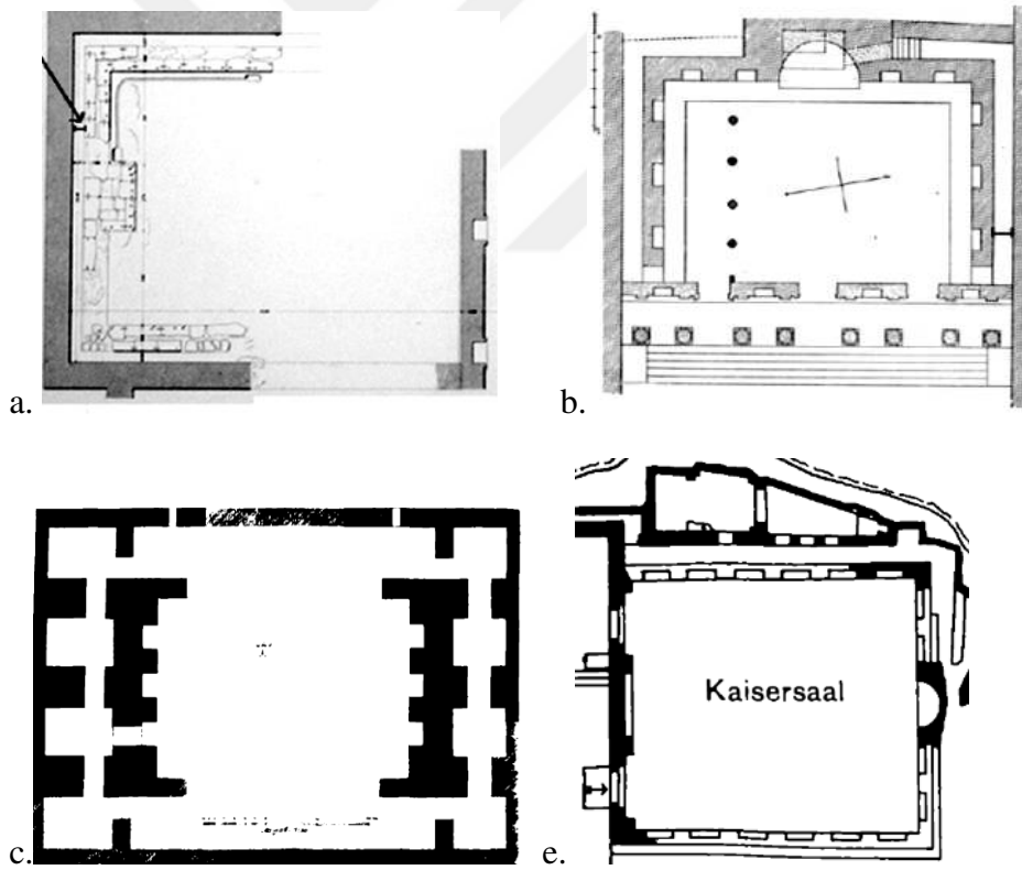
Şekil 4.3: Duvar Boşluğu Olan Kütüphaneler; a. Pergamon Kütüphanesi Podium ve Duvar Arasındaki Havalandırma Boşluğu, b. Ephesos Celsus Kütüphanesi Podium ve Duvar Arasında ki Boşluğun Görünümü, c. Nysa Kütüphanesi Havalandırma Boşluğu, e. Pergamon Asklepion Kütüphanesi Salon etrafını Çevreleyen Çift Duvar
