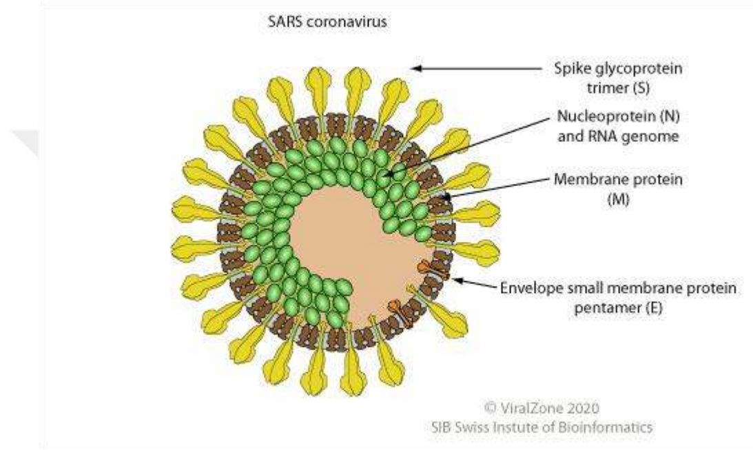
Şekil 7. Koronavirüs'ün yapısı
