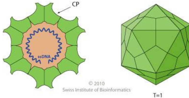
Şekil 8. Bokavirüsün yapısı-1
