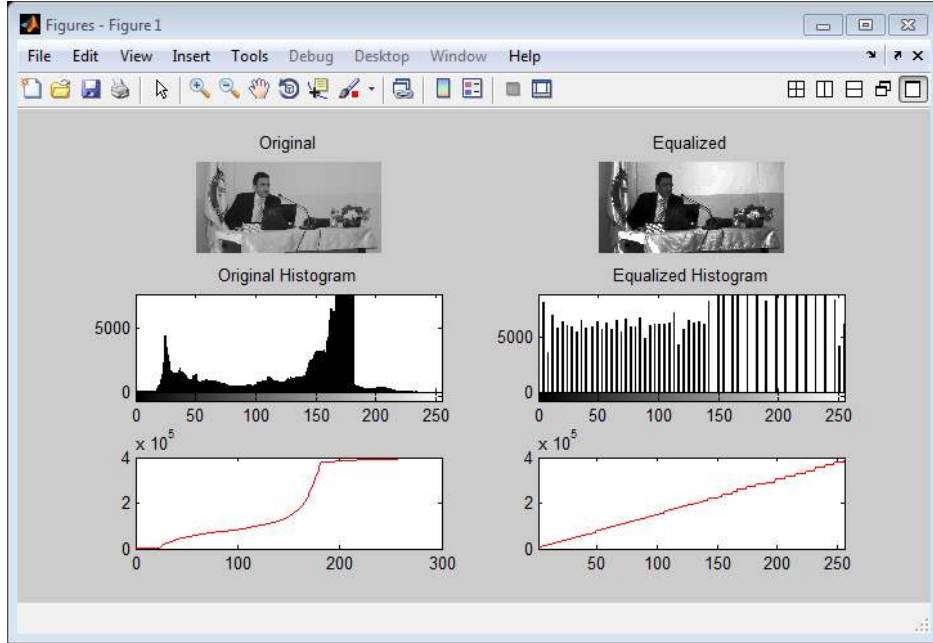
Şekil 3.7. Histogram Eşitleme
