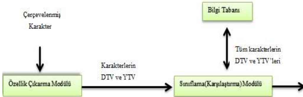
Şekil 3.22. Tekleştirme Modeli İle Tanıma Sisteminin Genel Yapısı
