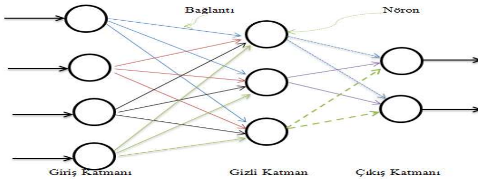
Şekil 5.16. ÇKA modeli
