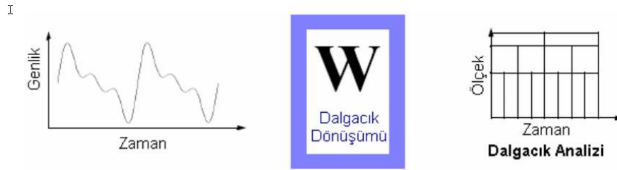
Şekil 5.11. Dalgacık Dönüşümü [78]
