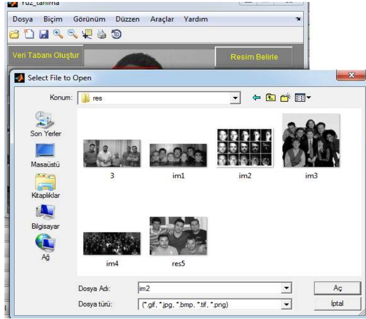
Şekil 6.12. Resim Belirleme
