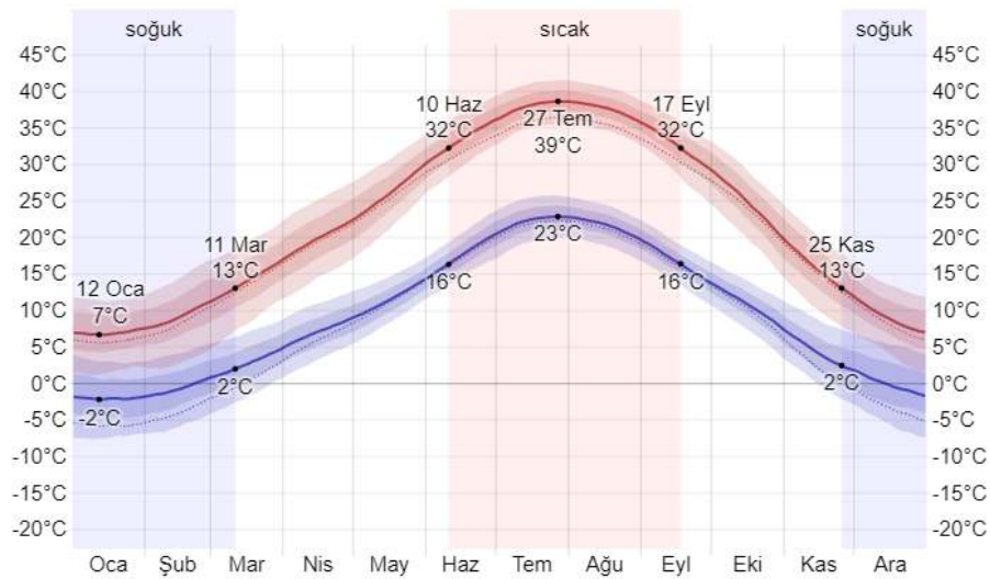
Şekil 3. 35 Günlük ortalama yüksek (kırmızı çizgi) ve düşük (mavi çizgi) sıcaklık (Weather Spark, 2022)
