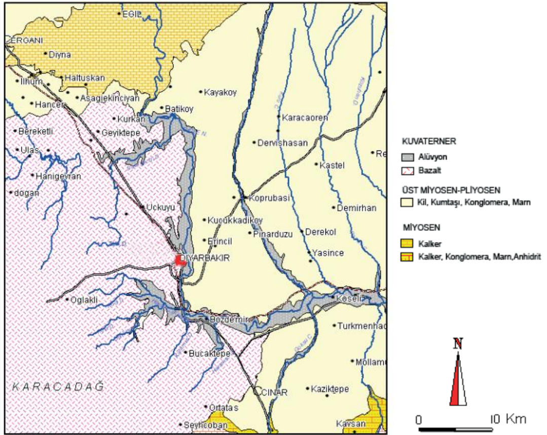
Şekil 3. 27 Diyarbakir kenti ve yakın çevresinin jeoloji haritası (Karadoğan, 2019)
