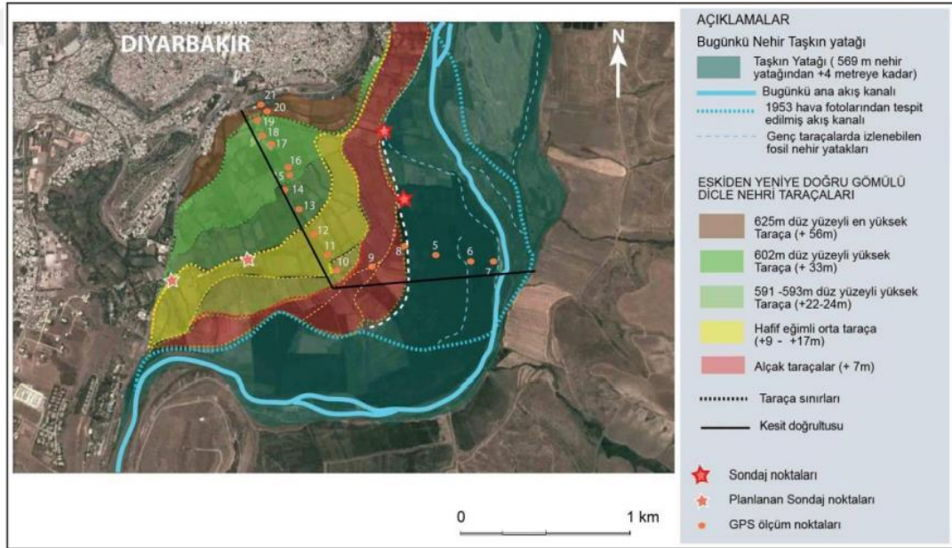
Şekil 3. 25 Hevsel Bahçeleri taraçalarının jeomorfoloji haritası (Karadoğan ve Kuzucuoğlu, 2018)
