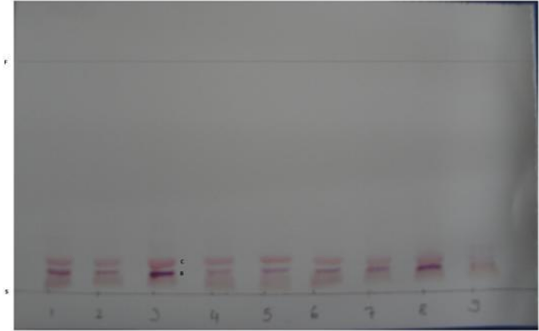
Resim 36. İTK plağında Hibiscus sabdariffa örnekleri (Tablo 6.'da belirtilen sıraya göre tatbik yapılmıştır.) Solvan Sistemi: Etil asetat: Glasiyel asetik asit: Formik asit: Su (100:11:11:26 h/h/h/h )
