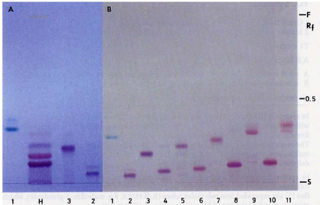
Resim 37. Ekstrelerin Plant Drug Analysis'e göre İTK deneyi sonuçları. Solvan Sistemi: Etil asetat: Glasiyel asetik asit: Formik asit: Su (100:11:11:26) Analiz numunesi: H Hibiscus flos (Metanollü ekstre, 25 µl) Referans maddeler: 1.metilen blue, 2.delfinidin-3,5- diglikozit, 3.delfinidin-3-glikozit, 4.petunid-3,5- diglikozit, 5.petunid-3-glikozit, 6.siyanidin-3,5- diglikozit, 7.siyanidin-3-glikozit, 8.malvinidin-3,5-diglikozit, 9.malvinidin-3-diglikozit, 10.paeonidin-3,5-diglikozit, 11.paeonidin-3-glikozit 121 .
