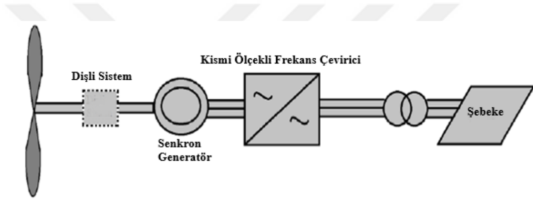
Şekil.2.5. Senkron generatörlerin şebekeye bağlantı şeması [28].
