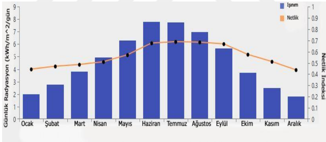
Şekil 4.10. Aylık ortalama solar radyasyon (kWh/m²/gün) profili (HOMER Energy, 2021)
