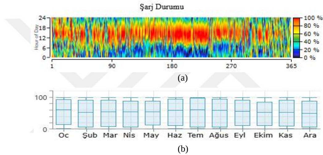
Şekil 5.14. PV, jeneratör, PHD sisteminin depolama performansı
