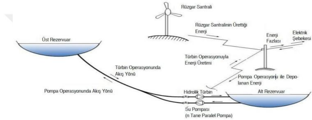
Şekil 4.3. Rüzgâr ve pompaj hidroelektrik depolamalı hibrit sistem (Ünver vd., 2015)
