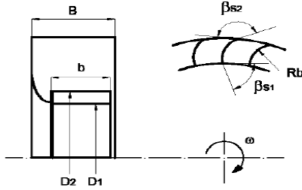
Şekil 2.4. Rotor parametreleri [10]
