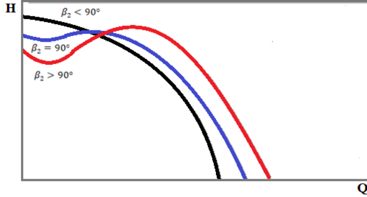
Şekil 3.4. Gerçek basma yüksekliği-debi eğrileri [14]
