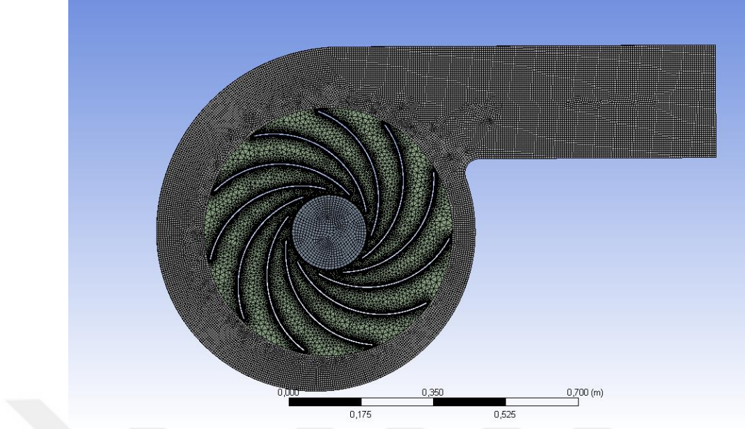
Şekil 5.1. Radyal fanın mesh yapısının gösterimi
