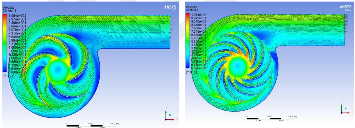
Şekil 5.12. Model 15 ve Model 111 akış hız modelleri
