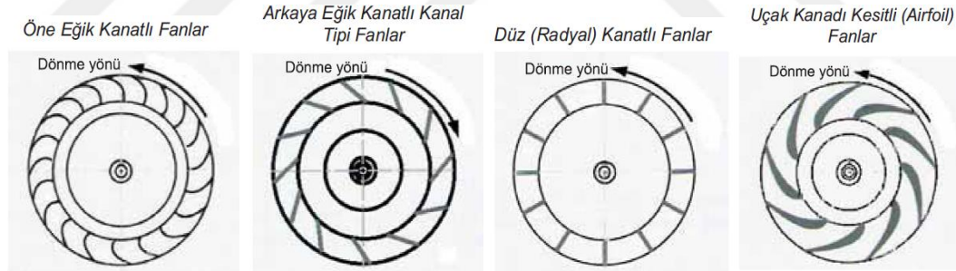
Şekil 2.5. Radyal fan çeşitleri [1]
