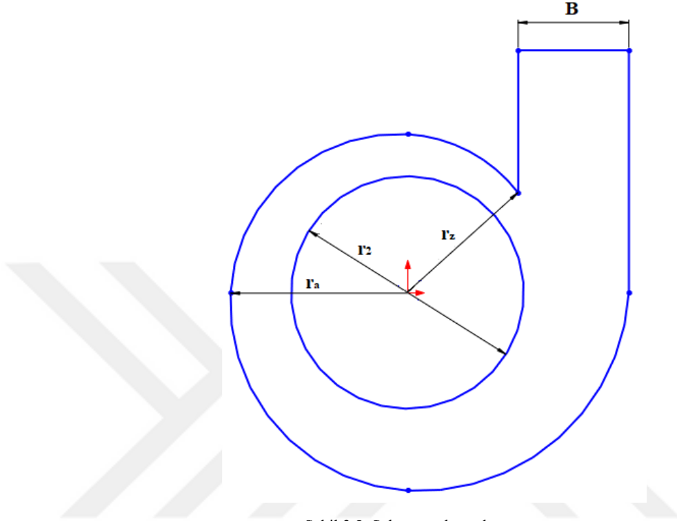
Şekil 3.8. Salyangoz boyutları
