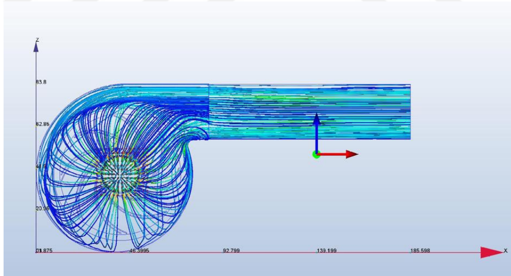
Şekil 5.4. Radyal fanın oluşturduğu akışın hızvektörlerinin çizgisel gösterimi
