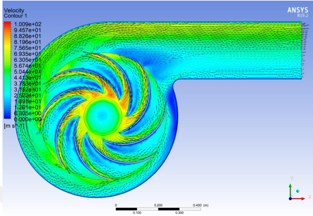
Şekil 5.3. Radyal fanın oluşturduğu akışın hız modellemesi
