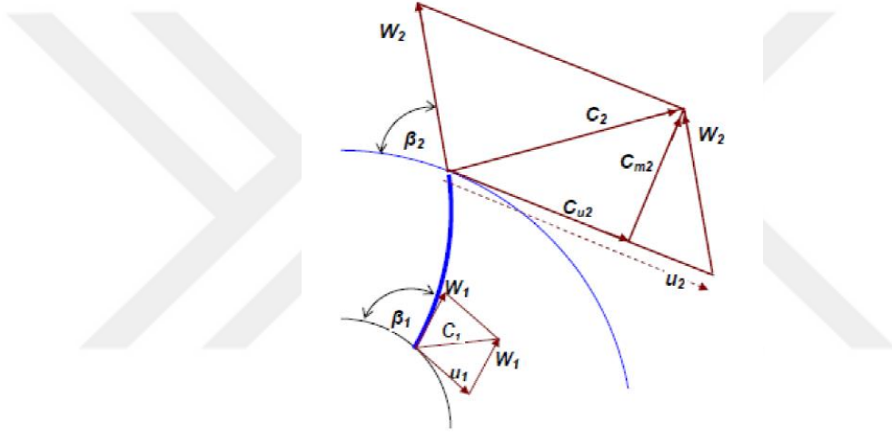
Şekil 3.1. Kanat giriş ve çıkışındaki hız üçgenleri [14]
