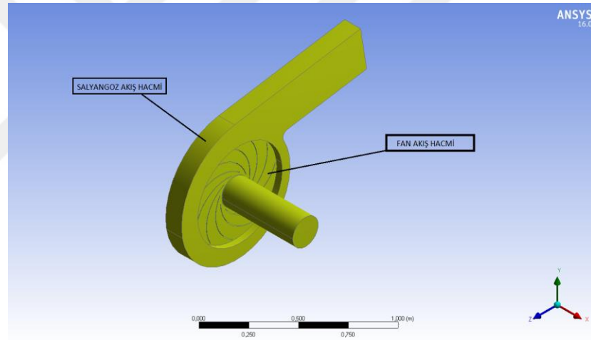
Şekil 5.2. Radyal fan içersindeki akış hacmi
