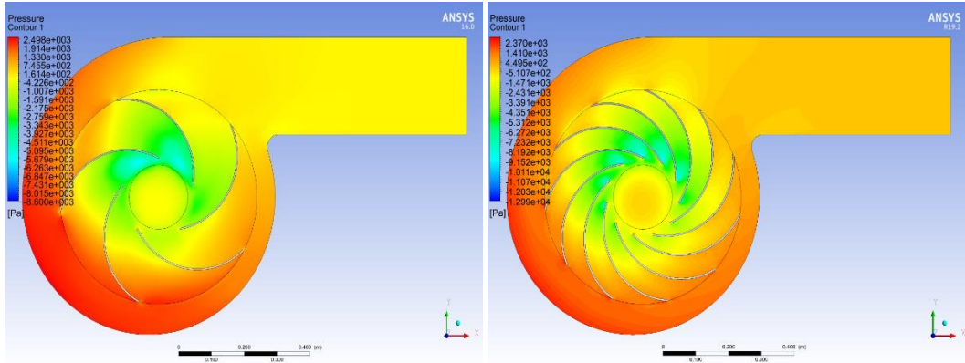
Şekil 5.11. Model 05 ve Model 011 akış basınç modelleri
