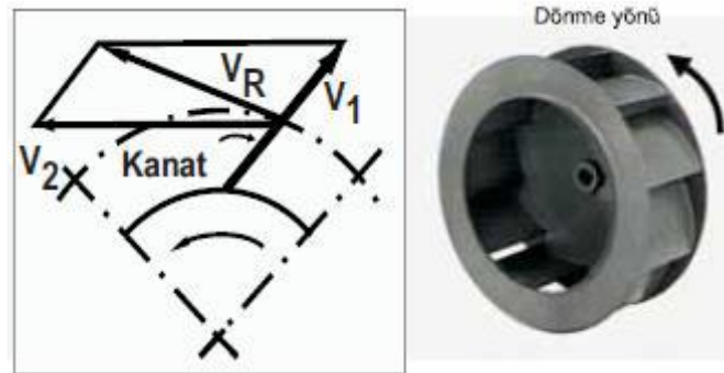
Şekil 2.13. Airfoil kanatlı radyal fan [2]
