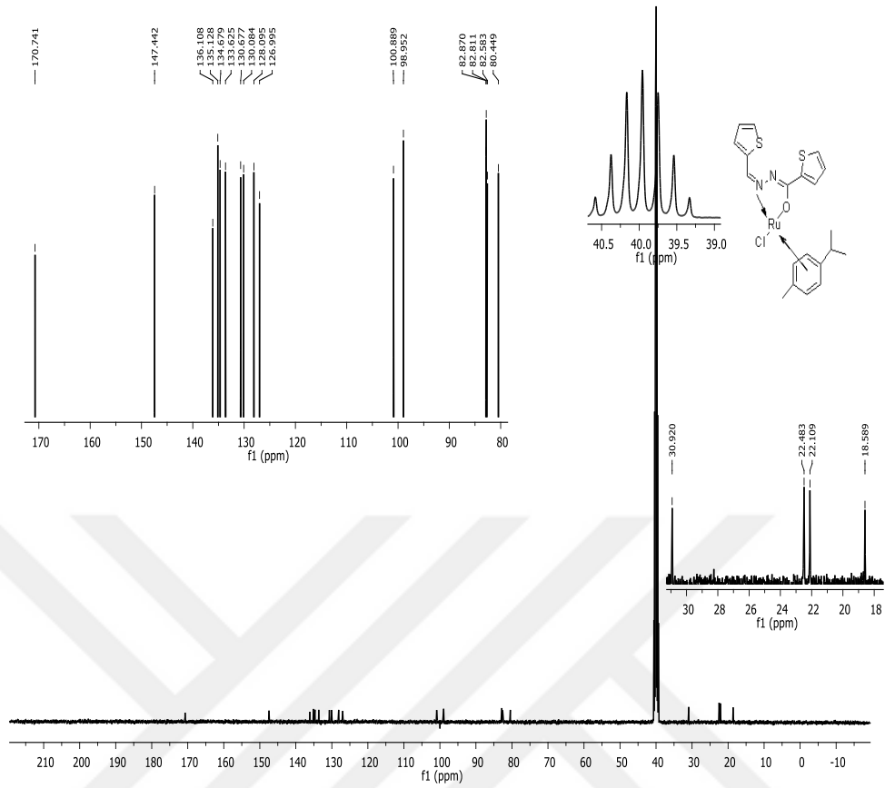
Şekil 16. N'-(tiyofen-2-ilmetilen)tiyofen-2-karbohidrazitin Rutenyum Kompleksinin (4a), ^{13}\text{C} -NMR spektrumu
