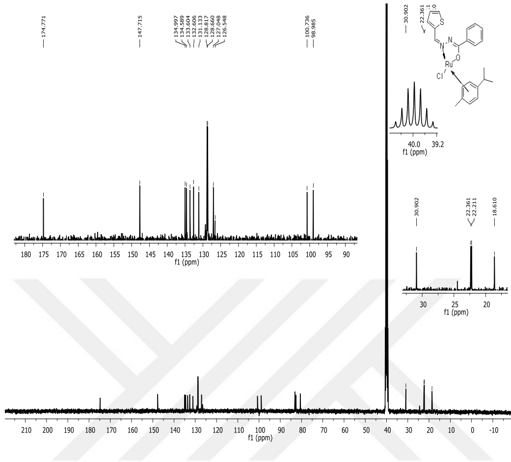
Şekil 21. N'-(tiyofen-2-ilmetilen) Benzohidrazitin Rutenyum Kompleksi (4b)'nin, ^{13}\text{C} -NMR spektrumu
