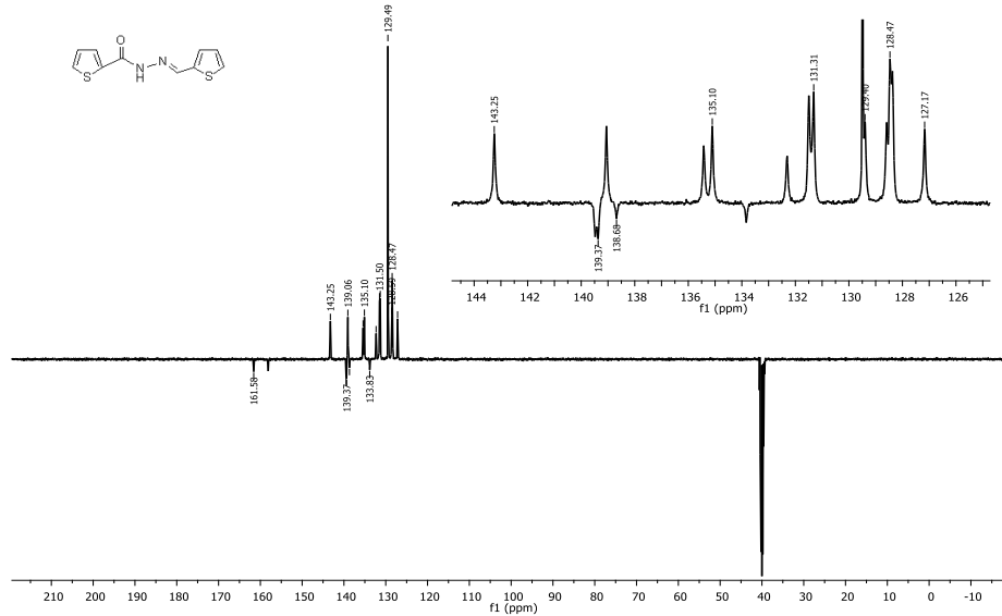
Şekil 8. N'-(tiyofen-2-ilmetilen)tiyofen-2-karbohidrazit (3a) molekülünün ^{13}\text{C} APT-NMR spektrumu
