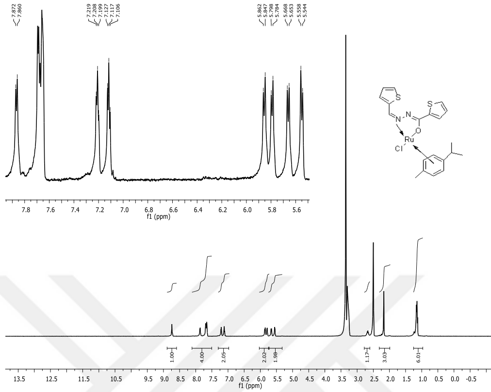
Şekil 15. N'-(tiyofen-2-ilmetilen)tiyofen-2-karbohidrazitin Rutenyum Kompleksinin (4a), ^1\text{H} -NMR spektrumu
