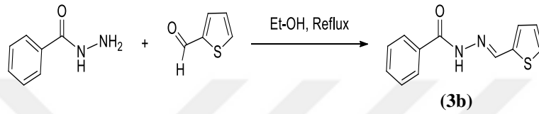
Şekil 9. N'-(tiyofen-2-ilmetilen) benzohidrazit ligandının (3b) sentez şeması
