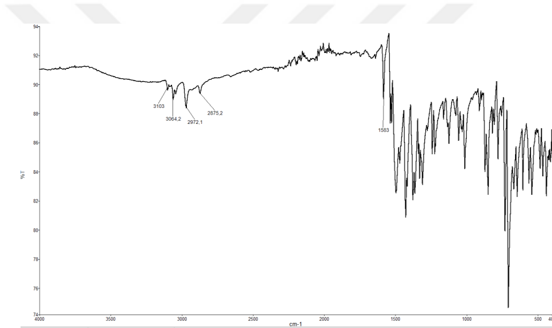
Şekil 14. N'-(tiyofen-2-ilmetilen)tiyofen-2-karbohidrazitin Rutenyum Kompleksinin (4a), FT-IR spektrumu
