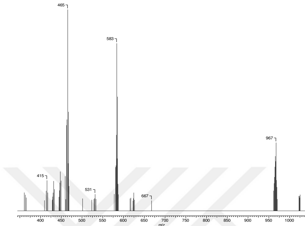
Şekil 22. N'-( tiyofen-2-iletillen) Benzohidrazitin Rutenyum Kompleksi (4b)'nin, ESI-MS spektrumu
