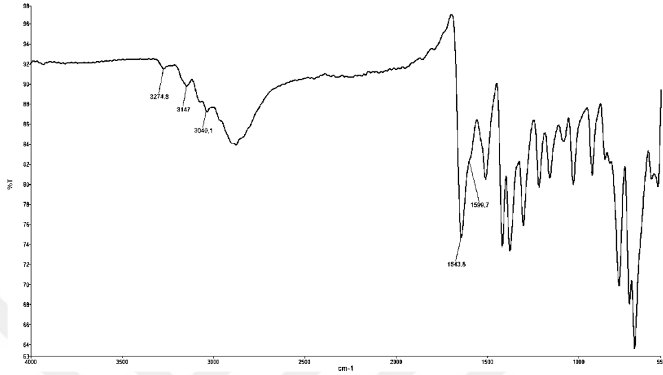
Şekil 6. N'-(tiyofen-2-ilmetilen)tiyofen-2-karbohidrazit (3a) molekülünün FT-IR spektrumu.
