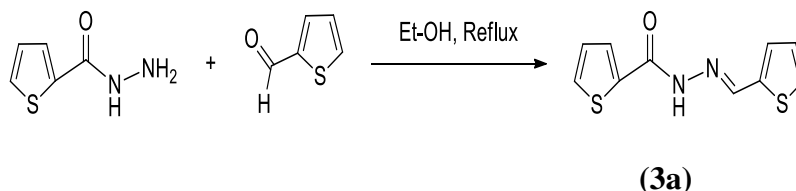
Şekil 5. N'-(tiyofen-2-ilmetlen)tiyofen-2-karbohidrazit (3a) ligandının sentez şeması
