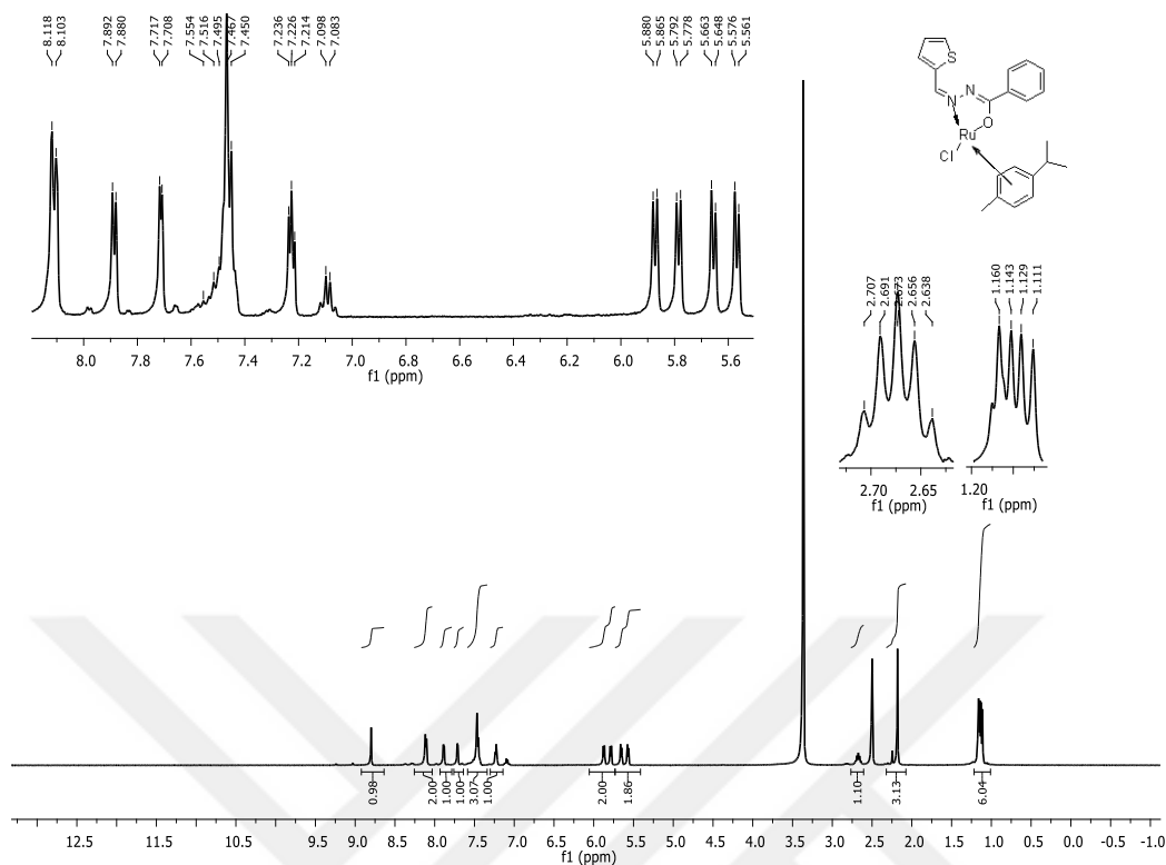
Şekil 20. N'-( tiyofen-2-ilymetilen) Benzohidrazitin Rutenyum Kompleksi (4b)'nin, ^1\text{H} -NMR spektrumu
