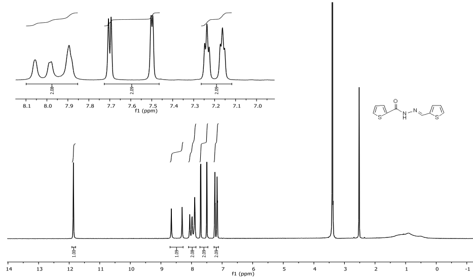
Şekil 7. N'-(tiyofen-2-ilmetilen)tiyofen-2-karbohidrazit (3a) molekülünün ^1\text{H} -NMR spektrumu
