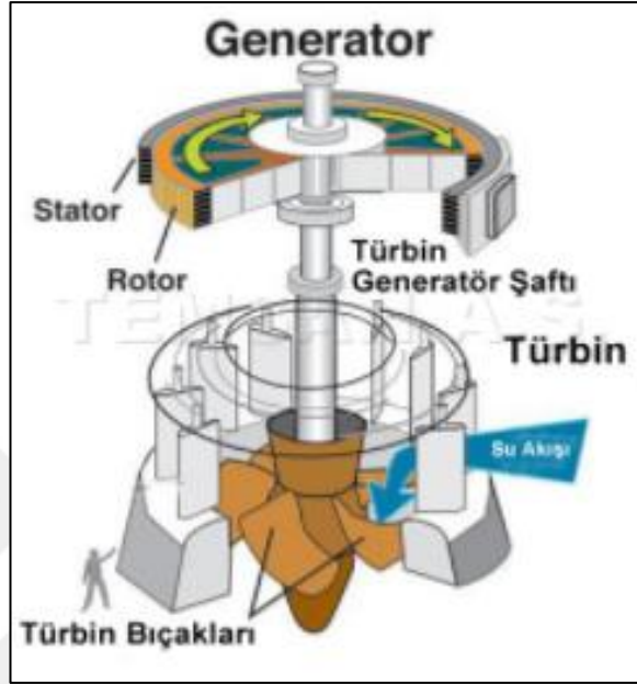
Şekil 2.8. Kaplan türbin prensip şeması (TEMSAN, 2018).
