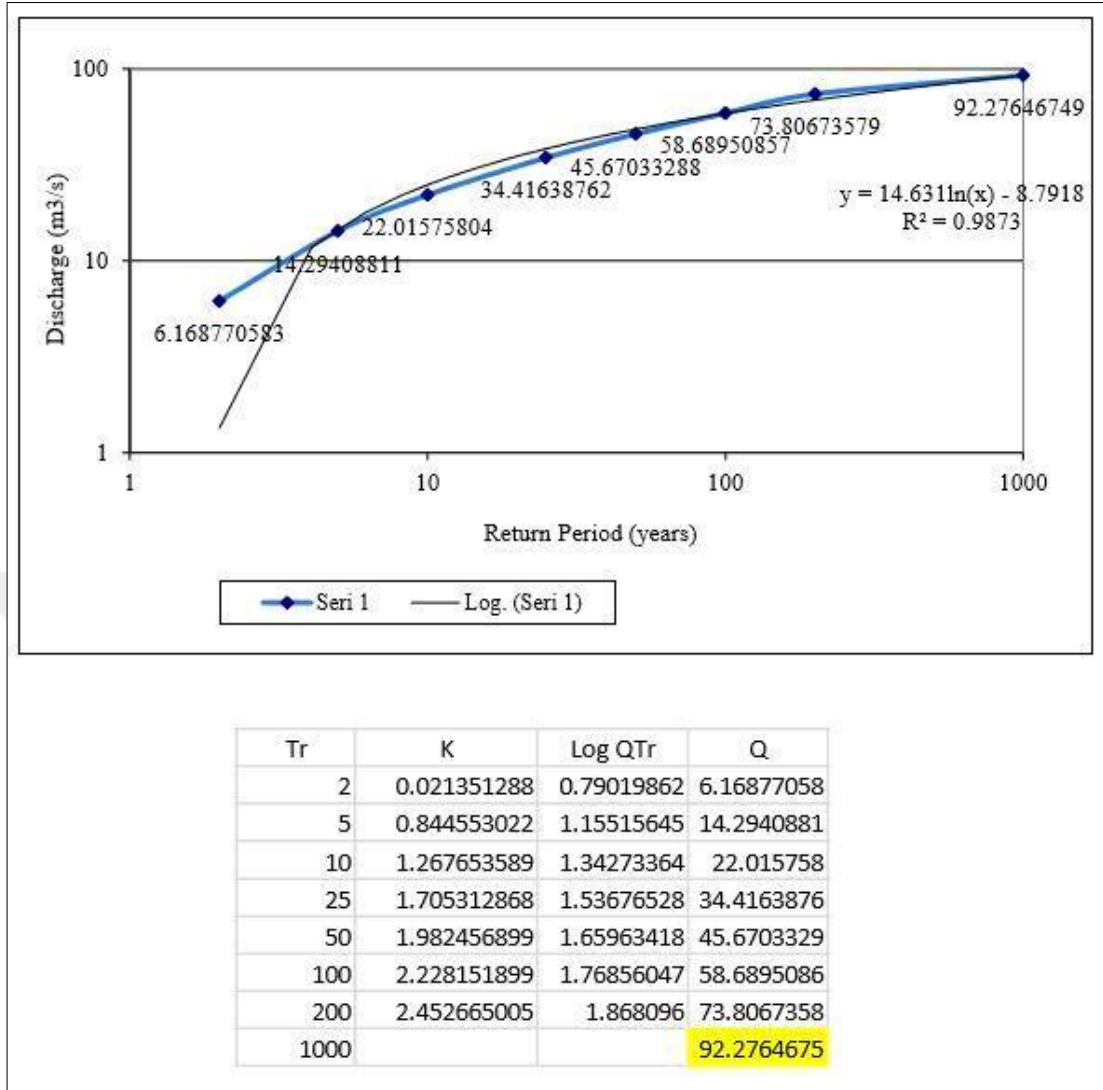
Şekil 6.10. Log Pearson Type 3 istatistiksel metoduna göre, DSI-12185 AGİ’de, 2, 5, 10, 25, 50, 100, 1000 yıllık taşkın tekrerr periyotlarında oluşması beklenen debiler.
