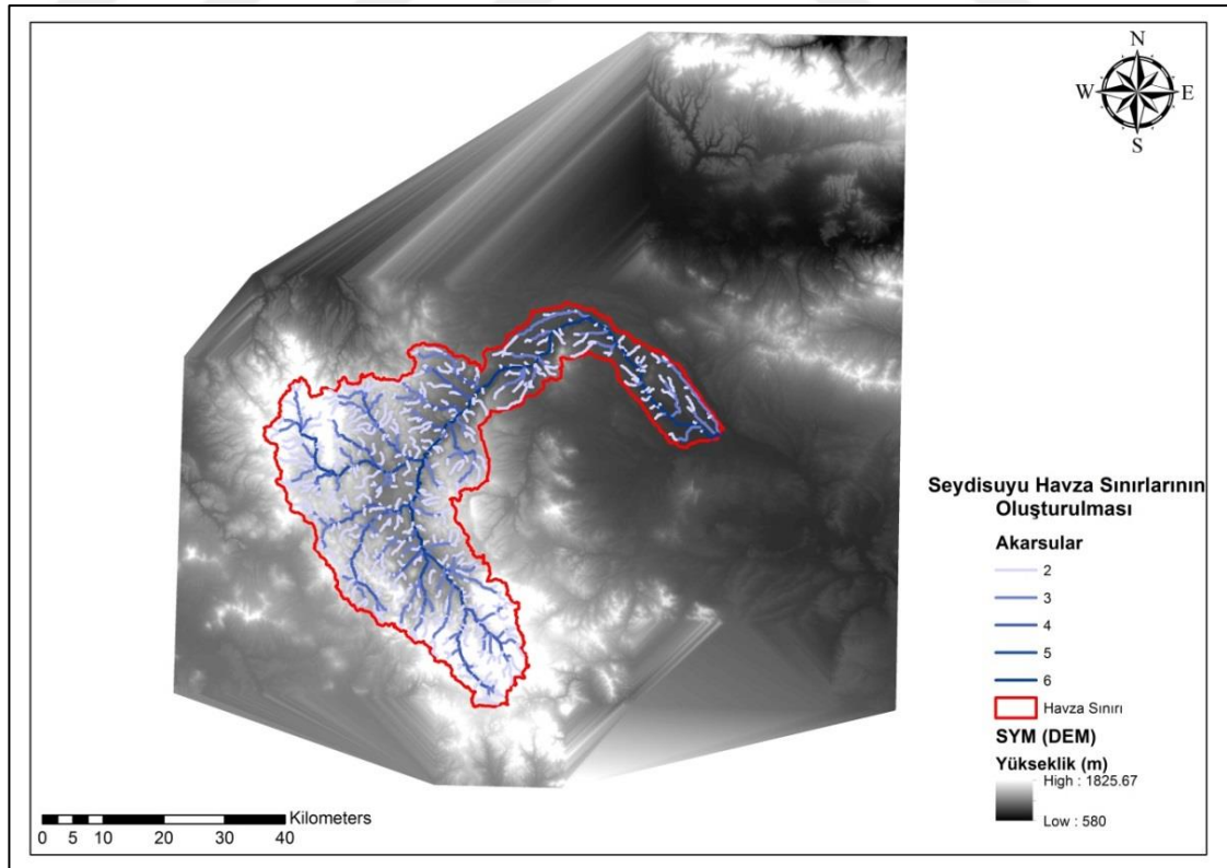
Şekil 5.20. Seydisuyu havzası.
