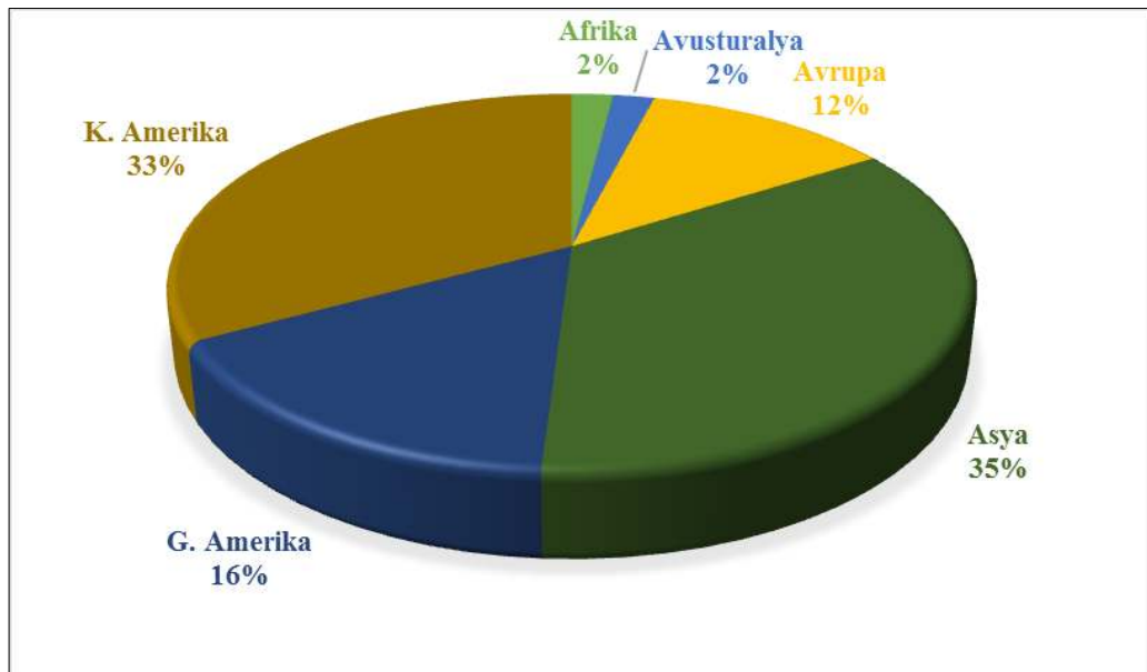
Şekil 2.5. Dünyada üretilen hidroelektrik enerjinin kıtalara göre dağılımı (Şekkeli ve Keçecioğlu, 2011).
