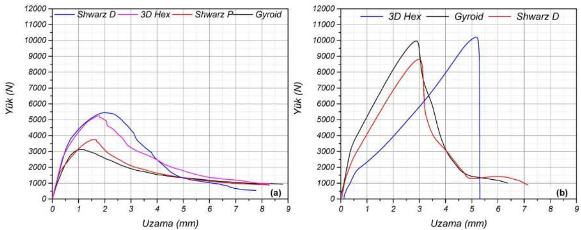
Şekil 3.29. % 25 doluluk oranına sahip ÜPMY vida çekme modellerine ait (a) PLA (b) HAp+PLA+TPE yük-uzama eğim grafiği
