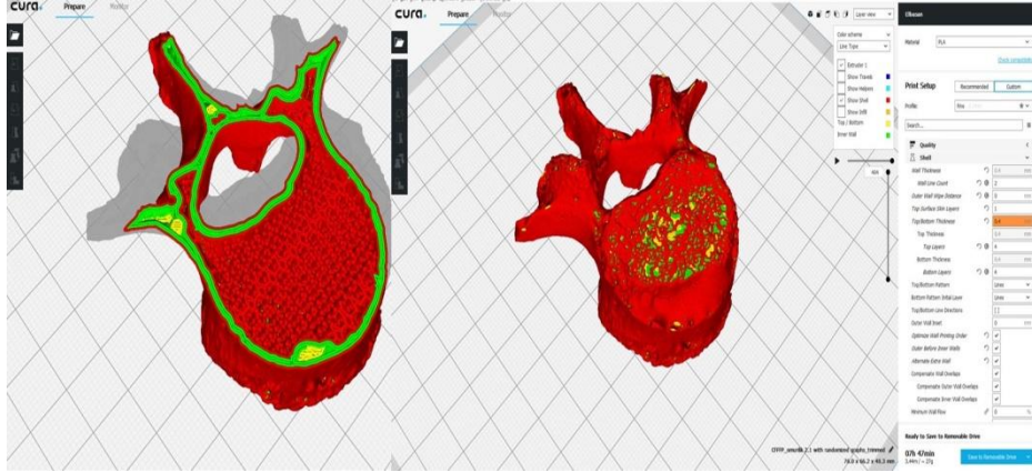
Şekil 2.9. 3B Omur modelinin Cura programında baskı parametrelerinin düzenlenmesi
