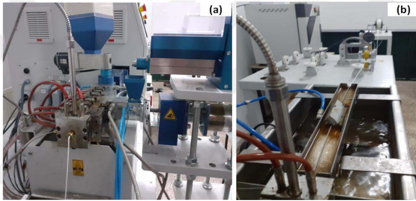
Şekil 2.4. Kompozit ve saf filamentlerin üretimi (a) çift taraflı ekstruder, (b) tek taraflı ekstruder
