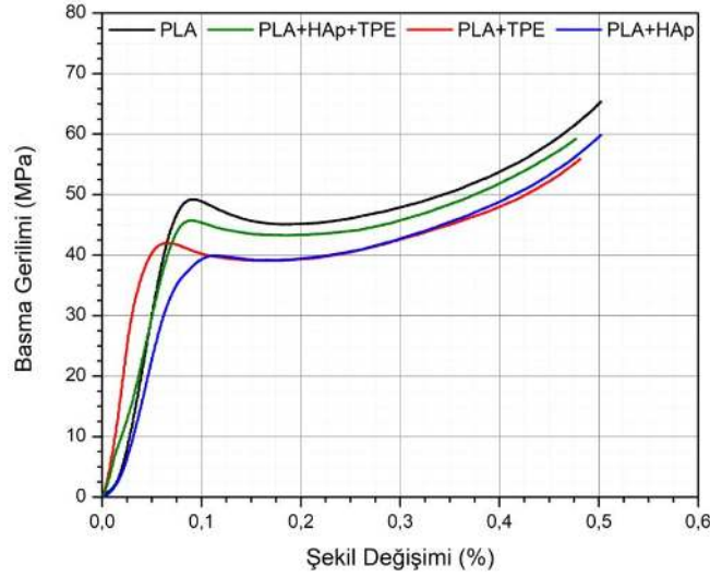
Şekil 3.15. PLA ve kompozit 3B basma numunelerine ait basma gerilim-şekil değişim grafiği
