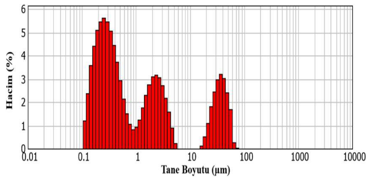
Şekil 3.4. Kalsinasyon yöntemi ile elde edilen hidroksiapatit tane boyut-hacim dağılımı
