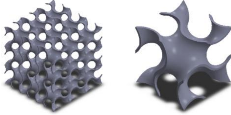
Şekil 1.5. Gyroid kafes yapısı [43]
