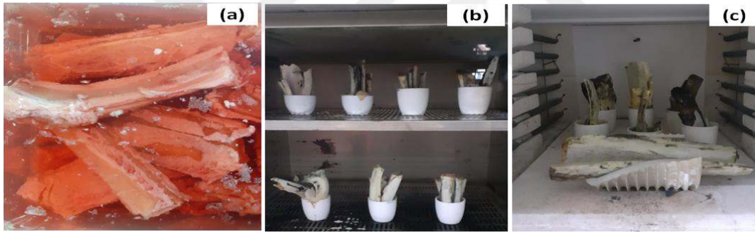
Şekil 2.2. Kalsinasyon yöntemi ile HA üretimi (a) solüsyonu (b) kurutma (c) kalsinasyon
